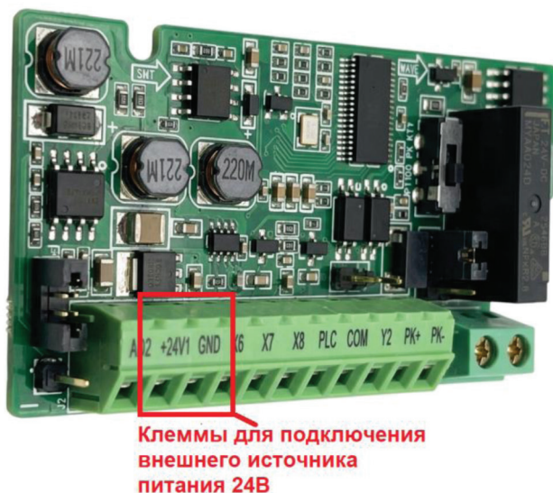
Рисунок 7-2. Подключение внешнего источника питания к PBC00027 (последняя ревизия)
