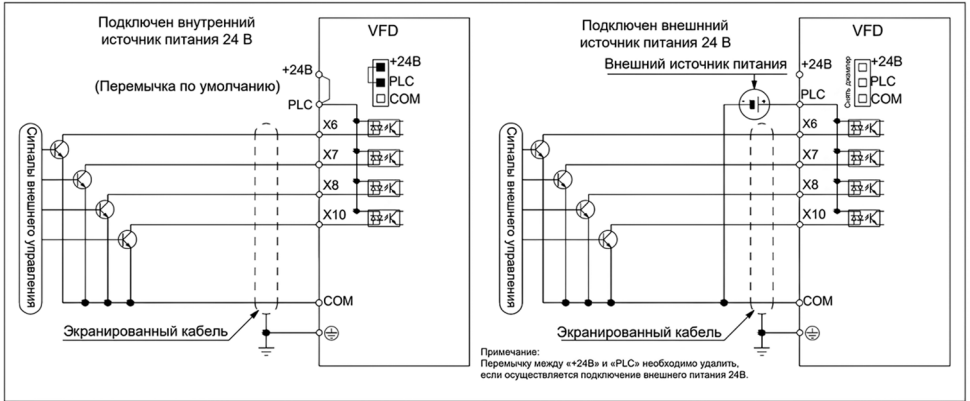
Рисунок 2.1-1. Подключение NPN
