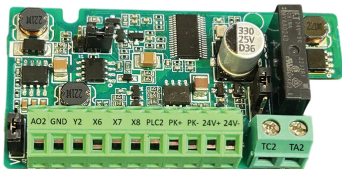
Рисунок 1-2. Внешний вид платы PBC00027 (первая ревизия)
