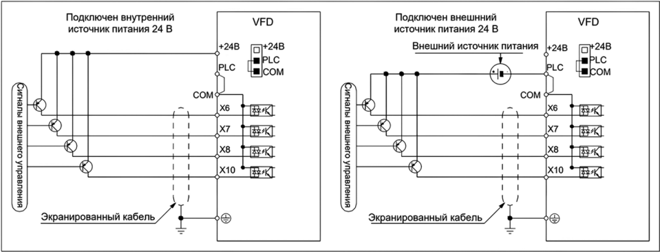
Рисунок 2.1-2. Подключение PNP
