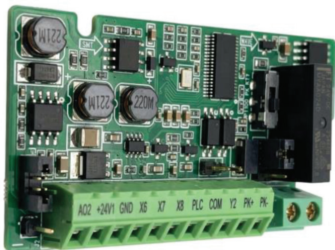
Рисунок 1-3. Внешний вид платы PBC00027 (последняя ревизия)
