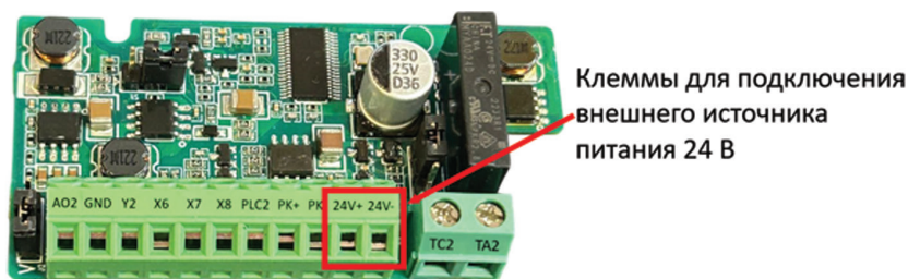
Рисунок 7-1. Подключение внешнего источника питания к PBC00027 (первая ревизия)
