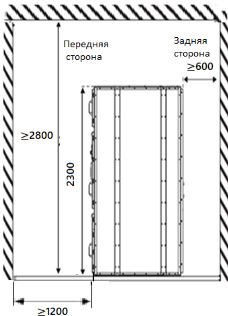
Рис. 6.3 – Установка УПП в помещении
