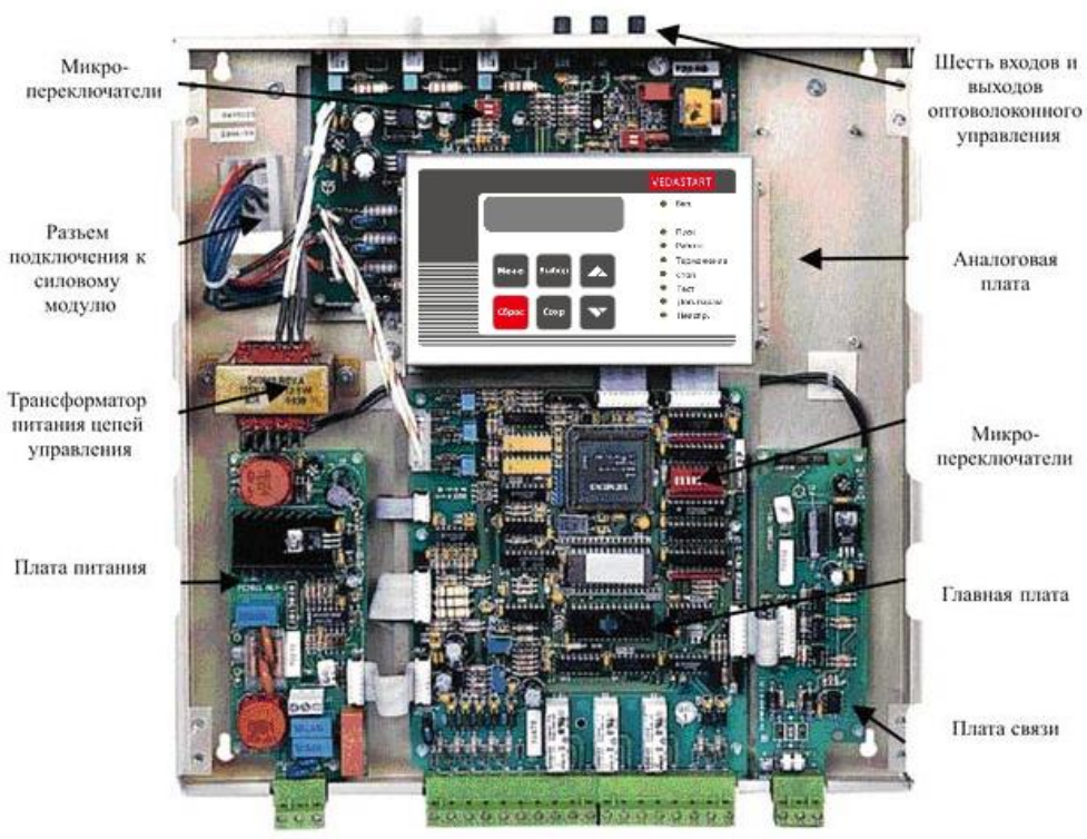
Рис. 7.4 – Модуль управления
