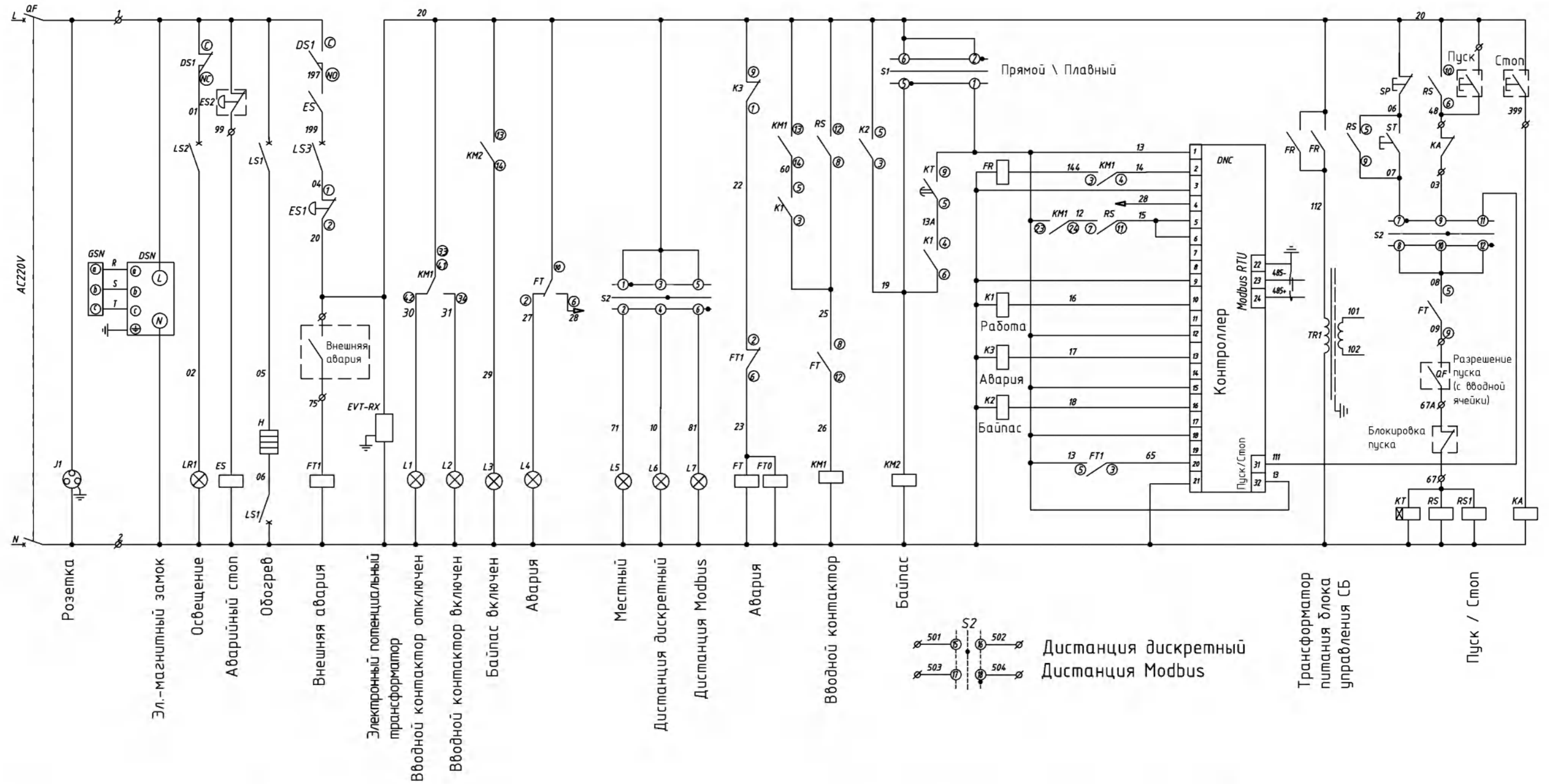
Схема вторичных цепей
