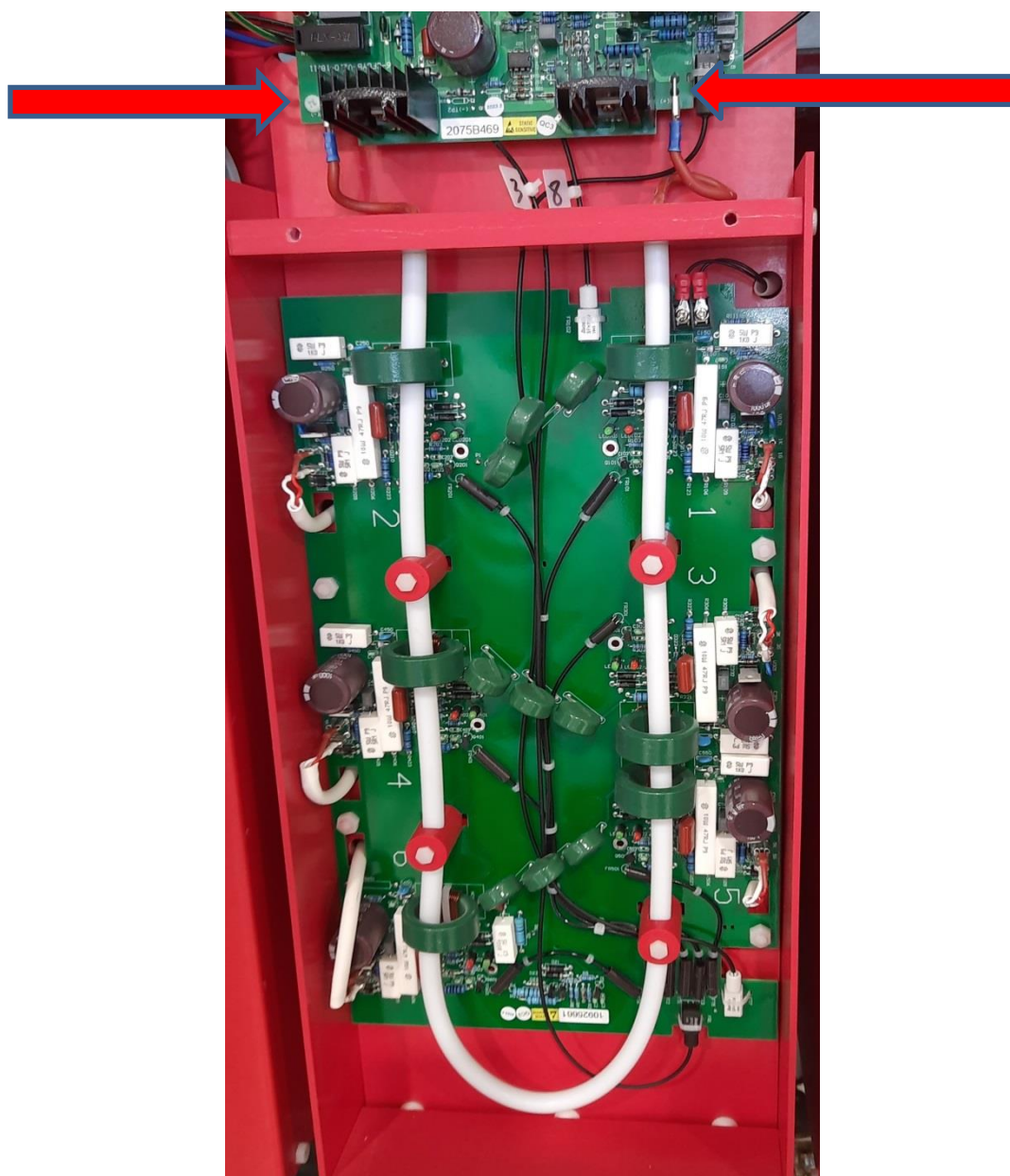
Рис. Б.4 – Плата управления тиристорами и блок питания платы управления тиристорами в силовом тиристорном блоке с указанием места измерения вторичного напряжения
