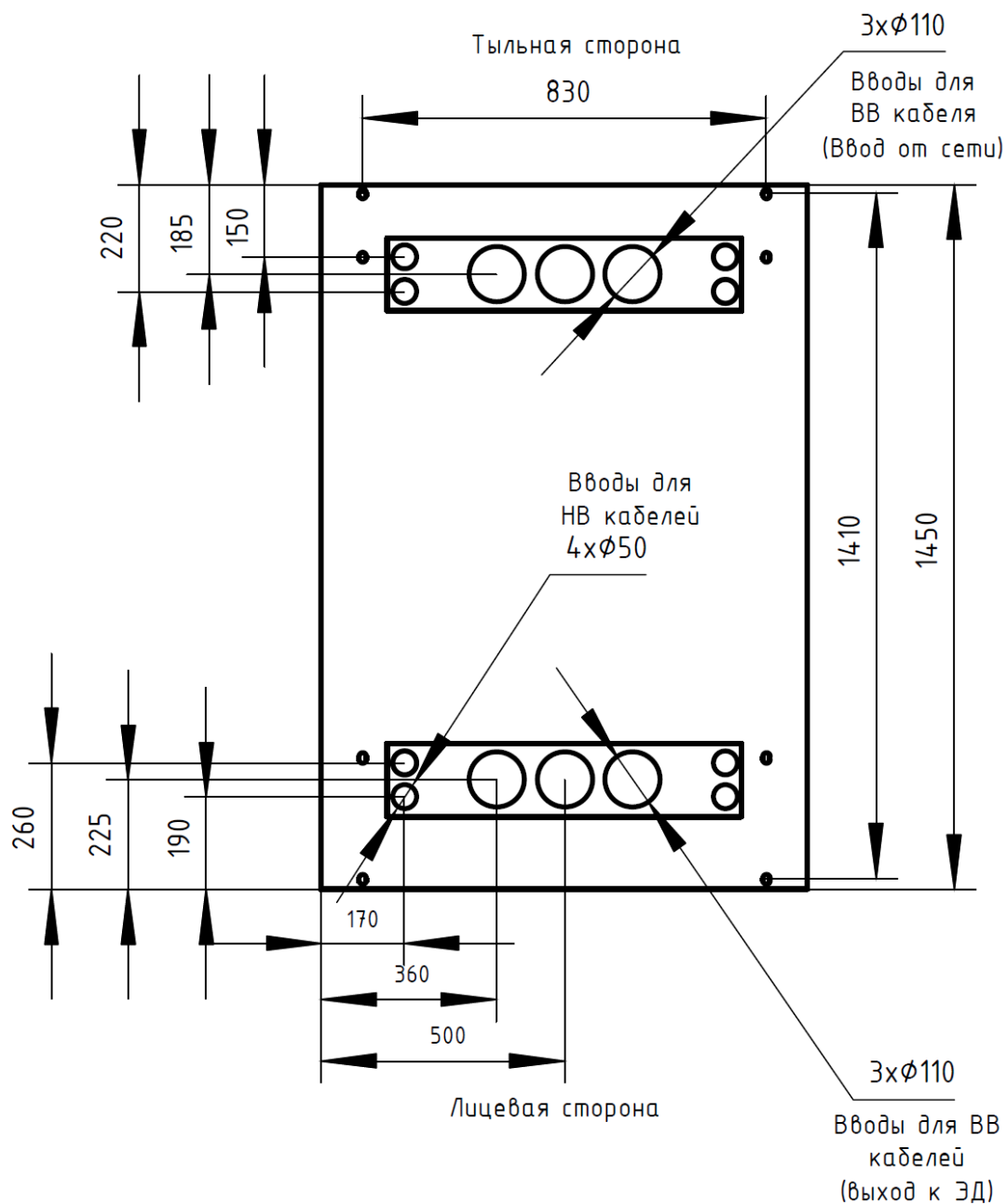
Рис. 6.2 – Рама основания УПП (вид сверху, на примере УПП с номинальным током до 300 А включительно)
