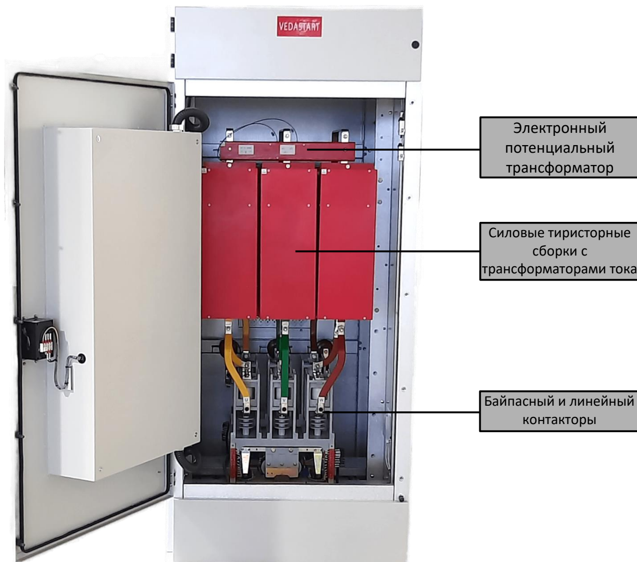
Рис. 7.1 - Внешний вид высоковольтного отсека УПП Vedastart
