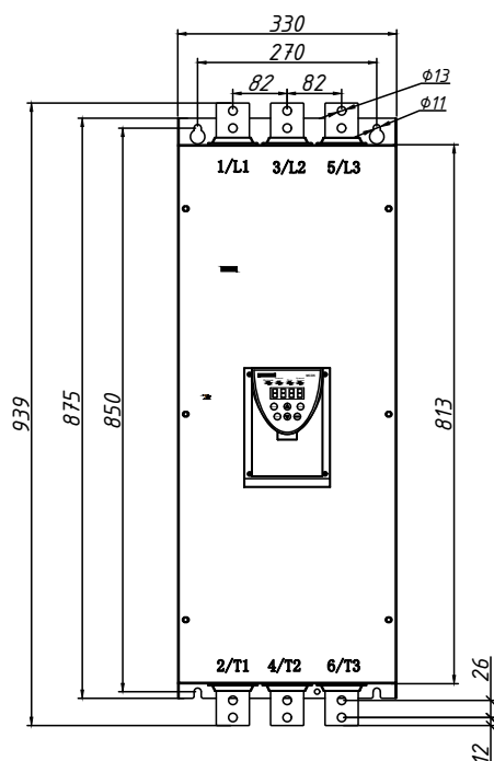
Типоразмер F6 (560-820A)
