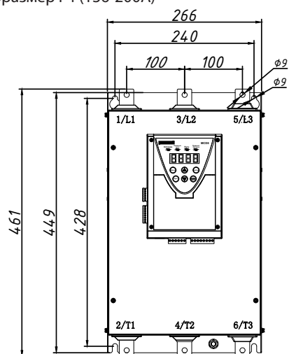
Типоразмер F4 (136-200A)
