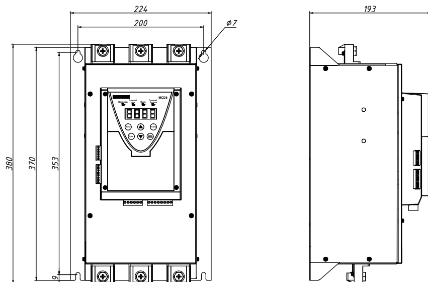
Типоразмер F3 (93-140A)
