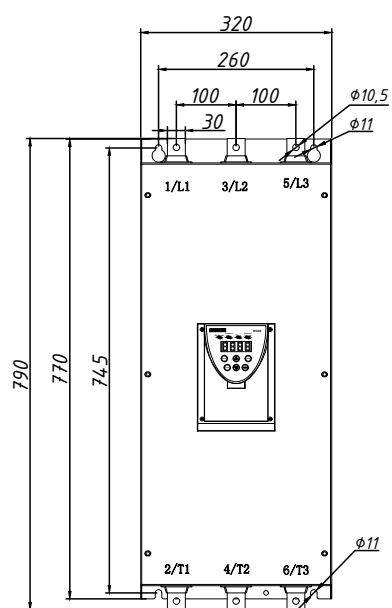
Типоразмер F5 (207-480A)
