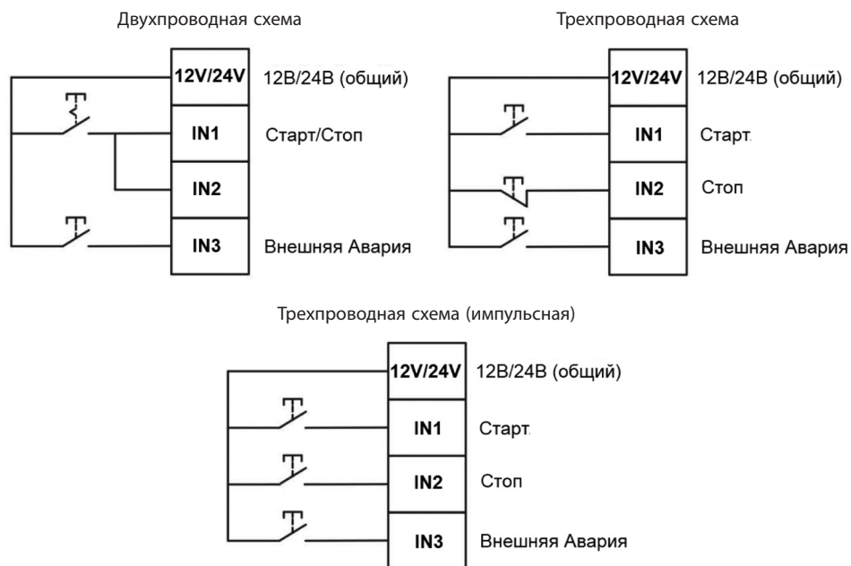
Рисунок 3. Режимы управления
