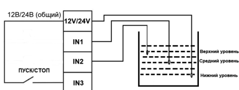
Рисунок 5. Параметр F36, функциональное описание
