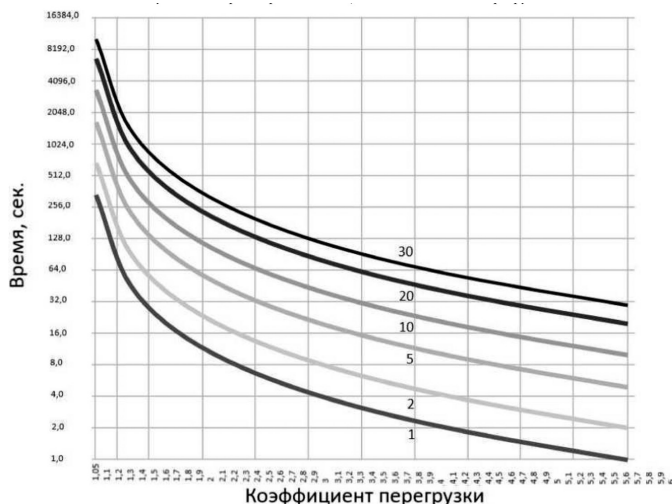
Рисунок 10. Характеристика защиты двигателя от перегрузки
