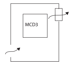
Шкаф общего назначения Вентилятор на выходе воздуха
