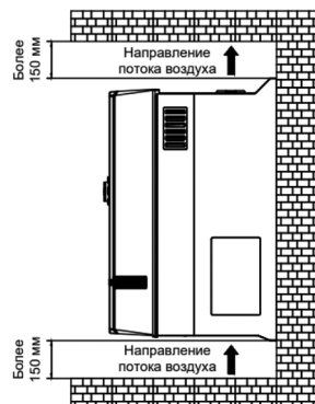
Рис. 3.5-1. Положение преобразователя частоты и требуемое пространство
