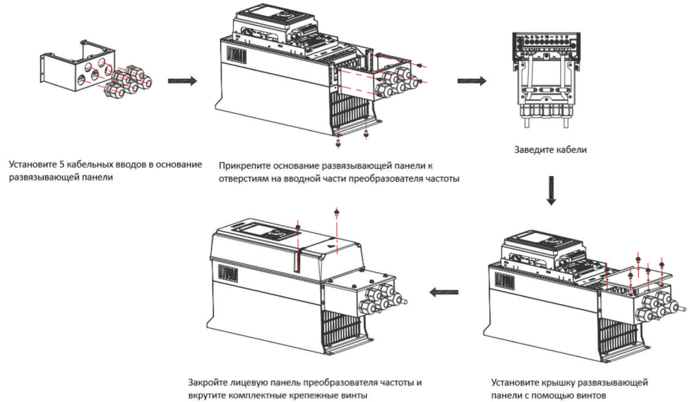
Рис. 3.6-6. Последовательность установки развязывающей панели
