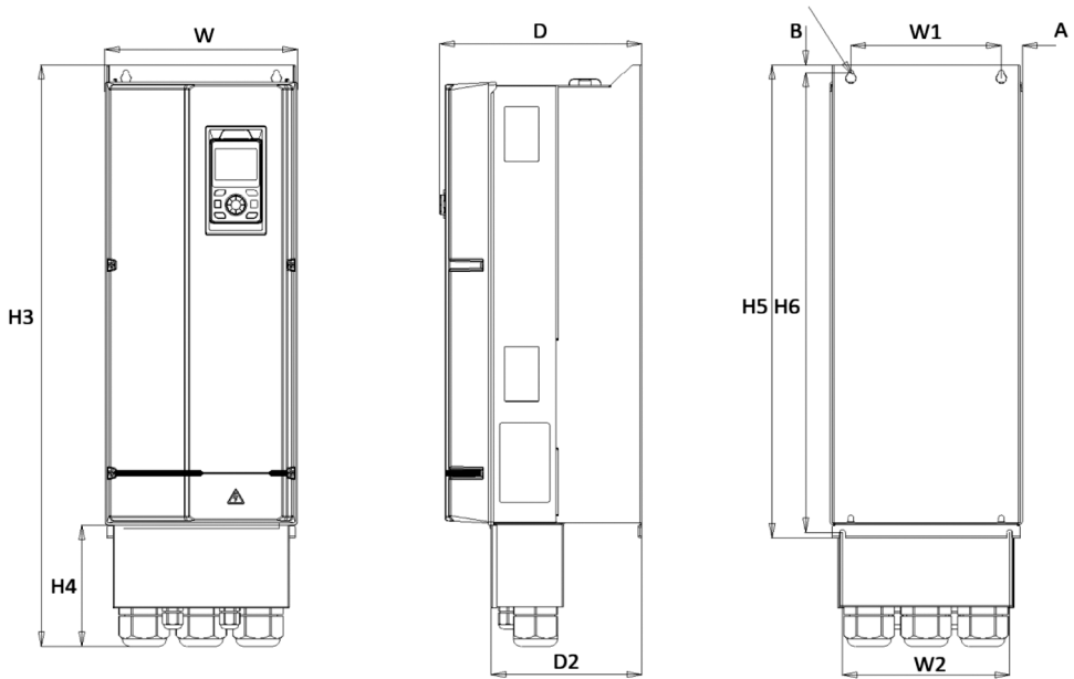
Рис. 3.6-5. Чертеж преобразователя частоты IP54 типоразмеров МН4
