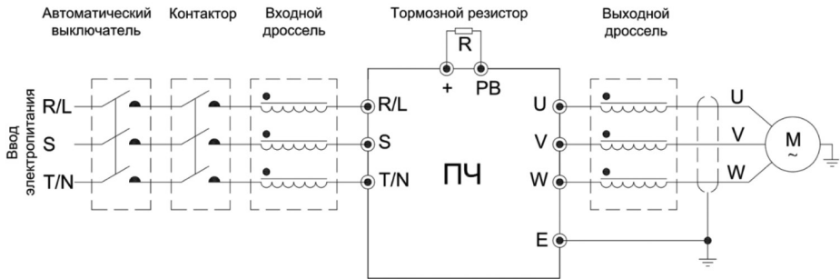
Рис. 4.1-1. Схема подключения преобразователя частоты
