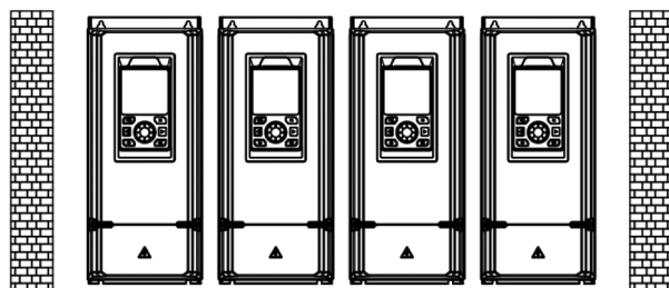
Рис. 3.5-1. Положение преобразователя частоты и требуемое пространство
