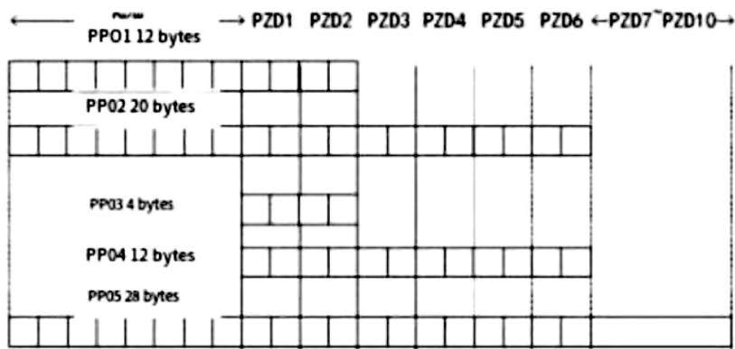
Рис. 8. Описание структуры данных PPO
