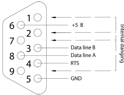
Рис. 3. Распиновка разъема DB9
