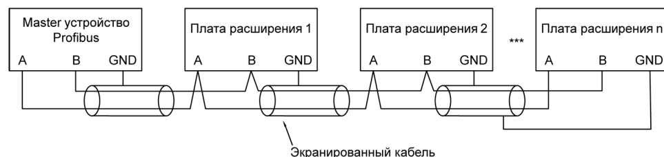
Рис. 7.1. Подключение к шине Profibus
