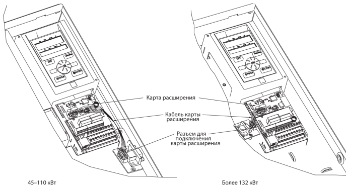
Рис. 2.2. Монтаж платы на преобразователях частоты высокой мощности
