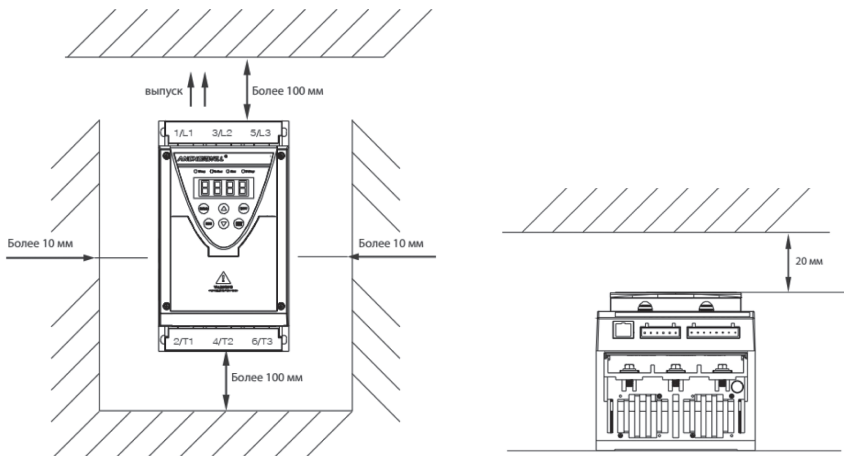
Рис. 3-1а. Расстояние между местами установки (мм)
