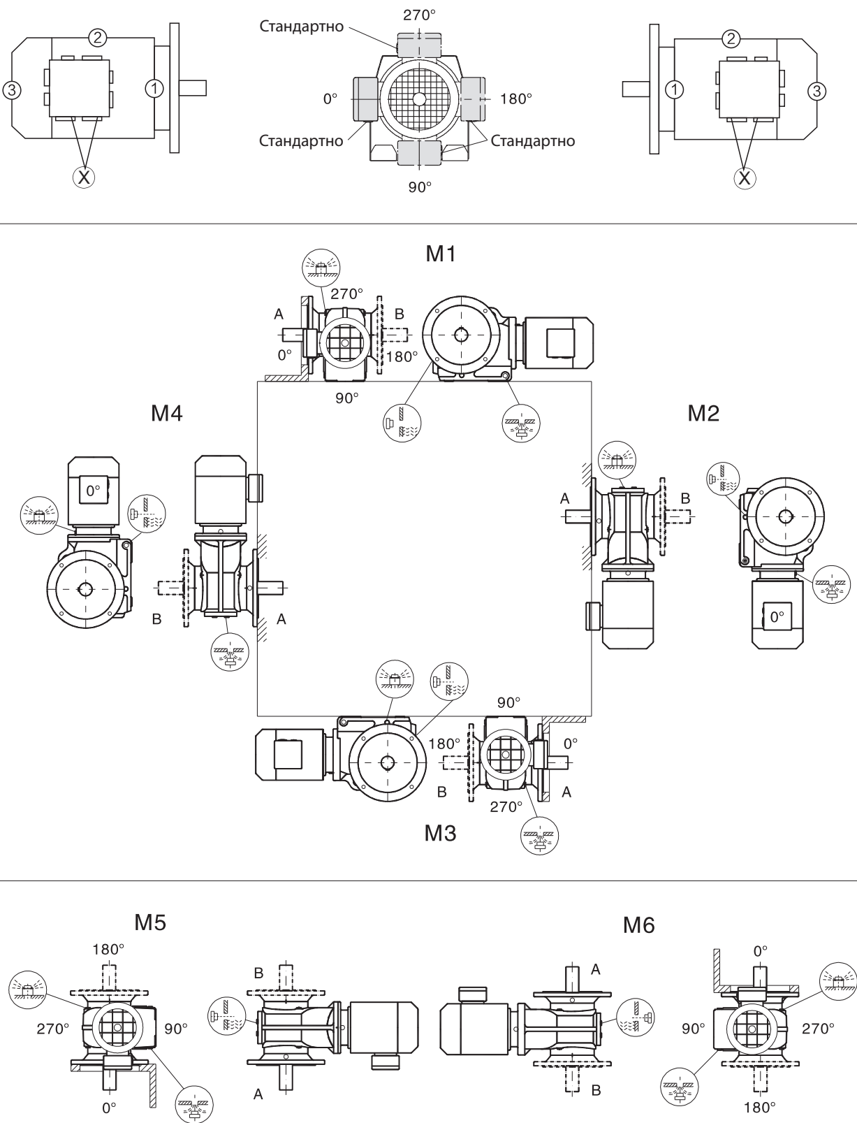
Пример монтажного положения
