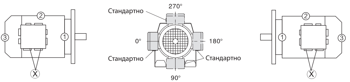
Пример монтажного положения
