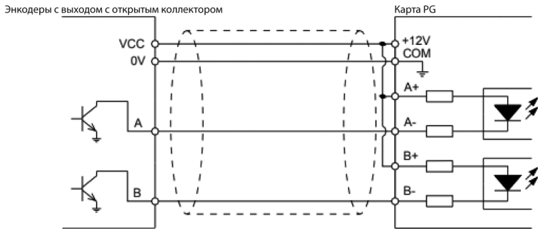
б) Электромонтажная схема энкодера с выходом с открытым коллектором
