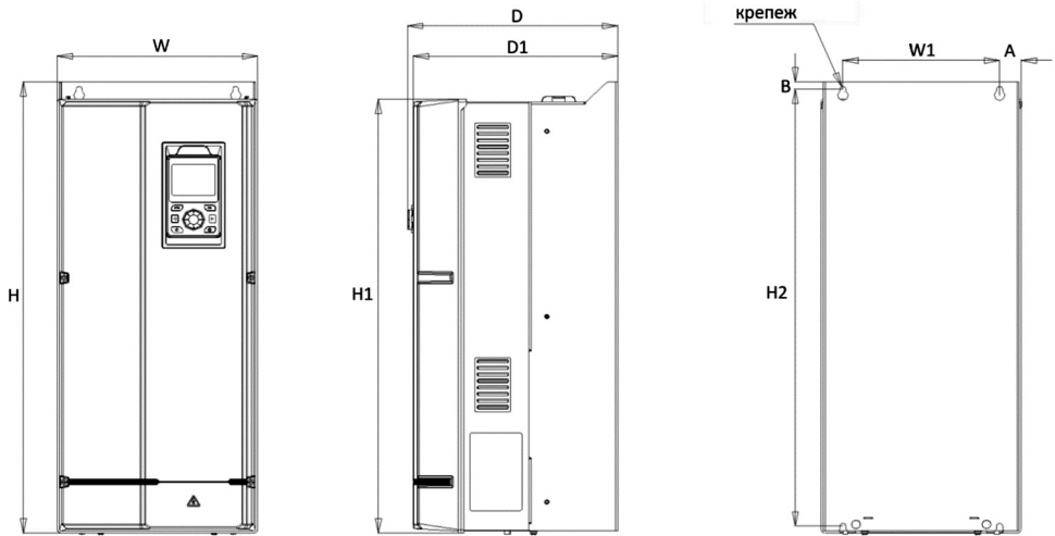
Рис. 3.6-2. Чертеж преобразователя частоты типоразмеров М4-М5
