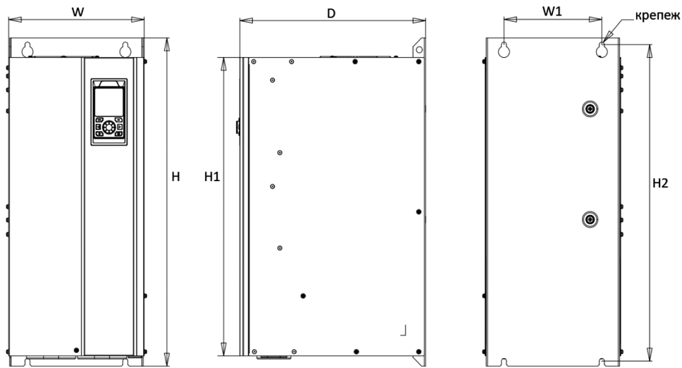
Рис. 3.6-3. Чертеж преобразователя частоты типоразмеров М6-М11
