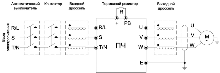
Рис. 4.1-1. Схема подключения преобразователя частоты
