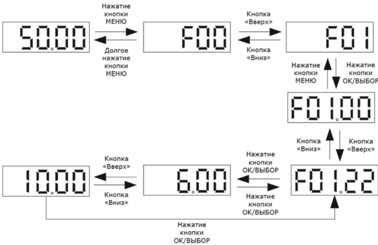
Рисунок 7.1-2. Базовые операции с панелью управления
