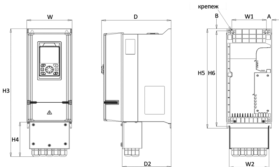
Рис. 3.6-4. Чертеж преобразователя частоты IP54 типоразмеров МН1-МН3
