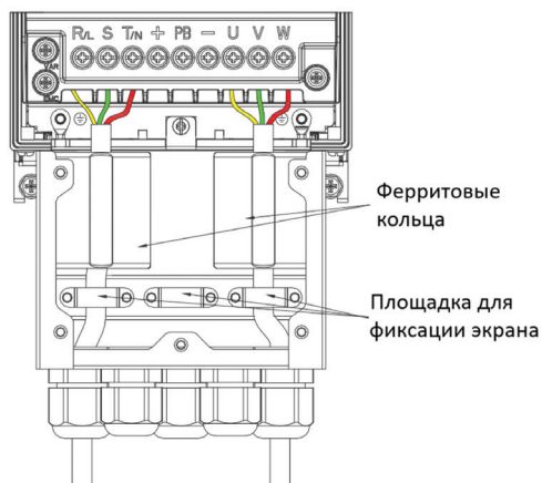
Рис. 3.6-7. Опции C2 для развязывающей панели
