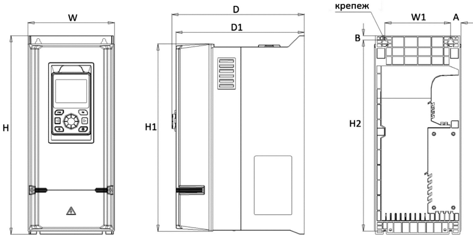
Рис. 3.6-1. Чертеж преобразователя частоты типоразмеров М1-М3
