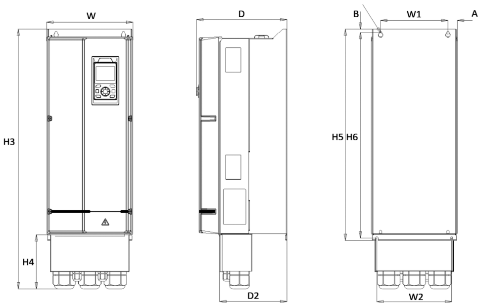
Рис. 3.6-5. Чертеж преобразователя частоты IP54 типоразмеров МН4-МН5
