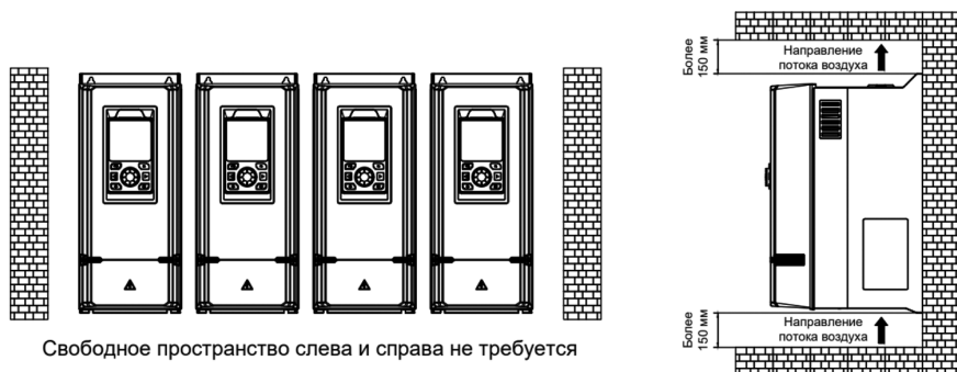
Рис. 3.5-1 Положение преобразователя частоты и требуемое пространство
