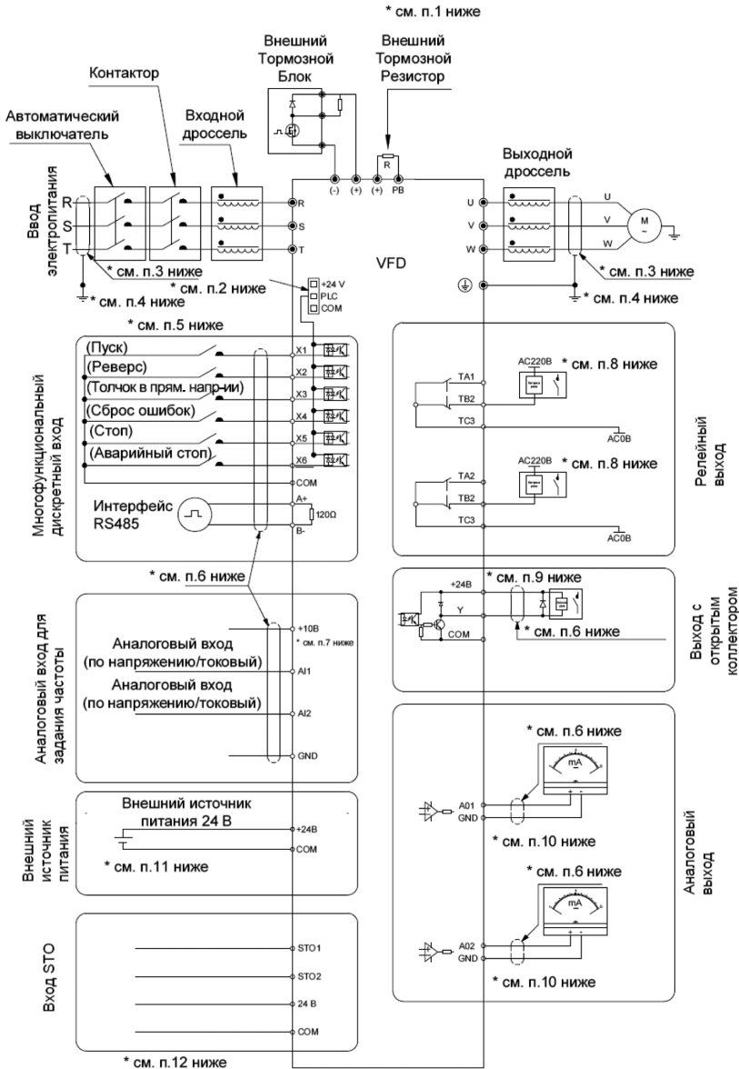
Рис. 4.2-1. Схема внешних подключений
