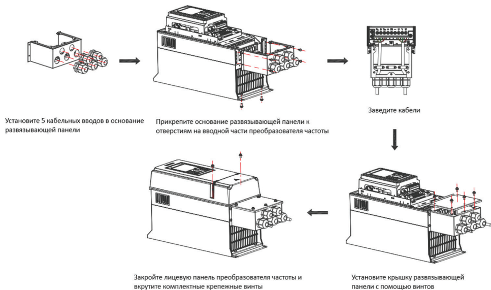
Рис. 3.6-6. Последовательность установки развязывающей панели
