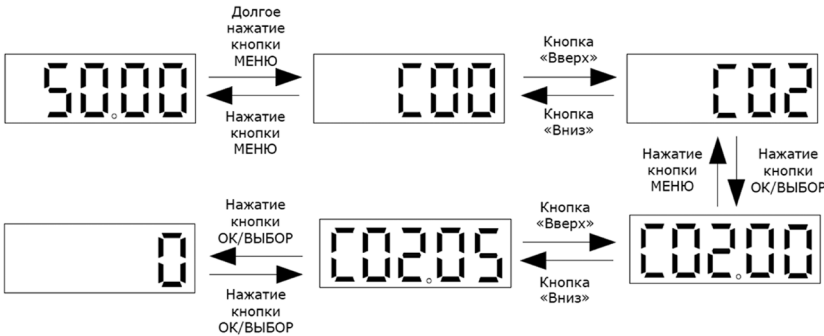
Рисунок 5.5-3. – Основные операции с панелью управления
