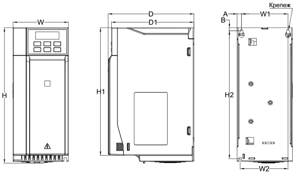
Рисунок 3.6-2 – Чертеж преобразователя частоты типоразмера В2
