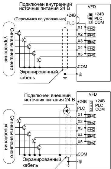
Рисунок 4.7-2. – Способ подключения логики NPN (перемычку между «+24 В» и «PLC» необходимо удалить, если осуществляется подключение внешнего питания 24 В)
