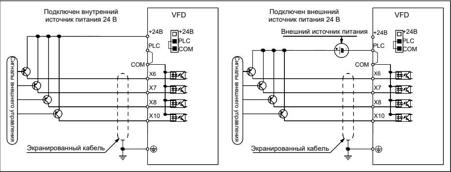
Рис. 2.1.2 Подключение PNP
