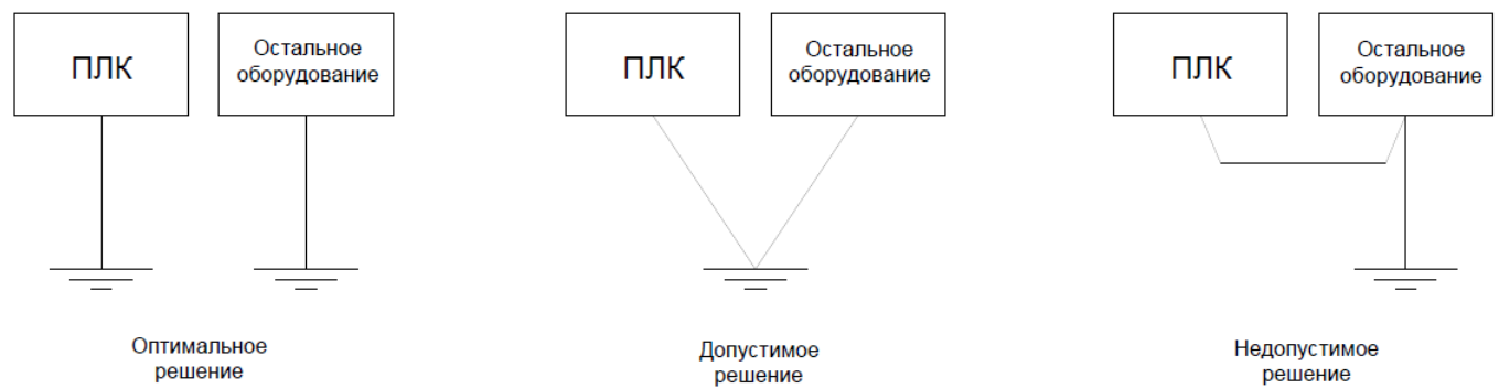
Рис. 5.3 Заземление ПЛК
