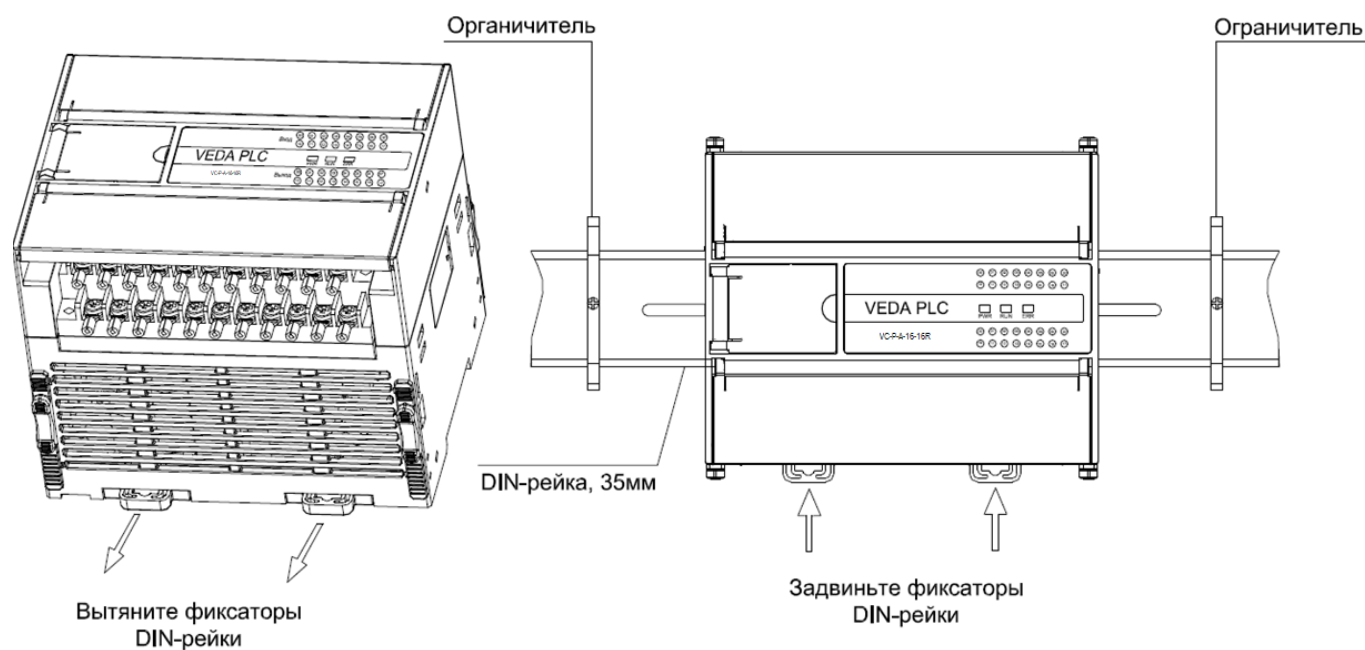
Рис. 5.2.1 Монтаж на DIN-рейку
