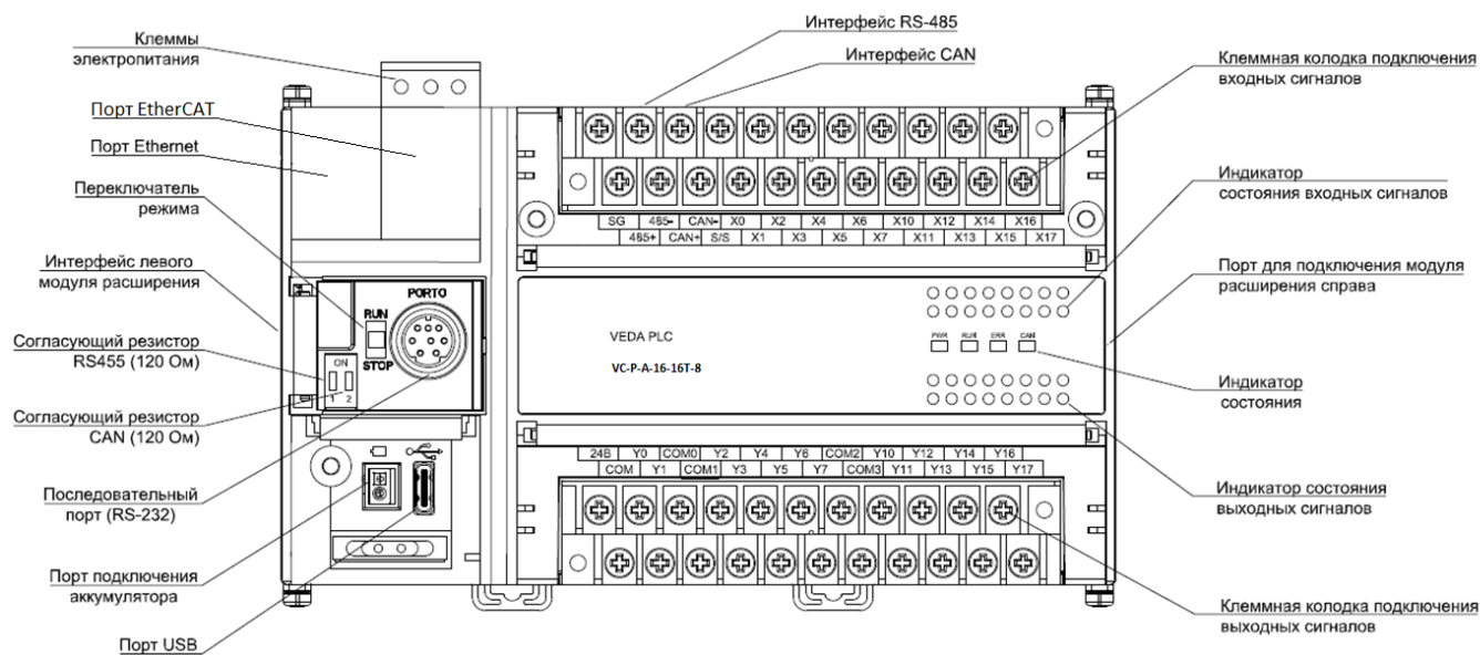
Рис. 1.2 Габаритный чертеж модуля серии VC-P
