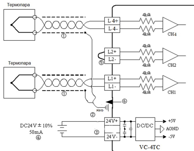
Рисунок 1-5. Электрическая схема подключения модуля VC-4TCO
