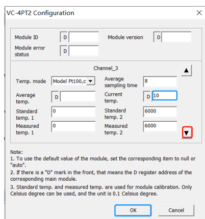
Рисунок 4-4 Настройка измерительного канала 3
