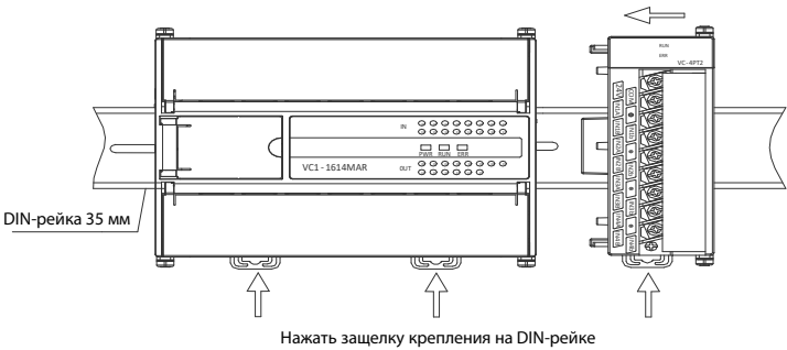
Рисунок 5-2 Монтаж модуля
