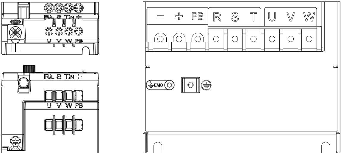
Рисунок 3.1-2 Расположение клемм
