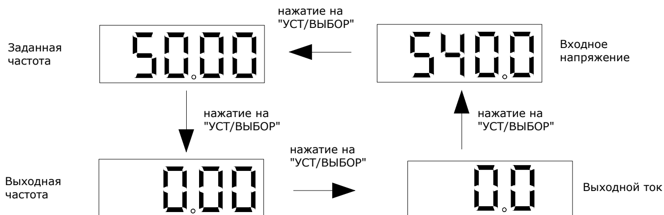
Рисунок 4.2-2 Переключение контролируемых параметров
