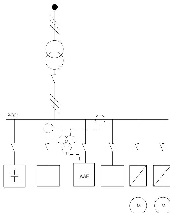
Рисунок 4.16 Конденсаторная батарея устанавливается со стороны РСС, а трансформаторы обеспечивают отсутствие измерения исправленного тока конденсатора.
