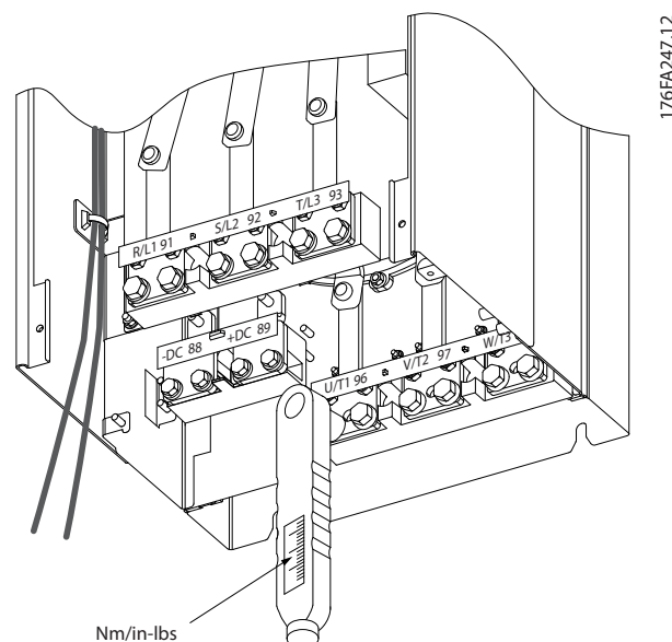
Рисунок 4.4 Для затягивания болтов используйте динамометрический ключ.
