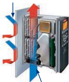
Конвекционное охлаждение
