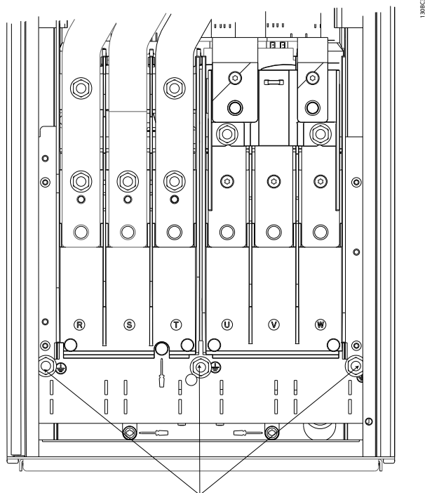
Рисунок 2.6 Заземление (зануление) для корпусов IP21/54.
