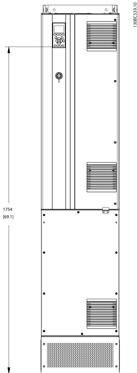
Рисунок 1.3 Корпус D7h
