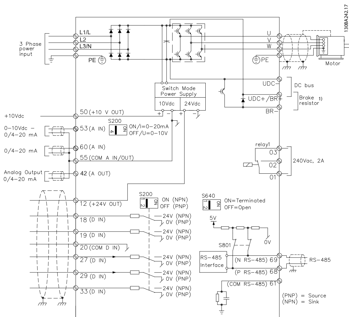
Рисунок 1.6 Схема электрических соединений всех клемм
