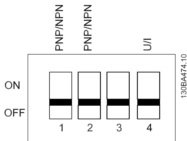
Рисунок 6.14 Переключатели S200, 1-4.
