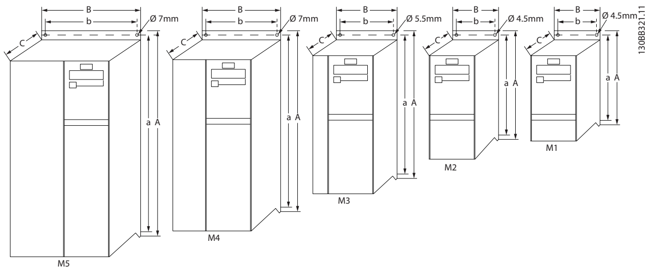
Рисунок 6.3 Габаритные размеры
