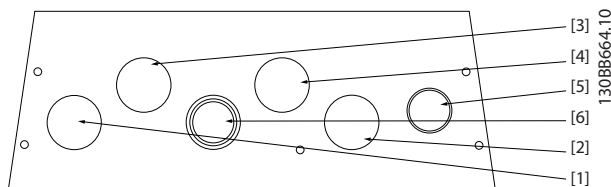
Рисунок 8.24 Размер корпуса A4, IP55, отверстия с резьбовыми уплотнениями
