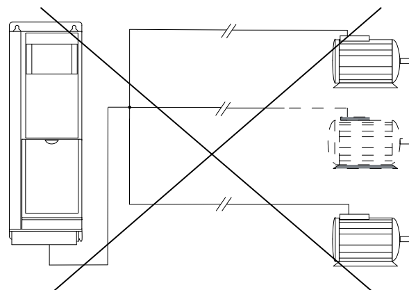
Рисунок 3.12 Подключение общим жгутом для кабелей большой длины
