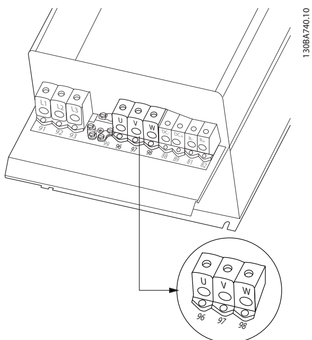
Рисунок 8.17 Подключение двигателя, корпуса C3 и C4
