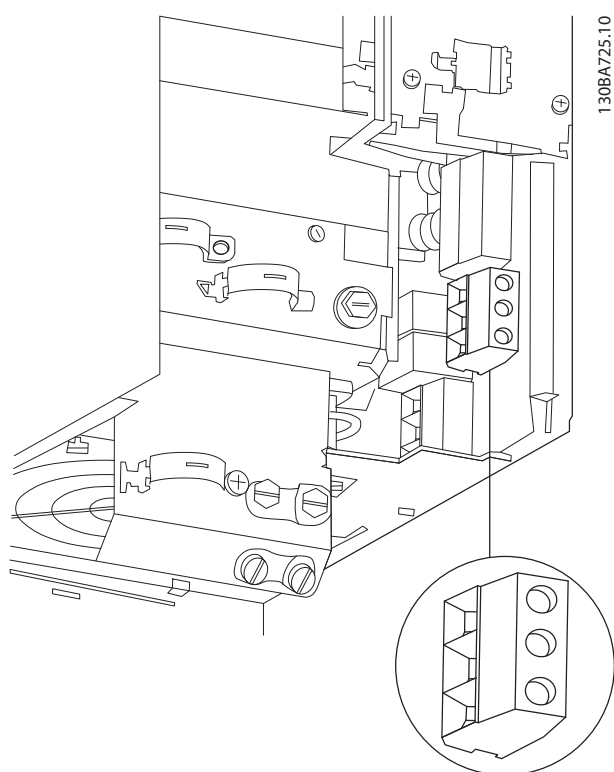
Рисунок 8.5 Подключение сети, корпус V3
