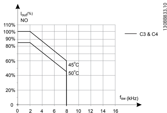
Рисунок 5.18 Снижение I_{\text{вых.}} при различных значениях T_{\text{окр.}} ср., МАКС. для корпусов размера C3 и C4, при использовании модели коммутации SFAVM в режиме нормальной перегрузки (крутящий момент 110 %)
