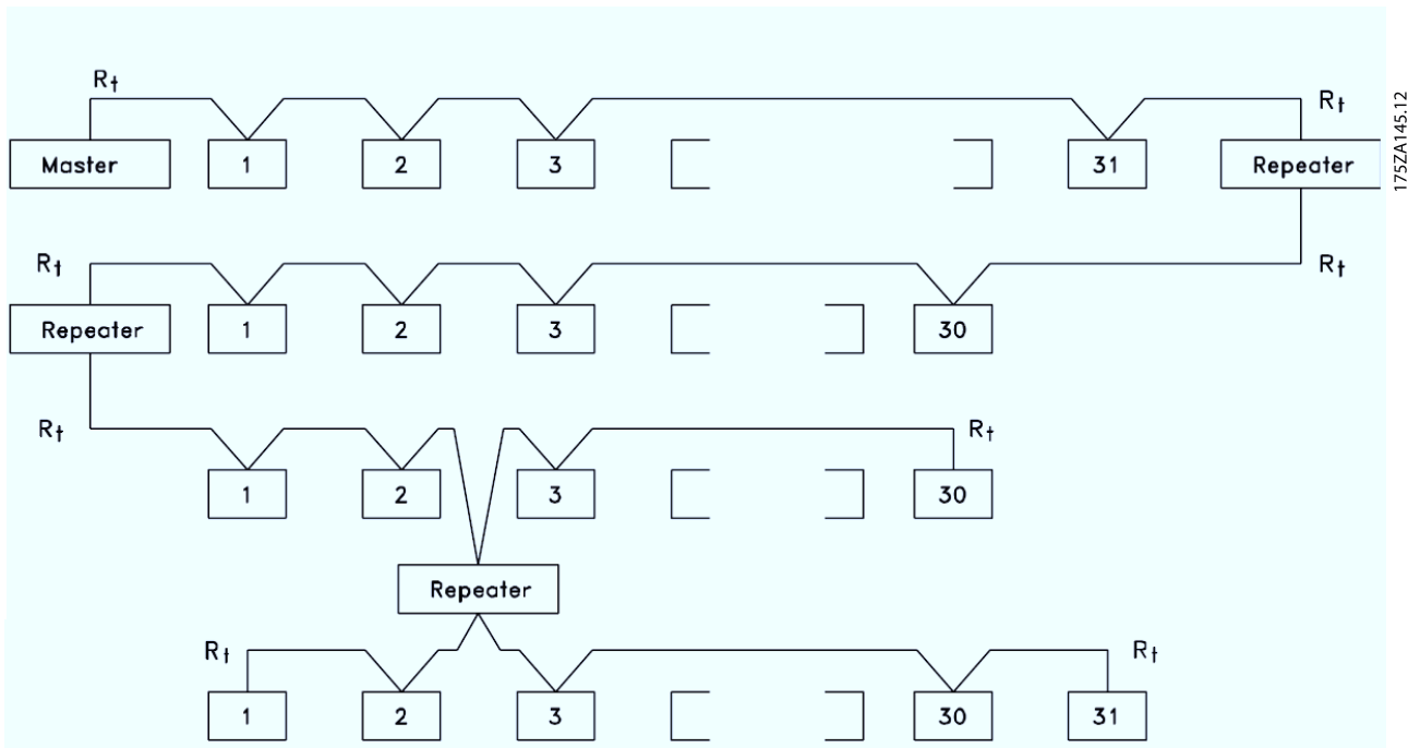
Рисунок 3.40 Интерфейс шины RS485
