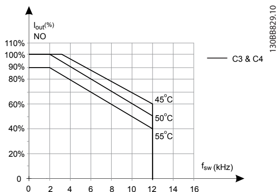
Рисунок 5.16 Снижение I_{\text{вых.}} при различных значениях T_{\text{окр.}} ср., МАКС. для корпусов размера C3 и C4, при использовании модели коммутации 60° AVM в режиме нормальной перегрузки (крутящий момент 110 %)
