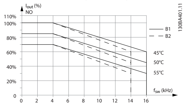
Рисунок 5.7 Снижение I_{\text{вых.}} при различных значениях T_{\text{окр.}} . СР., МАКС. для корпусов размера В1 и В2, при использовании модели коммутации 60° AVM в режиме нормальной перегрузки (перегрузка по крутящему моменту 110 %)
