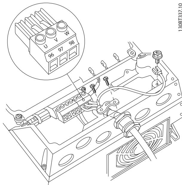
Рисунок 8.12 Подключение двигателя, корпуса A4/A5
