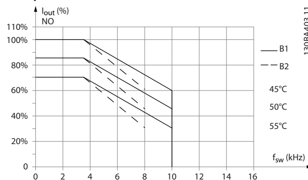
Рисунок 5.9 Снижение I_{\text{вых.}} при различных значениях T_{\text{окр.}} . СР., МАКС. для корпусов размера В1 и В2, при использовании модели коммутации SFAVM в режиме нормальной перегрузки (перегрузка по крутящему моменту 110 %).
