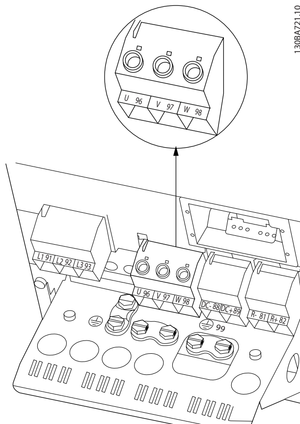
Рисунок 8.15 Подключение двигателя, корпус B4
