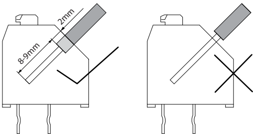
Рисунок 7.15 Монтаж кабелей
