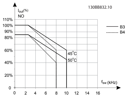
Рисунок 5.10 Снижение I_{\text{вых.}} при различных значениях T_{\text{окр.}} . СР., МАКС. для корпусов размера В3 и В4, при использовании модели коммутации SFAVM в режиме нормальной перегрузки (перегрузка по крутящему моменту 110 %)
