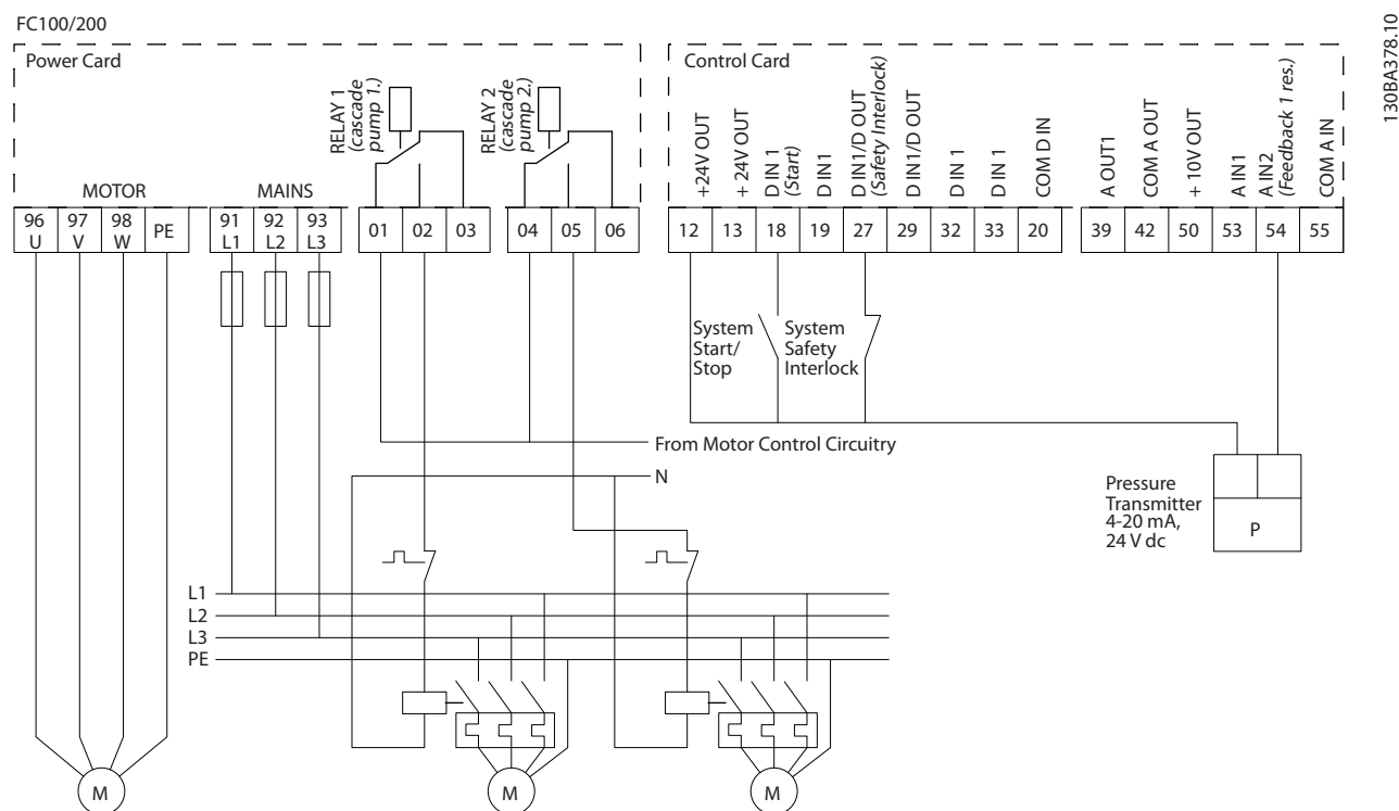
Рисунок 4.11 Схема электрических соединений каскадного контроллера
