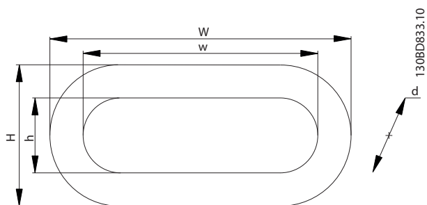
Рисунок 6.4 Сердечник HF-СМ
