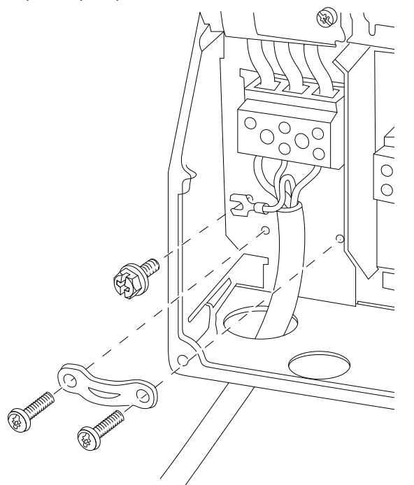
Рисунок 8.4 Подключение сети, корпуса B1 и B2
