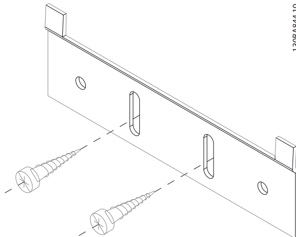
Рисунок 3.38 Нижний кронштейн
