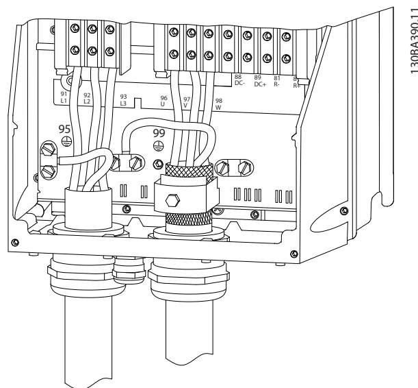
Рисунок 8.16 Подключение двигателя, корпуса C1 и C2 (IP21/NEMA Тип 1 и IP55/66/NEMA Тип 12)
