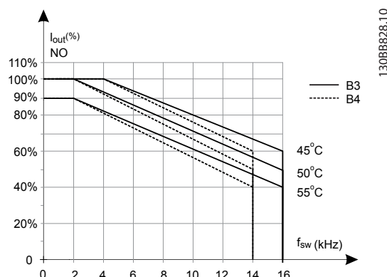
Рисунок 5.8 Снижение I_{\text{вых.}} при различных значениях T_{\text{окр.}} . СР., МАКС. для корпусов размера В3 и В4, при использовании модели коммутации 60° AVM в режиме нормальной перегрузки (перегрузка по крутящему моменту 110 %)
