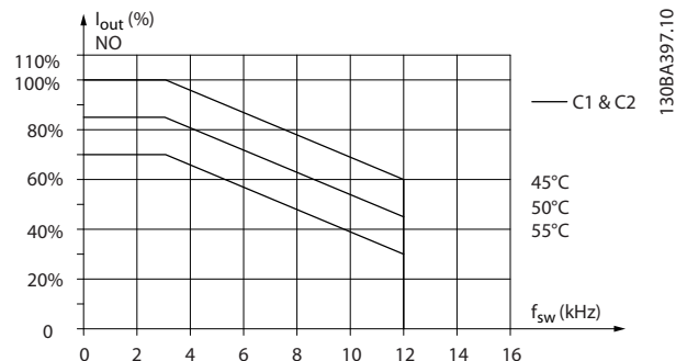
Рисунок 5.15 Снижение I_{\text{вых.}} при различных значениях T_{\text{окр.}} ср., МАКС. для корпусов размера C1 и C2, при использовании модели коммутации 60° AVM в режиме нормальной перегрузки (перегрузка по крутящему моменту 110 %)
