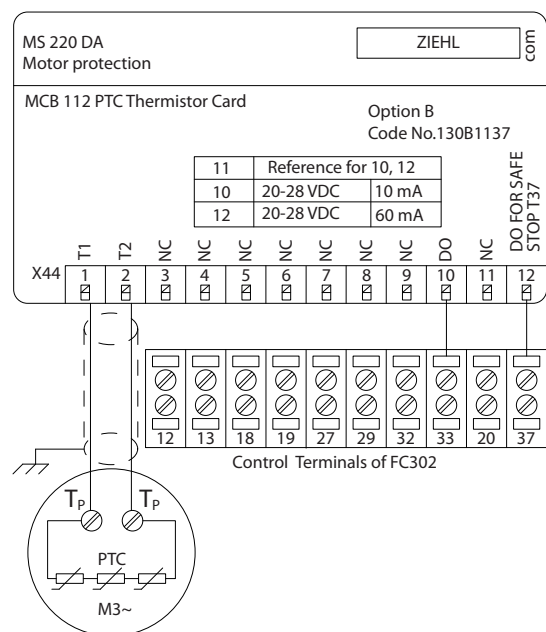
Рисунок 7.9 Монтаж MCB 112
