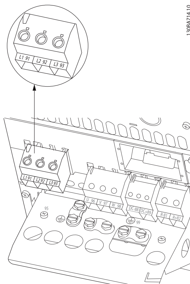
Рисунок 8.6 Подключение сети, корпус V4
