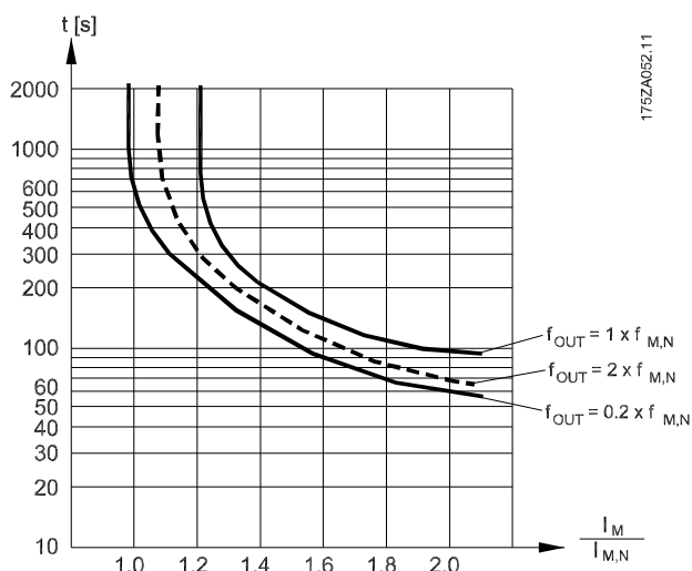
Рисунок 3.15 Профиль ЭТР
