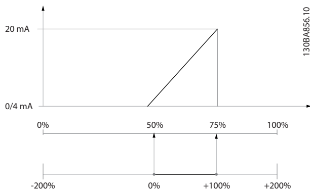
Рисунок 3.38 Пример 2
