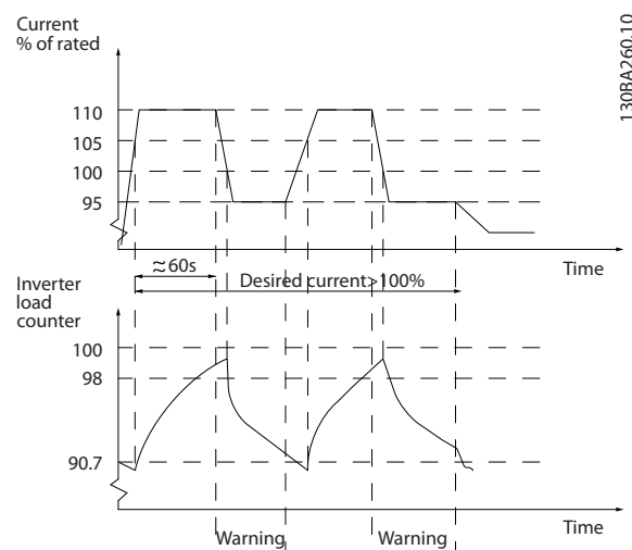
Рисунок 3.55 Выходной ток в условиях перегрузки
