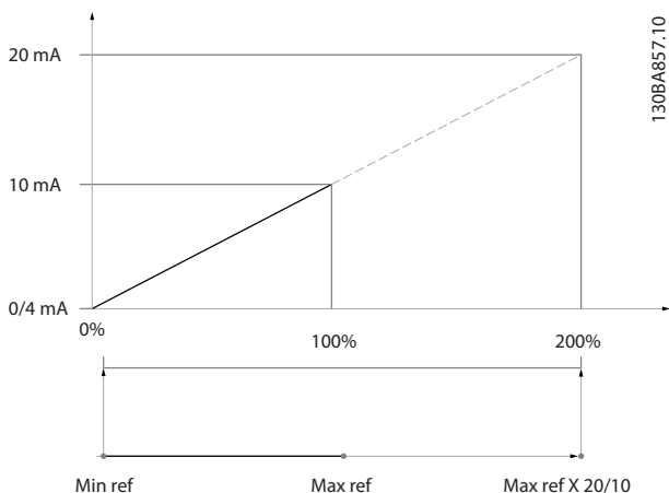
Рисунок 3.39 Пример 3
