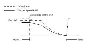
Рисунок 3.53 Кинетический резерв, более длительное замыкание сети
