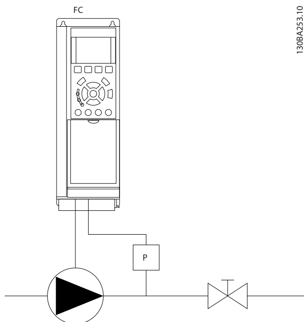
Рисунок 3.64 Схема обнаружения отсутствия потока
