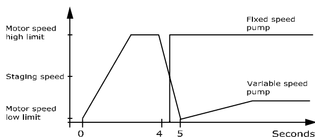
Рисунок 3.90 Порог включения
