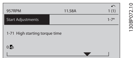
Рисунок 2.21 Сохранение
