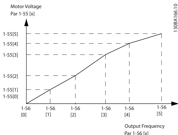
Рисунок 3.9 Характеристика U/f
