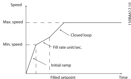
Рисунок 3.111 Вертикальная трубопроводная система
