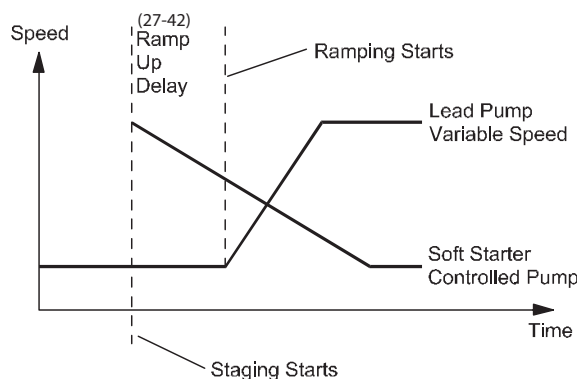
Рисунок 3.106 Задержка при разгоне
