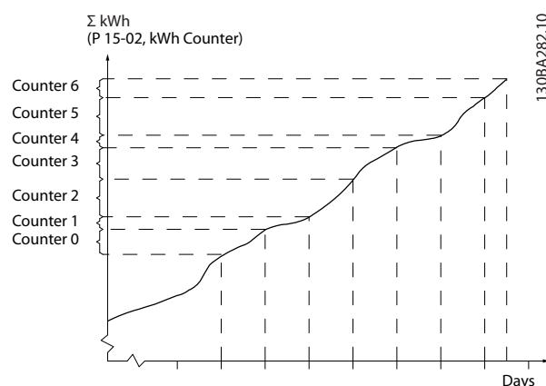
Рисунок 3.75 График энергопотребления
