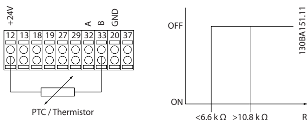
Рисунок 3.16 Подключение термистора
