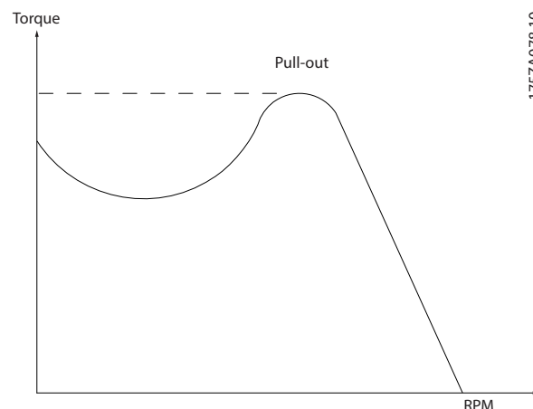
Рисунок 1.1 Момент срыва
