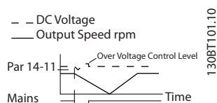
Рисунок 3.50 Управляемое замедление, короткое замыкание сети.
