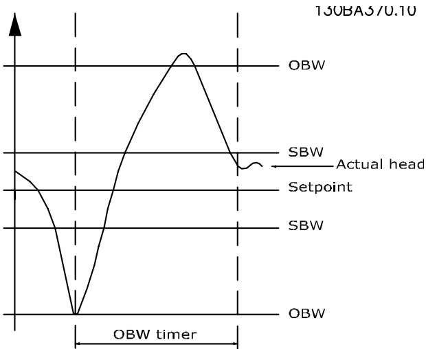
Рисунок 3.86 Время блокирования
