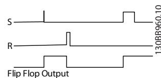
Рисунок 3.43 Выходы триггеров
