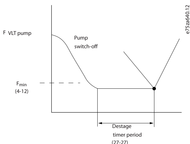
Рисунок 3.87 Задержка выключения
