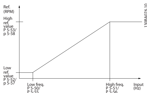
Рисунок 3.31 Импульсный вход
