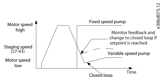
Рисунок 3.107 Порог включения
