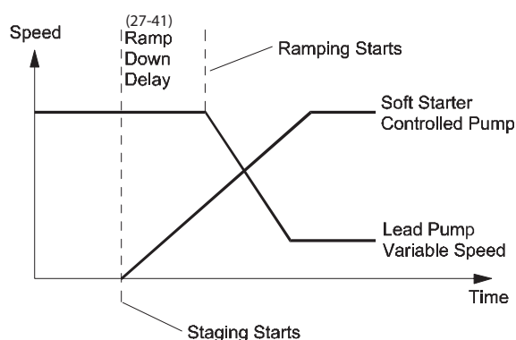
Рисунок 3.105 Задержка при замедлении
