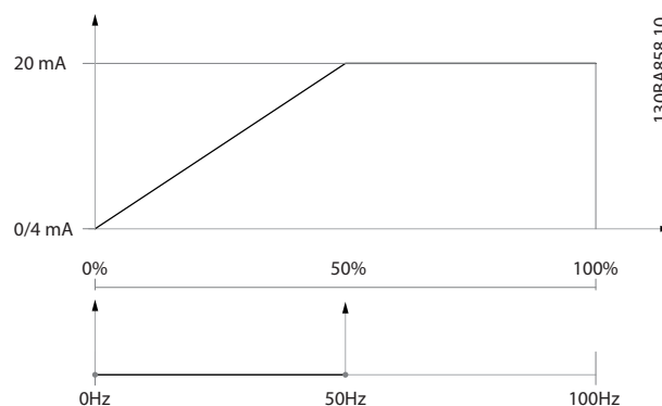
Рисунок 3.37 Пример 1
