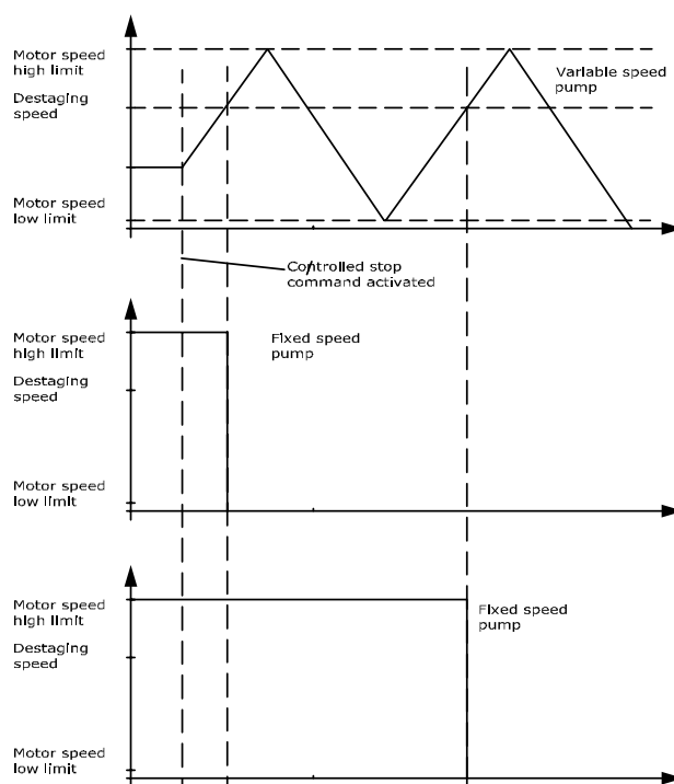
Рисунок 3.92 Скорости выключения
