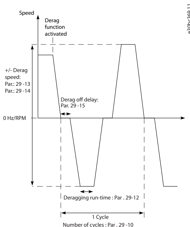
Рисунок 3.112 Функция очистки
