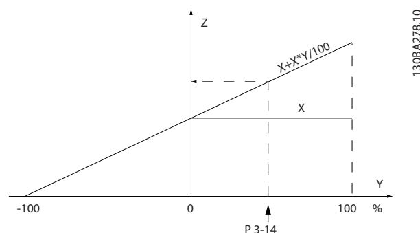
Рисунок 3.20 Фактическое задание
