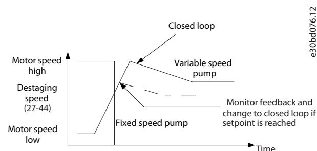
Рисунок 3.108 Порог выключения
