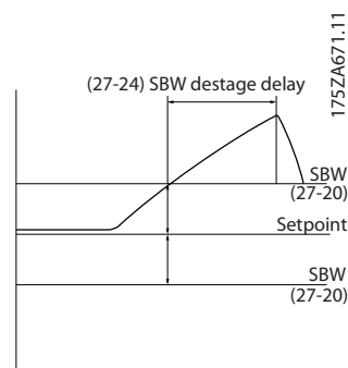
Рисунок 3.98 Задержка включения след. насоса (таймер)
