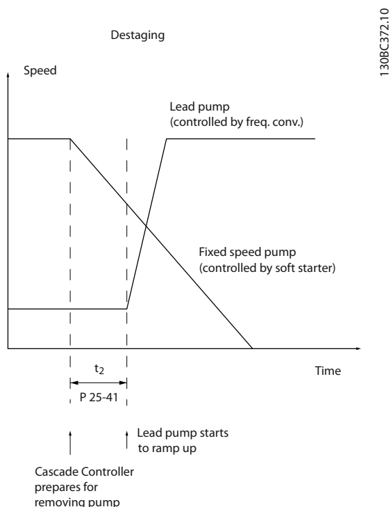
Рисунок 3.89 Выключение
