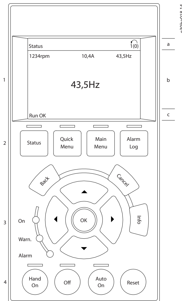
Рисунок 2.1 LCP
