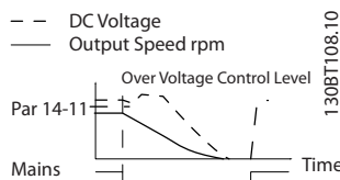
Рисунок 3.51 Управляемое замедление, более длительное замыкание цепи.
