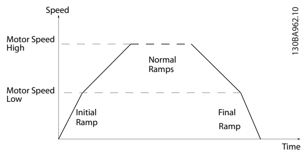
Рисунок 3.23 Время начального и конечного изменения скорости
