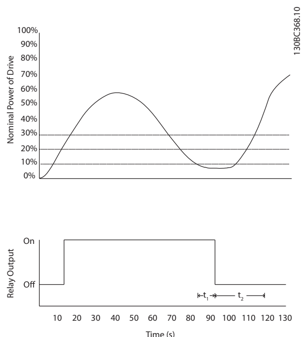
Рисунок 3.33 Пример выходной функции
