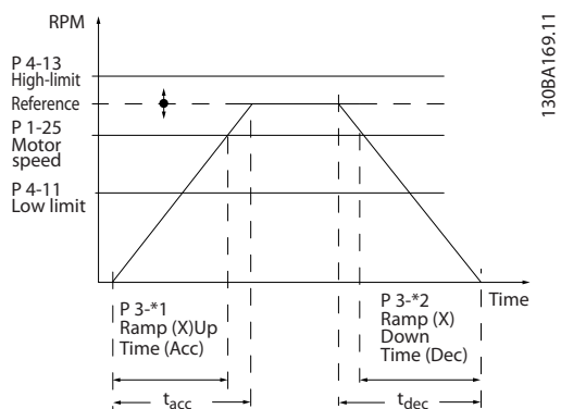
Рисунок 3.21 Изменение скорости 1
