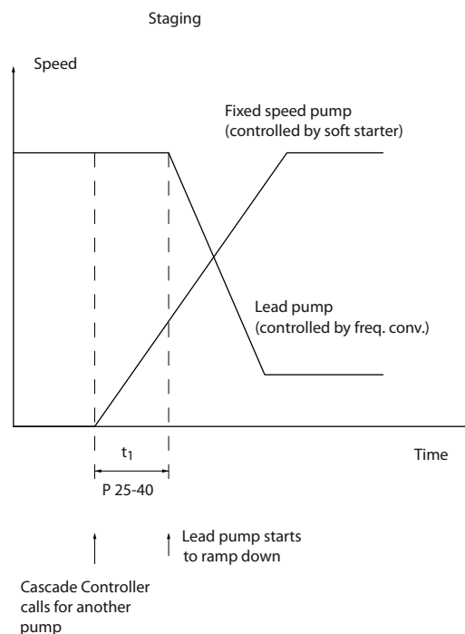
Рисунок 3.88 Включение
