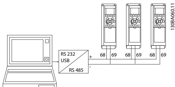
Рисунок 5.104 Параллельные подключения
