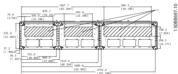
Рисунок 5.43 Типоразмер F13
