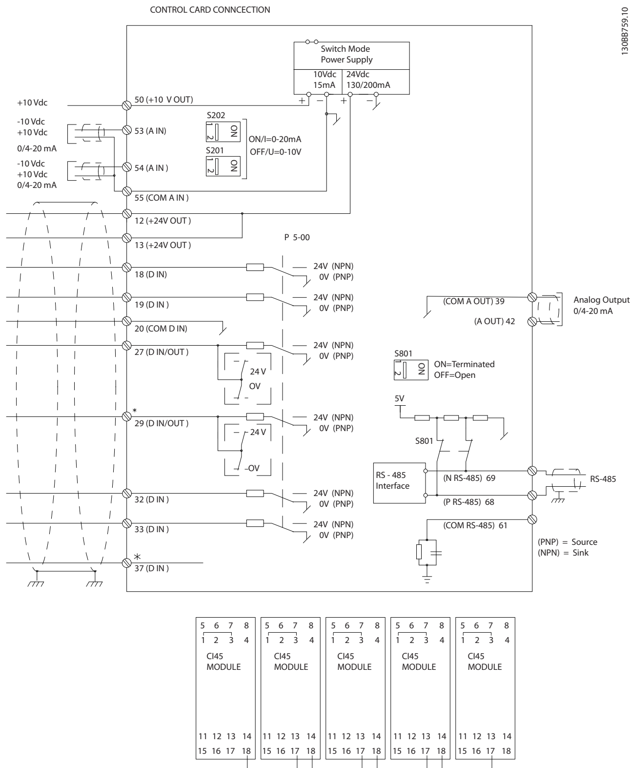
Рисунок 5.55 Схема кабеля управления
