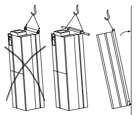
Рисунок 5.7 Рекомендуемый метод подъема, типоразмер E
