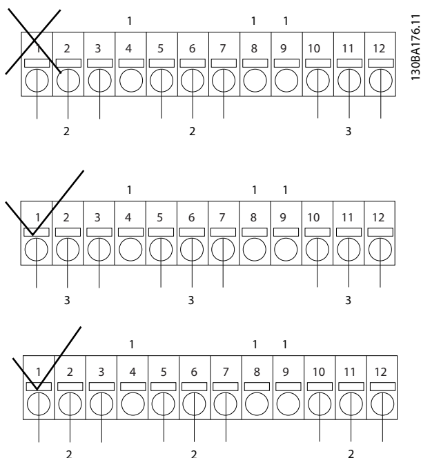
Рисунок 3.15 Клеммы
