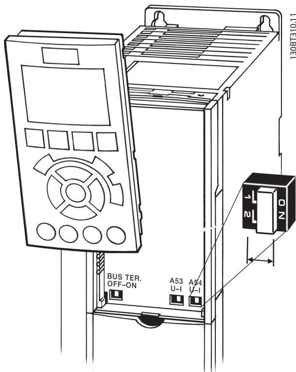
Рисунок 5.59 Расположения переключателей
