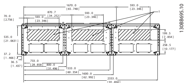
Рисунок 5.41 Типоразмер F11
