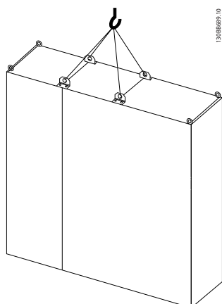
Рисунок 5.9 Рекомендуемый метод подъема, типоразмеры F3, F4, F11, F12 и F13
