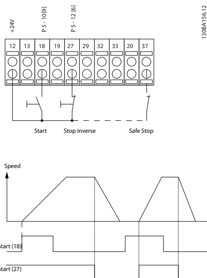
Рисунок 5.51 Клемма 37 предусматривается только с функцией безопасного останова!
