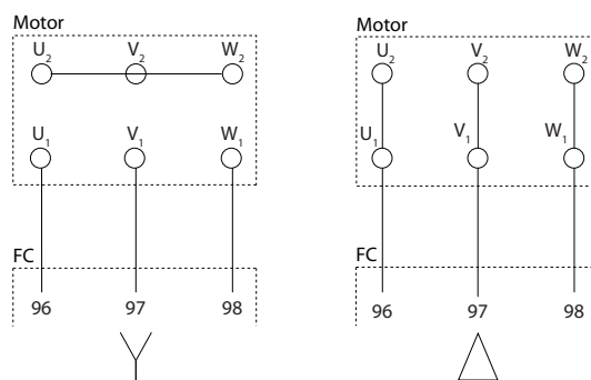
Рисунок 5.45 Подключение кабеля электродвигателя
