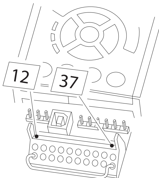
Рисунок 5.102 Перемычка между клеммой 37 и напряжением 24 В пост. тока
