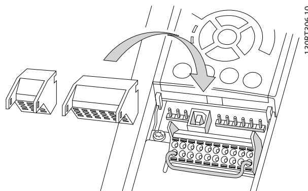
Рисунок 5.50 Клеммы управления
