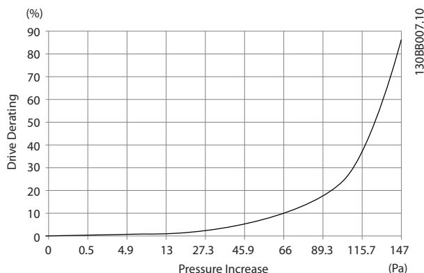
Рисунок 5.24 Снижение номинальных характеристик в корпусах D в зависимости от изменения давления Воздушный поток преобразователя частоты: 450 куб. футов/мин (765 м³/ч)
