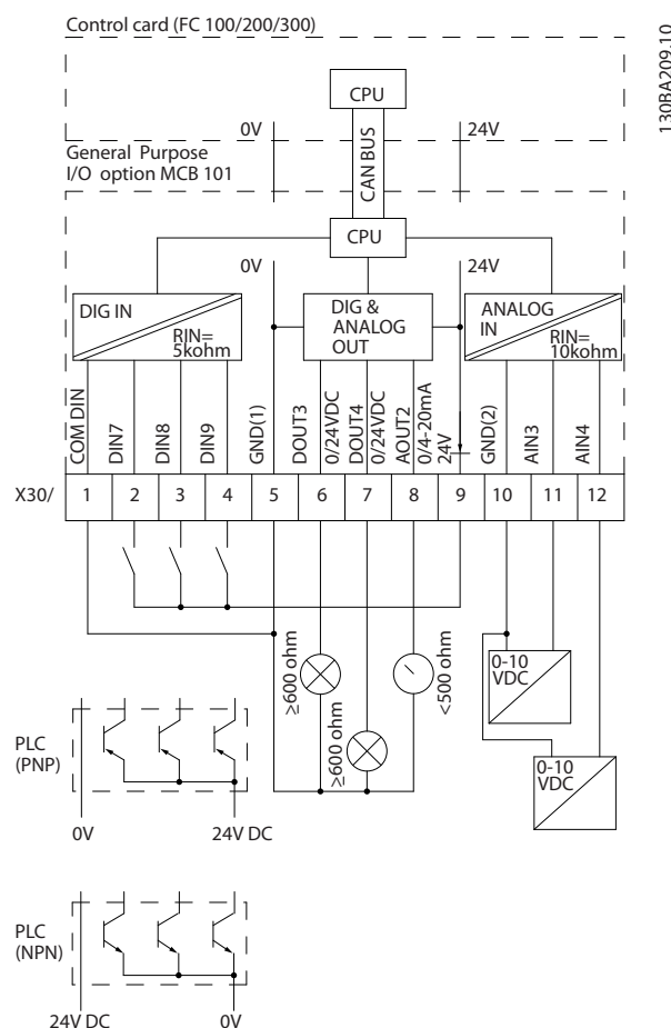
Рисунок 3.7 Принципиальная схема
