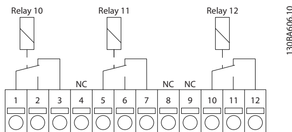
Рисунок 3.13 Присоединение проводов к клеммам
