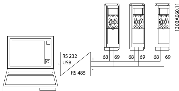
Рисунок 7.3 Параллельные подключения
