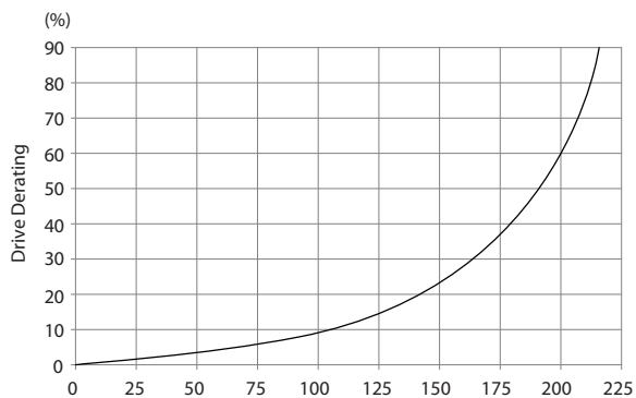
Рисунок 5.27 Снижение номинальных характеристик для корпусов F1, F2, F3, F4 в зависимости от изменения давления Воздушный поток преобразователя частоты: 580 куб. футов/мин (985 м³/ч)
