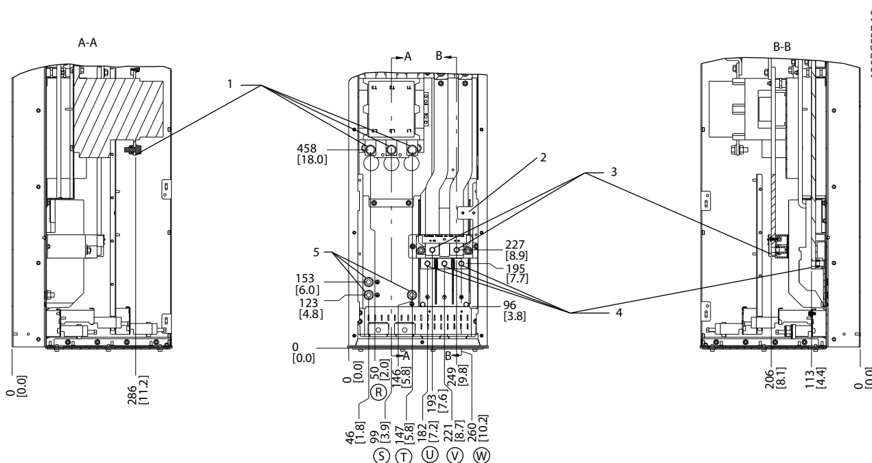
Рисунок 5.68 Расположение клемм, D6h с контактором
