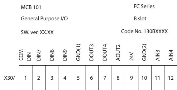
Рисунок 3.6 MCB 101
