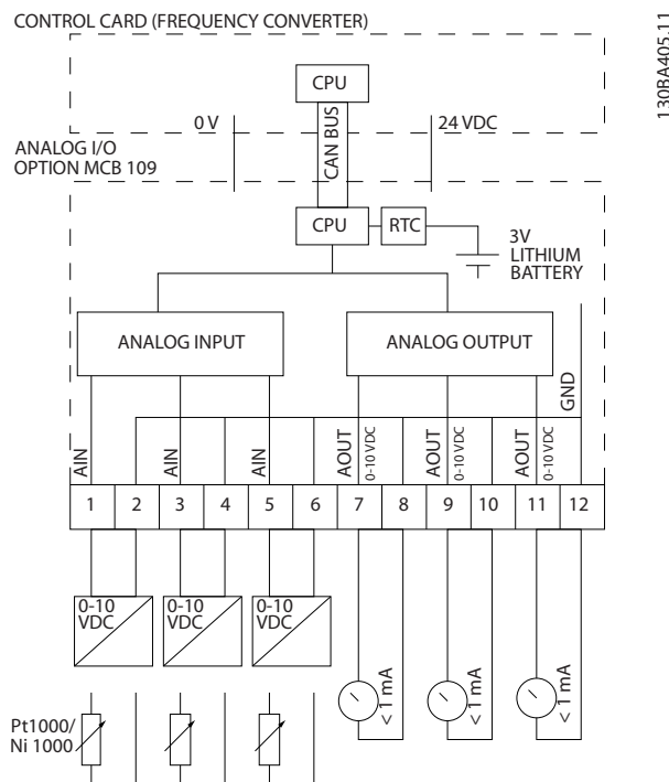
Рисунок 3.11 Принципиальная схема аналоговых входов/выходов, предусмотренных в преобразователе частоты
