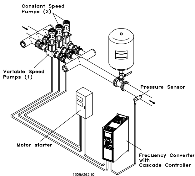
Рисунок 6.7 Каскадный контролер BASIC
