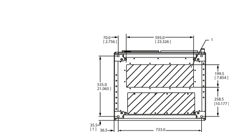
Рисунок 5.38 Типоразмер F8
