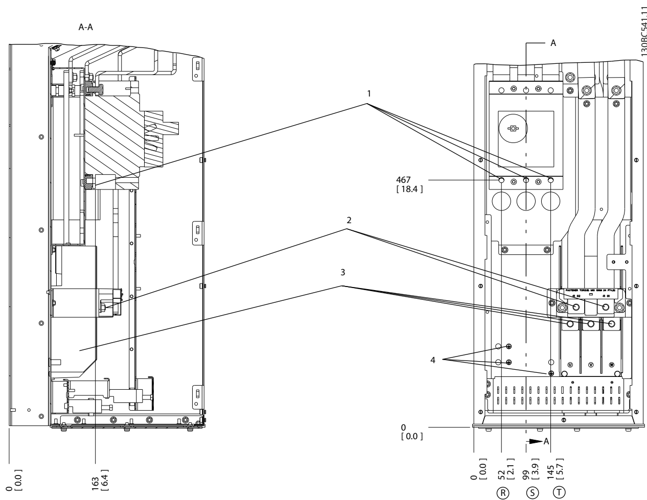
Рисунок 5.70 Расположение клемм, D6h с автоматическим выключателем
