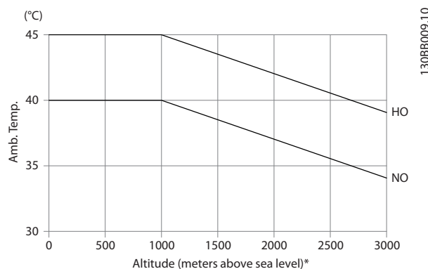
Рисунок 3.4 Снижение выходного тока в зависимости от высоты над уровнем моря при температуре окружающей среды T_{AMB, MAX}
