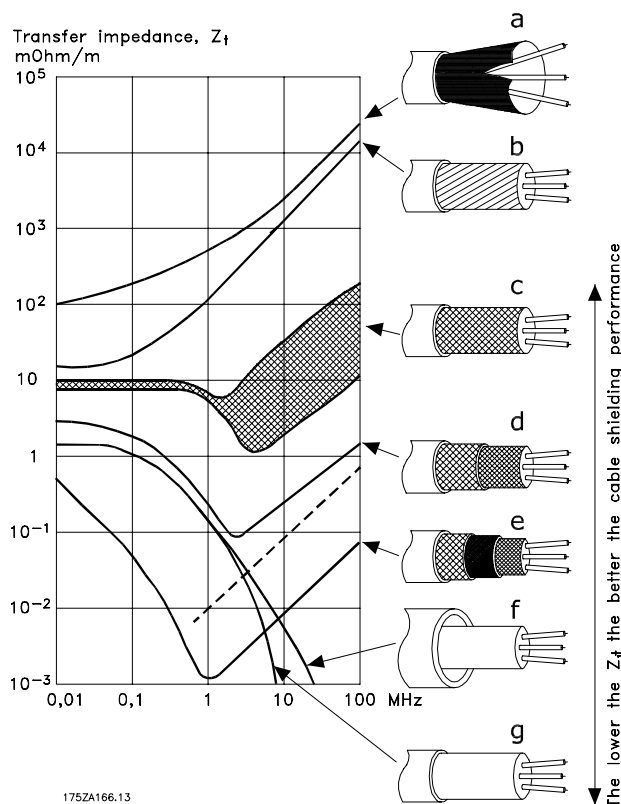
Рисунок 5.108 Передаточный импеданс Z_T
