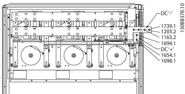
Рисунок 5.86 Расположение клемм — Клеммы генераторного режима — F2 и F4
