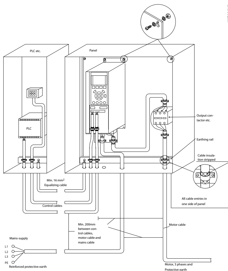
Рисунок 5.106 Корректный по ЭМС электрический монтаж преобразователя частоты в шкафу
