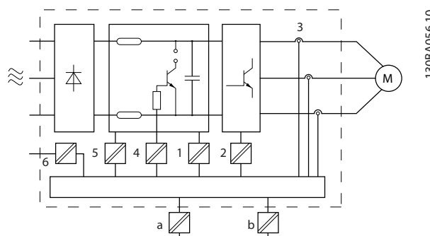
Рисунок 2.20 Гальваническая развязка
