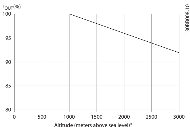
Рисунок 3.3 Снижение выходного тока в зависимости от высоты над уровнем моря при температуре окружающей среды T_{AMB, MAX}
