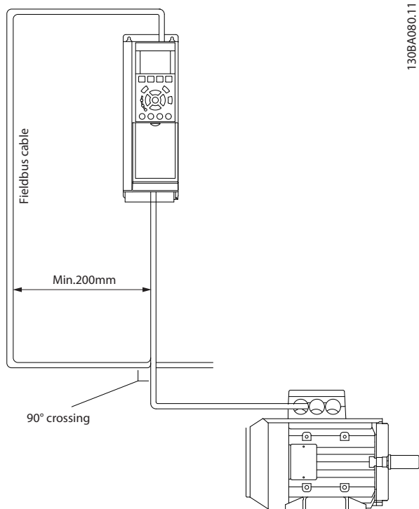
Рисунок 7.2 Обеспечение ЭМС
