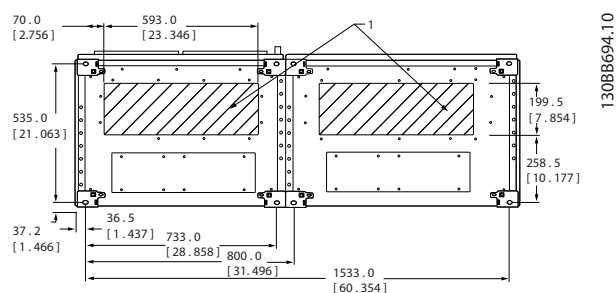
Рисунок 5.40 Типоразмер F10
