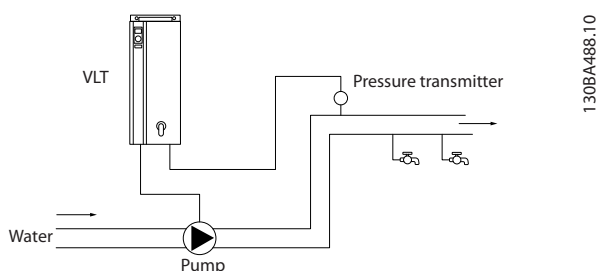
Рисунок 2.16 ПИД-регулятор с замкнутым контуром
