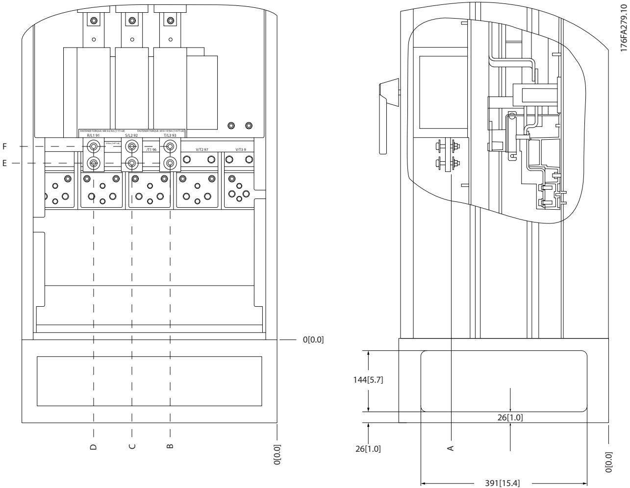
Рисунок 5.78 Расположение расцепителя питания на корпусе IP21 (NEMA тип 1) и IP54 (NEMA тип 12)
