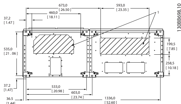
Рисунок 5.39 Типоразмер F9
