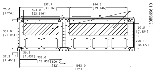
Рисунок 5.42 Типоразмер F12
