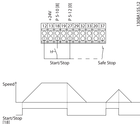
Рисунок 6.1 Клемма 37: предусматривается только с функцией безопасного останова!
