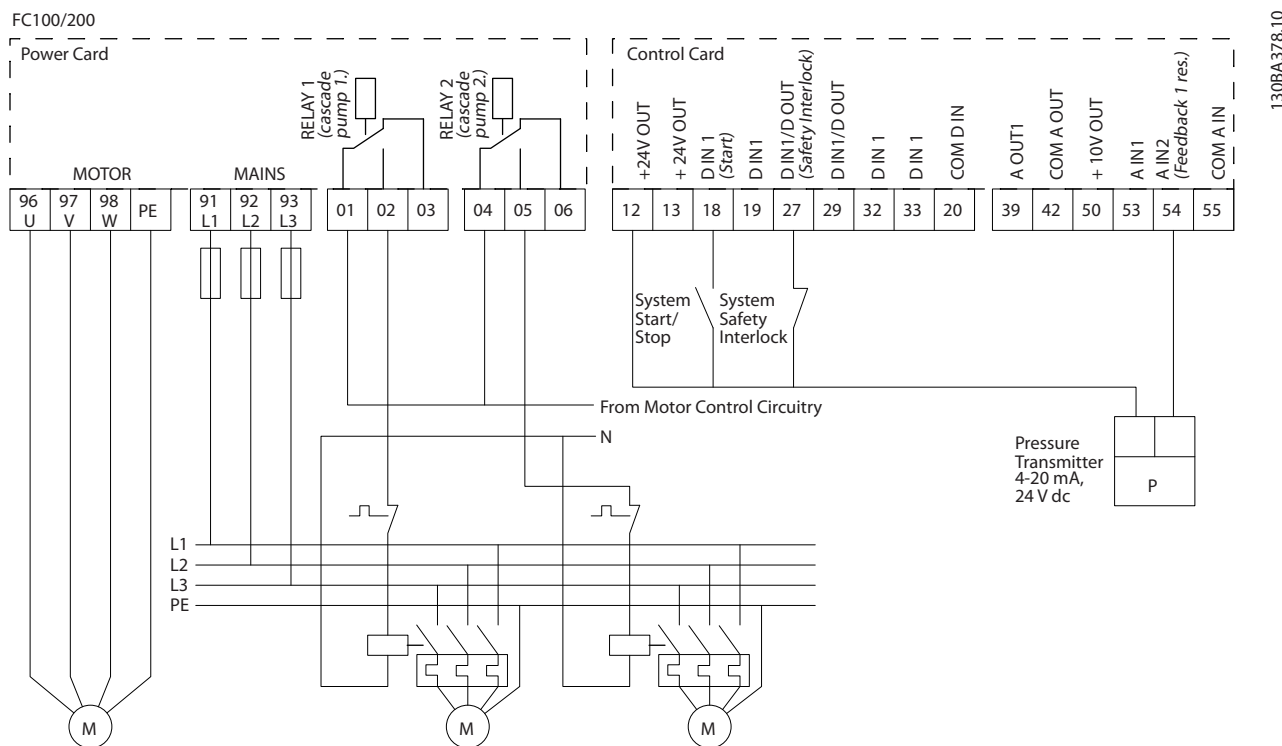
Рисунок 6.9 Схема электрических соединений каскадного контролера
