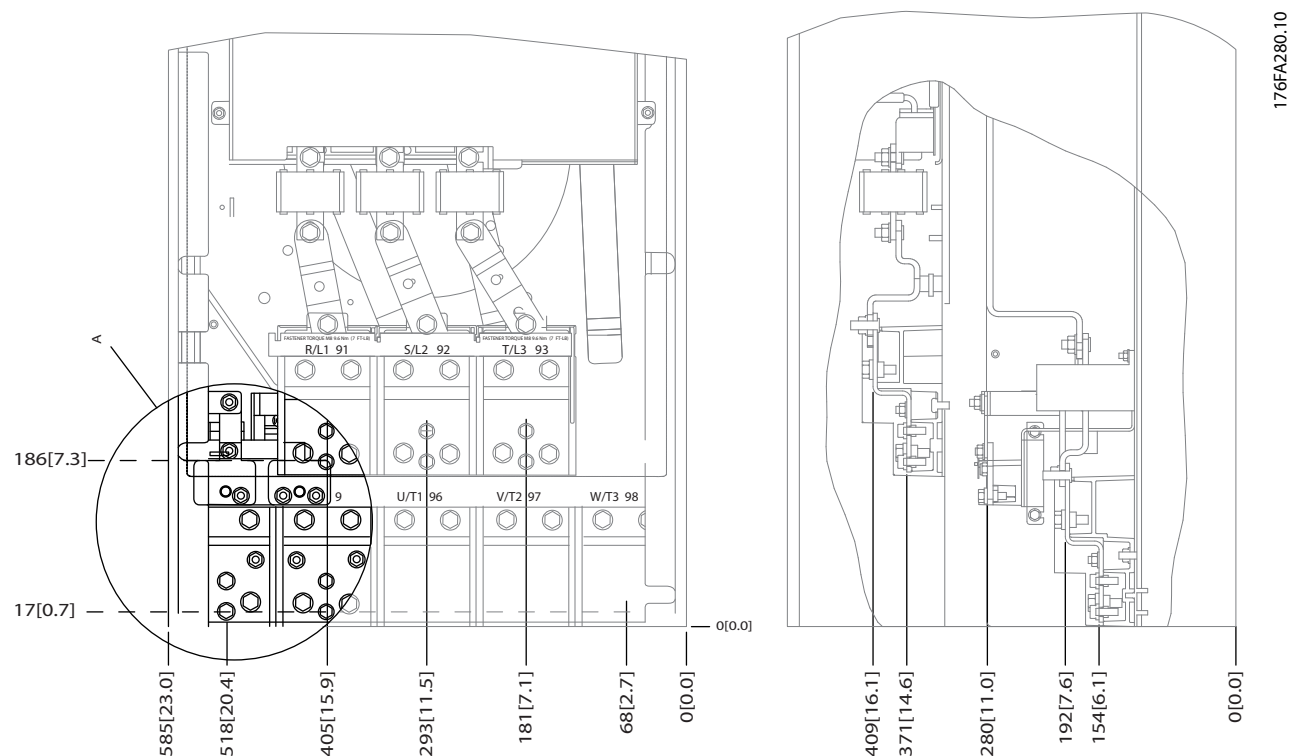
Рисунок 5.79 Расположение клемм электропитания корпусов IP00
