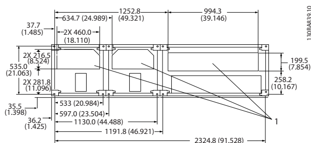
Рисунок 5.37 F4, вид снизу
