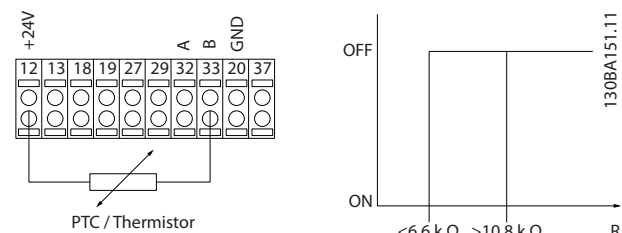
Рисунок 2.28 Цифровой вход и источник питания 24 В
