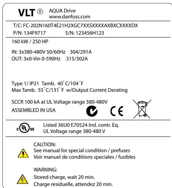
Рисунок 5.5 Паспортная табличка
