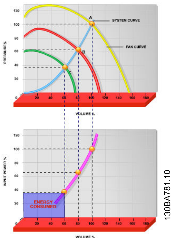
Рисунок 2.2 Энергосбережение
