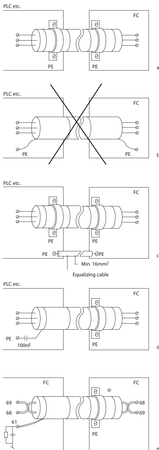
Рисунок 5.109 Заземление
