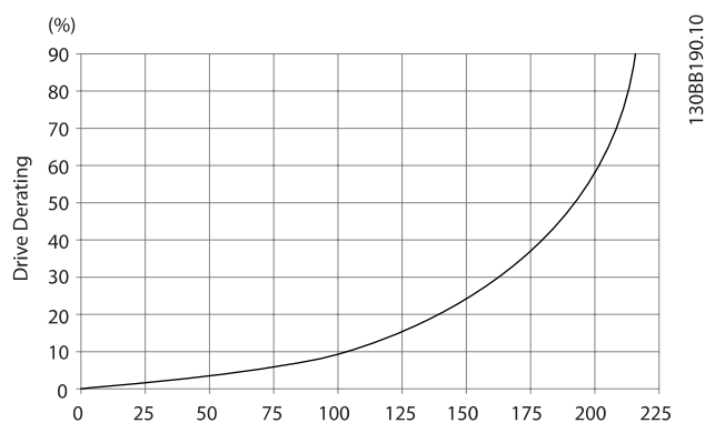
Рисунок 4.23: Корпус F, снижение значений относит. Изменение давления Воздушный поток привода: 580 куб. футов/мин (985 м³/час)
