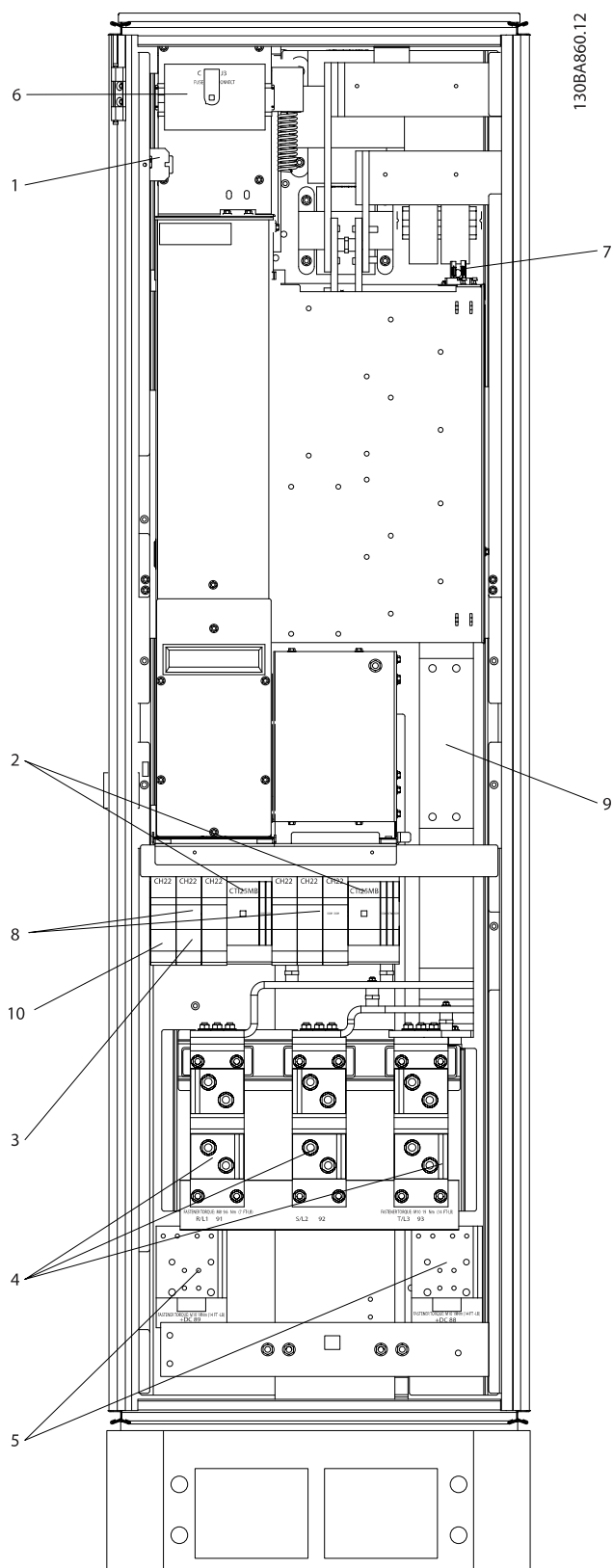
Рисунок 4.31: Шкаф выпрямителя, размер корпуса F17
