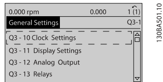
Рисунок 6.6: Шаг 5: С помощью навигационных кнопок "вверх"/"вниз" выберите, например, Q3-12 Аналоговые выходы . Нажмите [OK].
