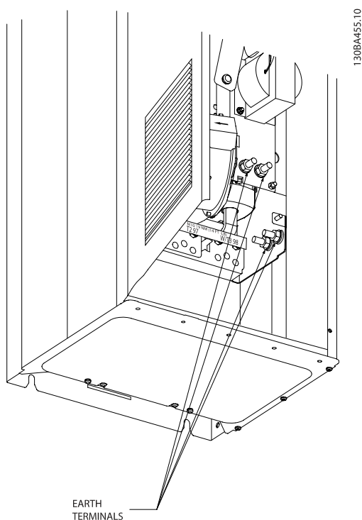
Рисунок 4.28: Расположение клемм заземления (секция привода)
