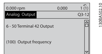
Рисунок 6.7: Шаг 6: Выберите параметр 6-50 Клемма 42, выход . Нажмите [OK].
