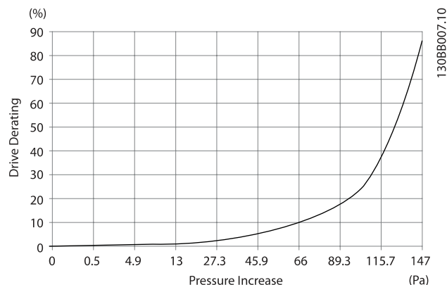
Рисунок 4.20: Корпус D Снижение значений относит. Изменение давления
