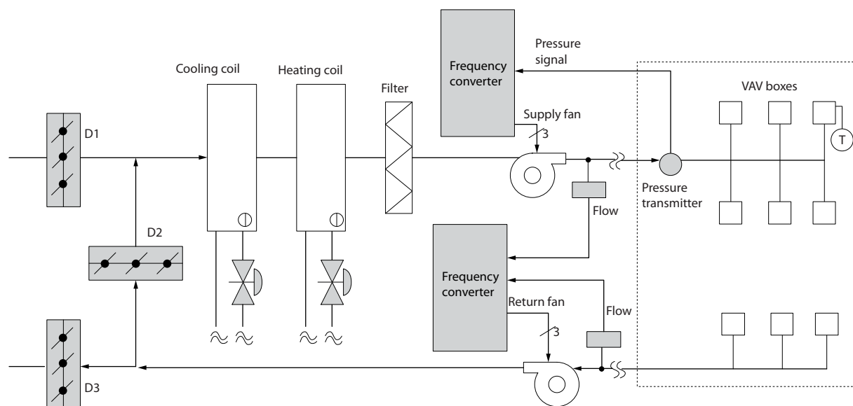
Рисунок 3.11 Переменный объем воздуха
