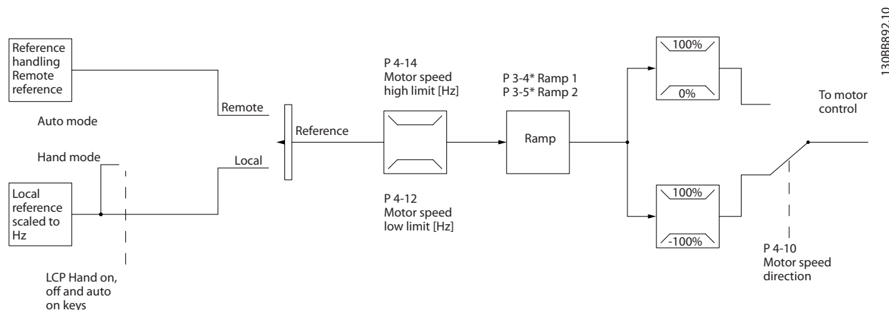
Рисунок 3.17 Структура разомкнутого контура
