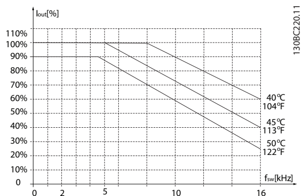
Рисунок 3.25 2,2–4,0 кВт (3,0–5,4 л. с.), 400 В, размер корпуса H2, IP20
