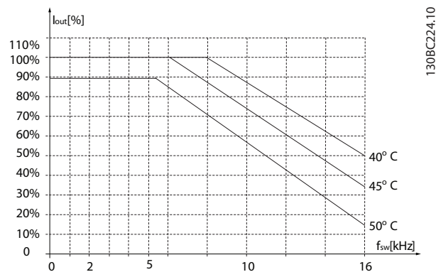
Рисунок 3.29 11–15 кВт (15–20 л. с.), 400 В, размер корпуса H4, IP20
