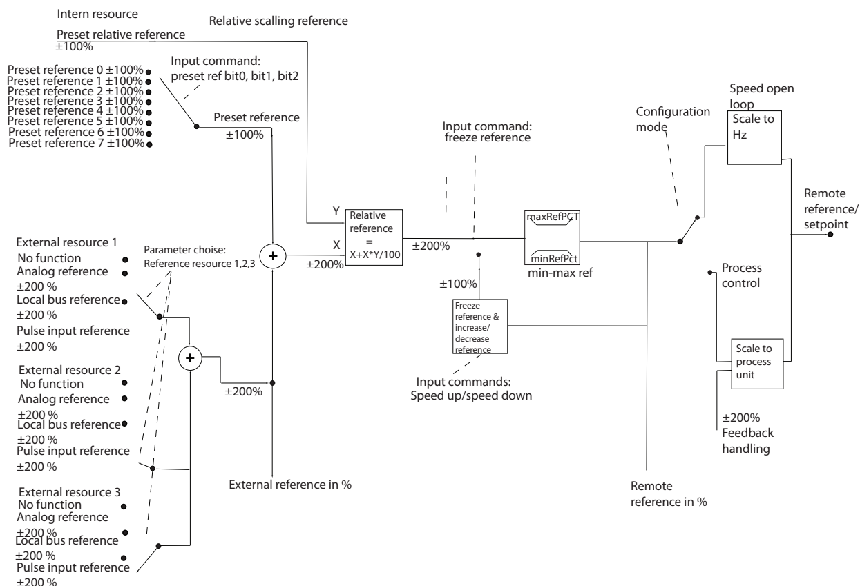
Рисунок 3.21 Блок-схема дистанционного задания
