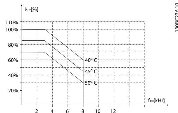
Рисунок 3.41 75–90 кВт (100–120 л. с.), 600 В, размер корпуса H8, IP20
