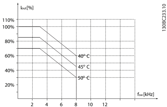
Рисунок 3.38 45–55 кВт (60–74 л. с.), 600 В, размер корпуса H7, IP20
