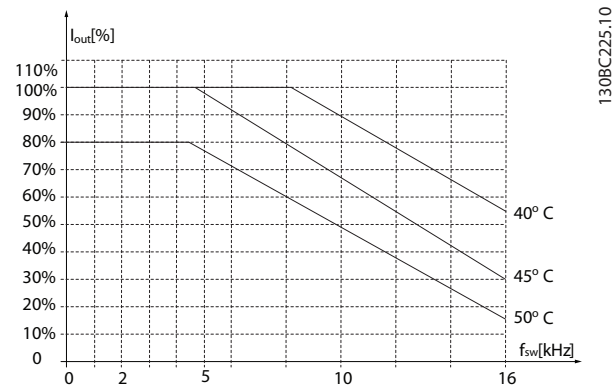
Рисунок 3.30 11 кВт (15 л. с.), 200 В, размер корпуса H5, IP20
