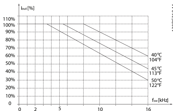
Рисунок 3.23 0,37–1,5 кВт (0,5–2,0 л. с.), 400 В, размер корпуса H1, IP20
