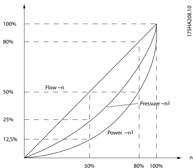
Рисунок 3.3 Законы пропорционального управления
