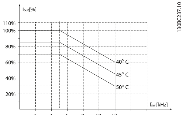
Рисунок 3.42 2,2–3 кВт (3,0–4,0 л. с.), 600 В, размер корпуса H9, IP20
