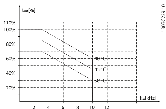
Рисунок 3.44 11–15 кВт (15–20 л. с.), 600 В, размер корпуса H10, IP20
