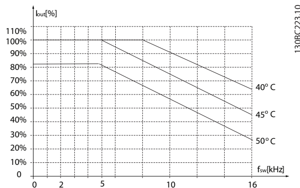
Рисунок 3.28 5,5–7,5 кВт (7,4–10 л. с.), 200 В, размер корпуса H4, IP20
