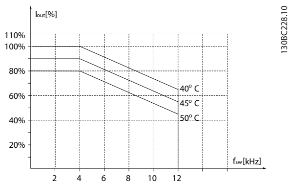
Рисунок 3.33 30–37 кВт (40–50 л. с.), 400 В, размер корпуса H6, IP20
