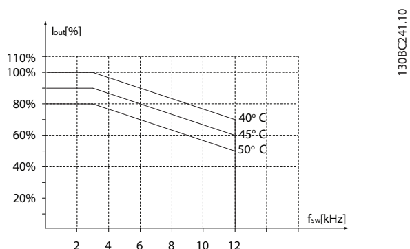
Рисунок 3.49 37 кВт (50 л. с.), 400 В, размер корпуса 16, IP54
