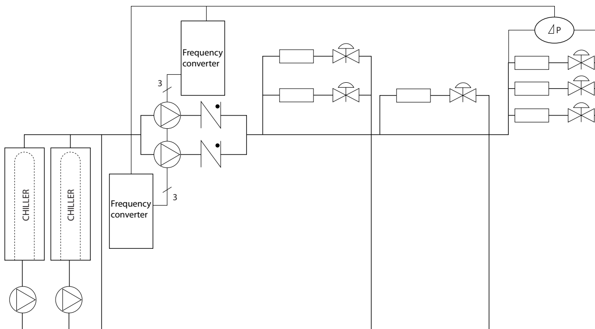
Рисунок 3.16 Вторичные насосы
