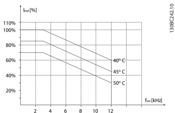
Рисунок 3.50 45–55 кВт (60–74 л. с.), 400 В, размер корпуса 17, IP54
