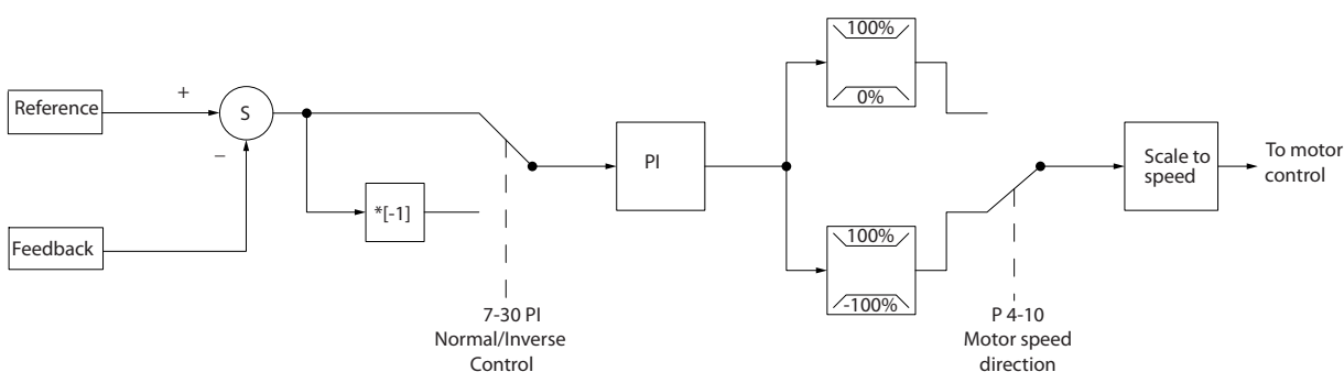
Рисунок 3.19 Замкнутый контур структуры управления
