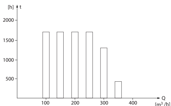
Рисунок 3.6 Распределение расхода в течение 1 года
