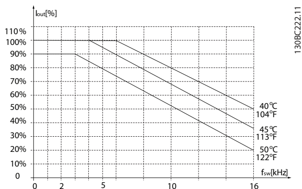
Рисунок 3.27 5,5–7,5 кВт (7,4–10 л. с.), 400 В, размер корпуса H3, IP20
