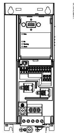
Рисунок 7.2 Заводская установка переключателя
