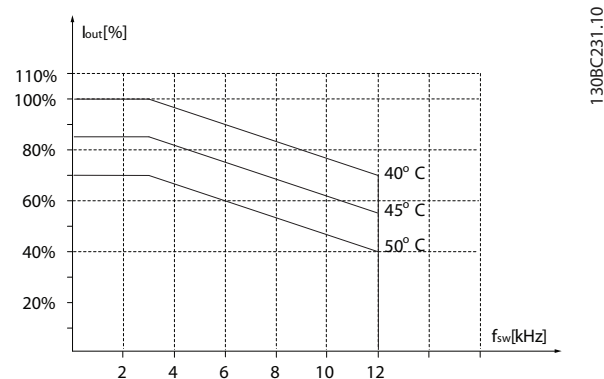
Рисунок 3.36 22–30 кВт (30–40 л. с.), 200 В, размер корпуса H7, IP20
