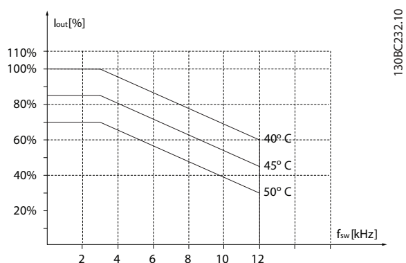
Рисунок 3.37 55–75 кВт (74–100 л. с.), 400 В, размер корпуса H7, IP20
