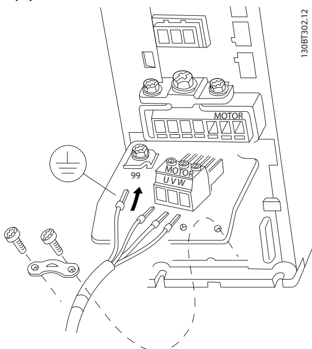
Рисунок 5.6 Подключение двигателя, размер корпуса Н9
