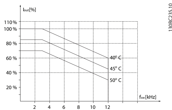
Рисунок 3.40 90 кВт (120 л. с.), 400 В, размер корпуса H8, IP20
