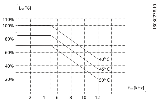
Рисунок 3.43 5,5–7,5 кВт (7,4–10 л. с.), 600 В, размер корпуса Н9, IP20
