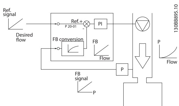
Рисунок 3.20 Преобразование сигнала обратной связи
