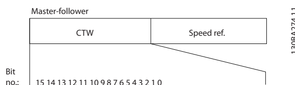
Рисунок 7.15 Командное слово, соответствующее профилю FC
