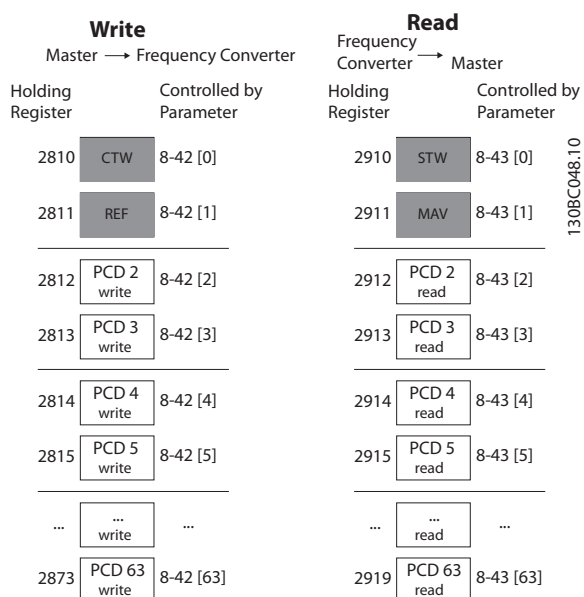
Рисунок 7.14 Доступ посредством чтения/записи PCD
