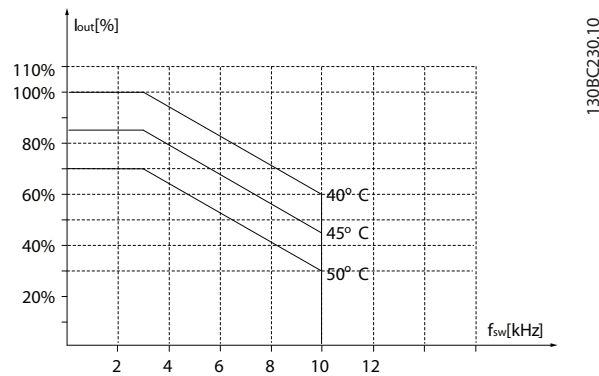
Рисунок 3.35 22–30 кВт (30–40 л. с.), 600 В, размер корпуса H6, IP20
