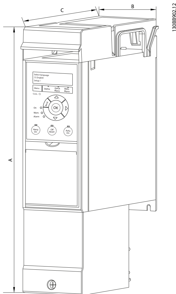
Рисунок 4.6 Н1–Н5 (см. данные в Таблица 4.4)
