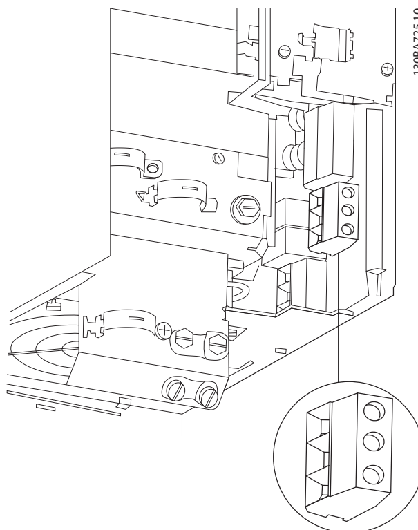
Рисунок 5.7 Размер корпуса Н10
