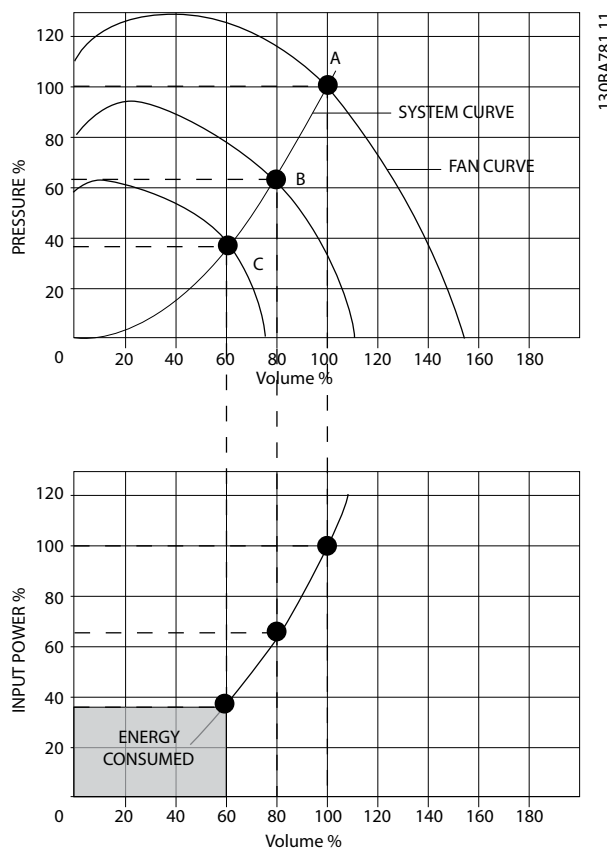
Рисунок 3.2 Экономия энергии благодаря применению решений с преобразователями частоты
