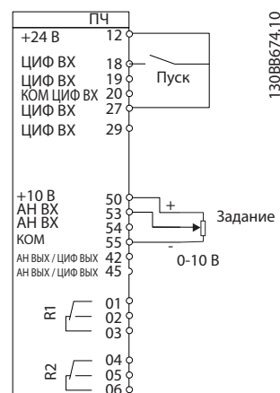
Рисунок 6.2 Проводка преобразователя частоты
