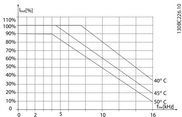
Рисунок 3.31 18,5–22 кВт (25–30 л. с.), 400 В, размер корпуса H5, IP20
