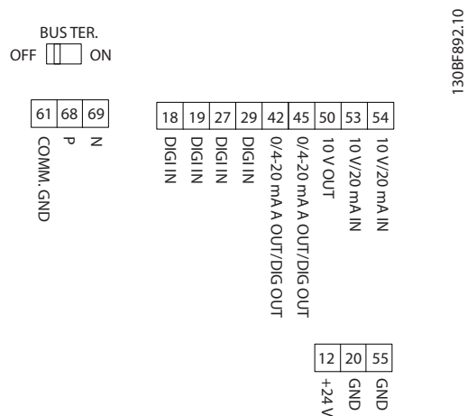
Рисунок 5.17 Клеммы управления
