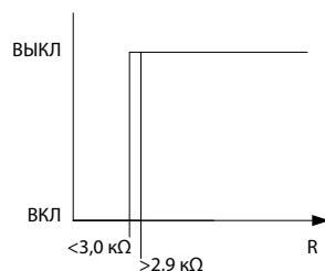
Рисунок 3.59 Аналоговый вход/питание 10 В
