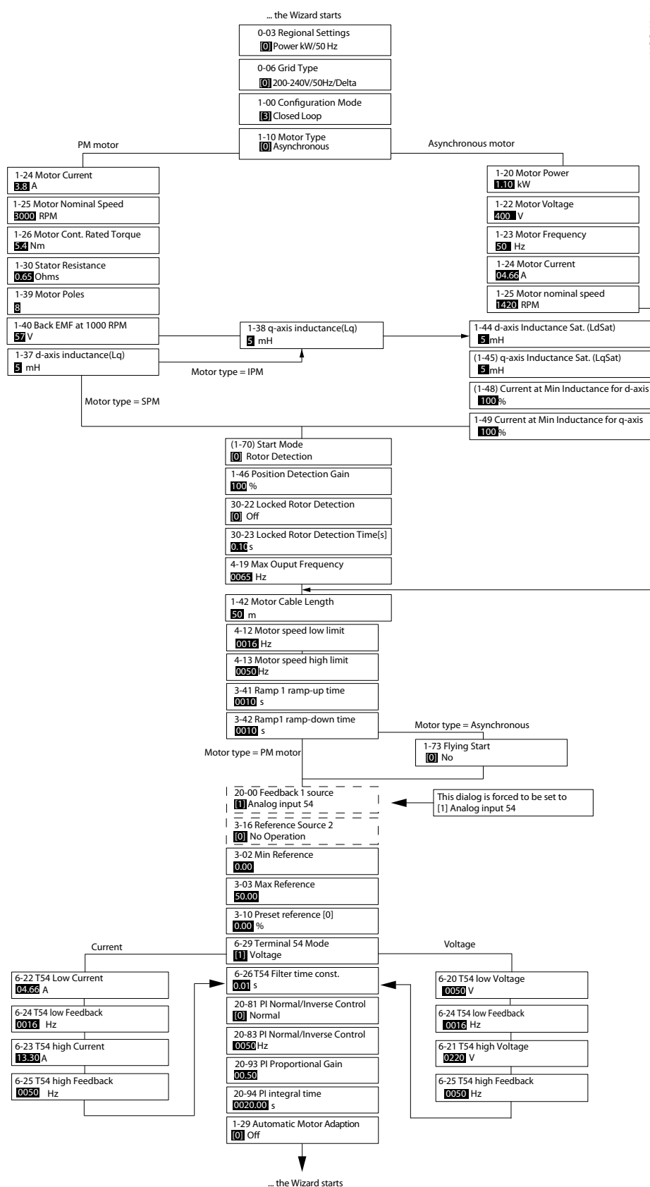
Рисунок 6.5 Мастер настройки параметров применений с замкнутым контуром
