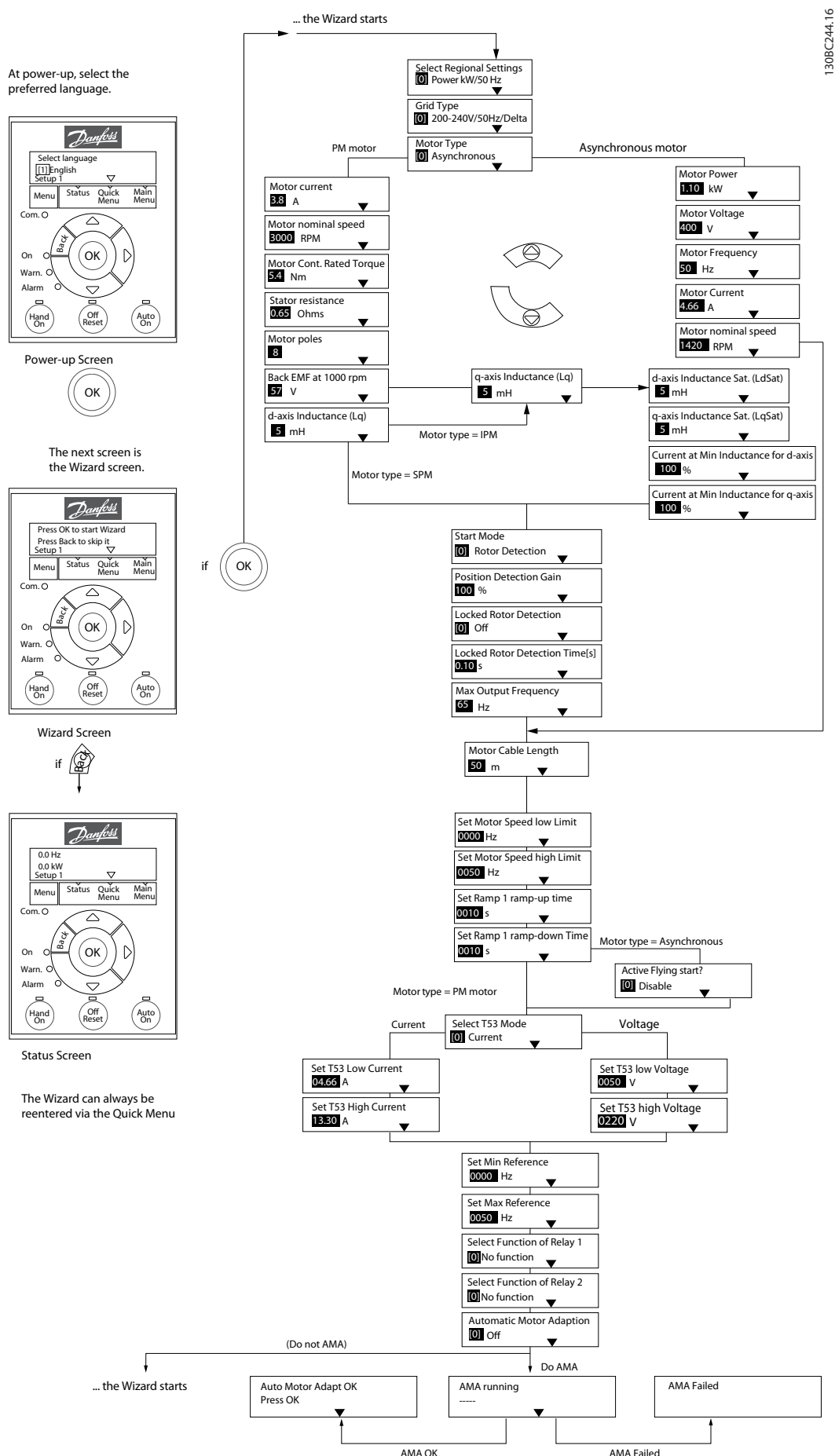
Рисунок 6.4 Мастер настройки параметров применений с разомкнутым контуром
