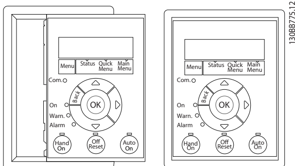
Рисунок 4.2 Установите уплотнитель
