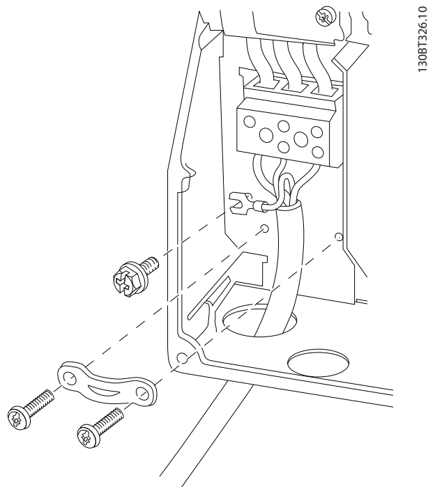
Рисунок 5.12 Подключение сети питания для корпусов I6 IP54, 380–480 В, 22–37 кВт (30–50 л. с.)
