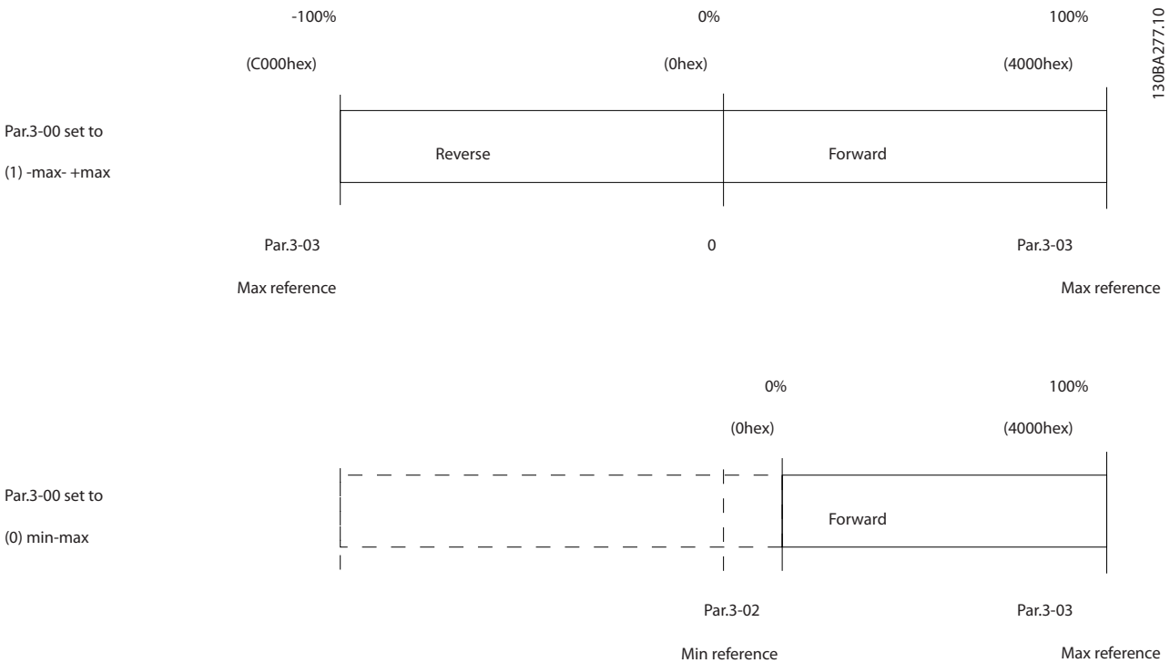
Рисунок 7.18 Задание и MAV
