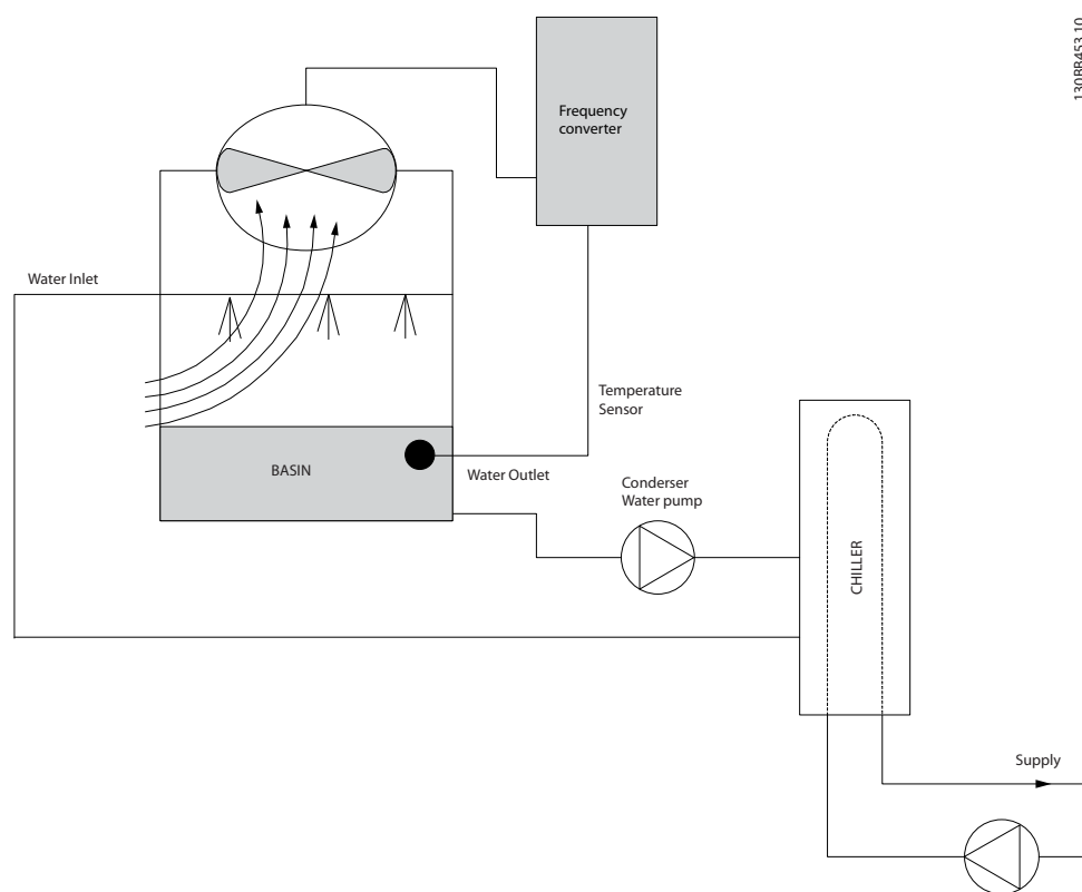
Рисунок 3.13 Вентилятор градирни
