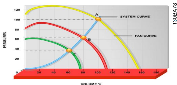
Рисунок 3.1 Кривые вентиляторов (А, В и С) в случае их уменьшенной производительности
