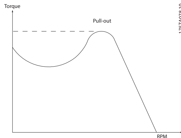
Рисунок 1.1 Момент срыва
