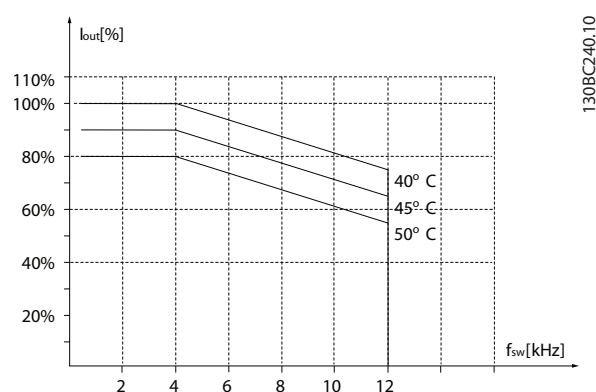
Рисунок 3.48 22–30 кВт (30–40 л. с.), 400 В, размер корпуса I6, IP54
