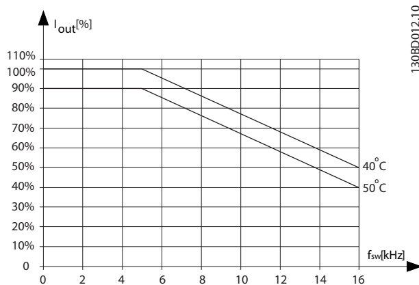
Рисунок 3.47 11–18,5 кВт (15–25 л. с.), 400 В, размер корпуса I4, IP54
