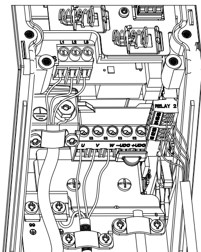
Рисунок 5.11 IP54, размеры корпуса I2, I3, I4
