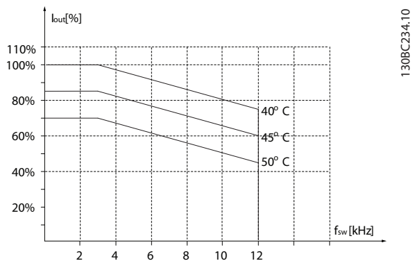
Рисунок 3.39 37–45 кВт (50–60 л. с.), 200 В, размер корпуса H8, IP20
