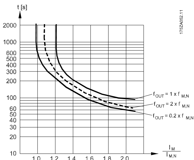
Рисунок 3.56 Характеристики тепловой защиты двигателя
