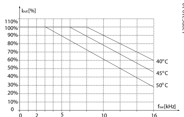
Рисунок 3.24 2,2 кВт (3,0 л. с.), 200 В, размер корпуса H2, IP20
