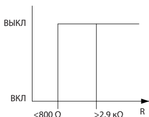
Рисунок 3.58 Цифровой вход/питание 10 В
