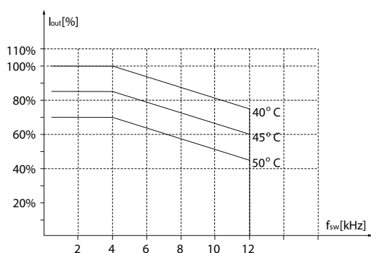
Рисунок 3.32 15–18,5 кВт (20–25 л. с.), 200 В, размер корпуса H6, IP20
