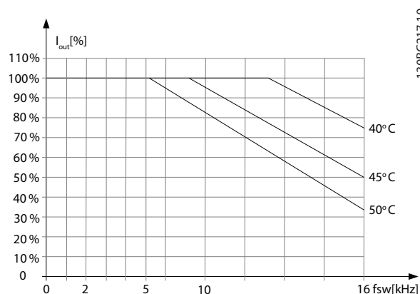
Рисунок 3.22 0,25–0,75 кВт (0,34–1,0 л. с.), 200 В, размер корпуса H1, IP20
