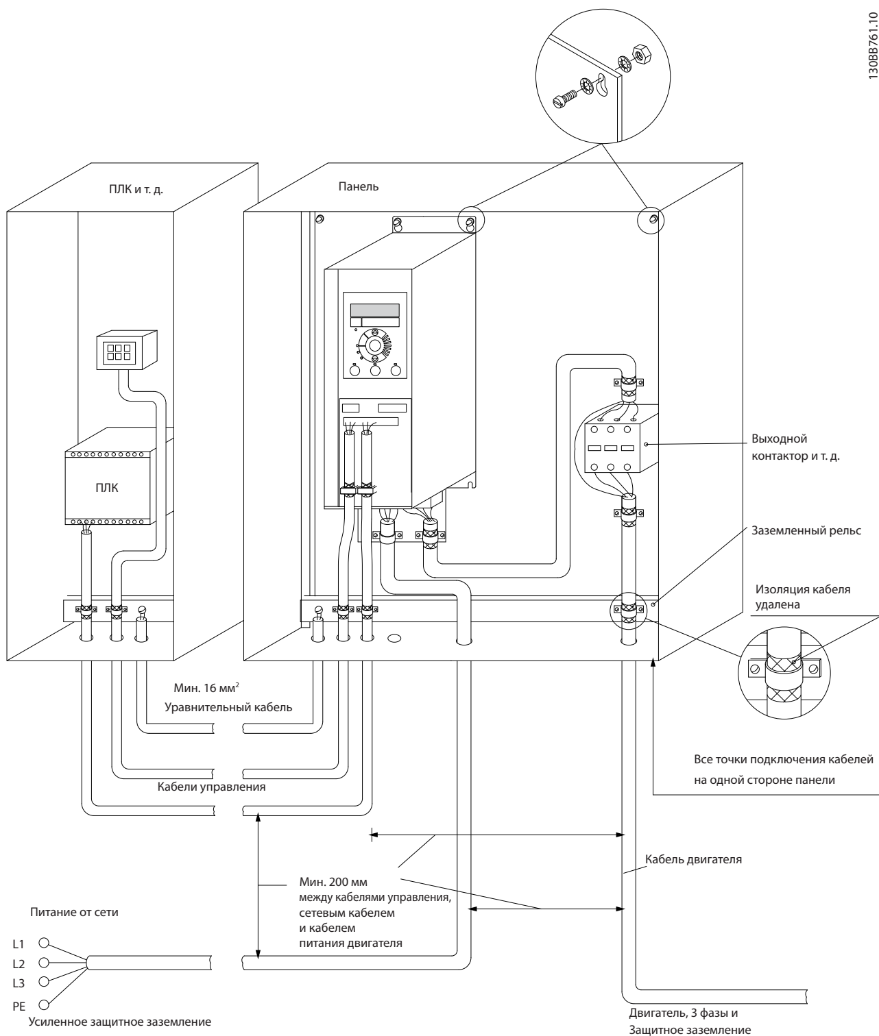
Рисунок 5.16 Электрический монтаж с учетом требований ЭМС
