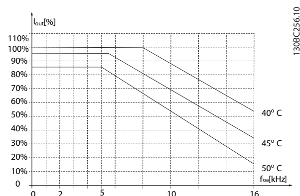
Рисунок 3.46 5,5–7,5 кВт (7,4–10 л. с.), 400 В, размер корпуса I3, IP54
