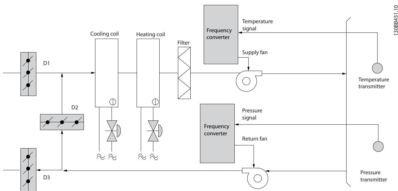
Рисунок 3.12 Постоянный объем воздуха
