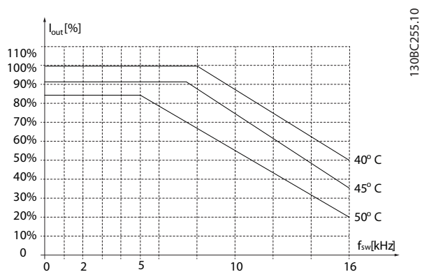
Рисунок 3.45 0,75–4,0 кВт (1,0–5,4 л. с.), 400 В, размер корпуса I2, IP54
