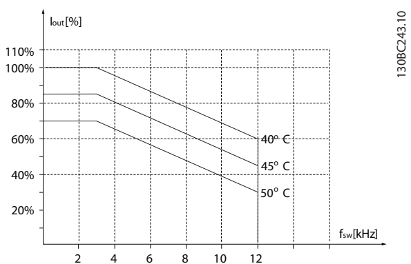
Рисунок 3.51 75–90 кВт (100–120 л. с.), 400 В, размер корпуса 18, IP54
