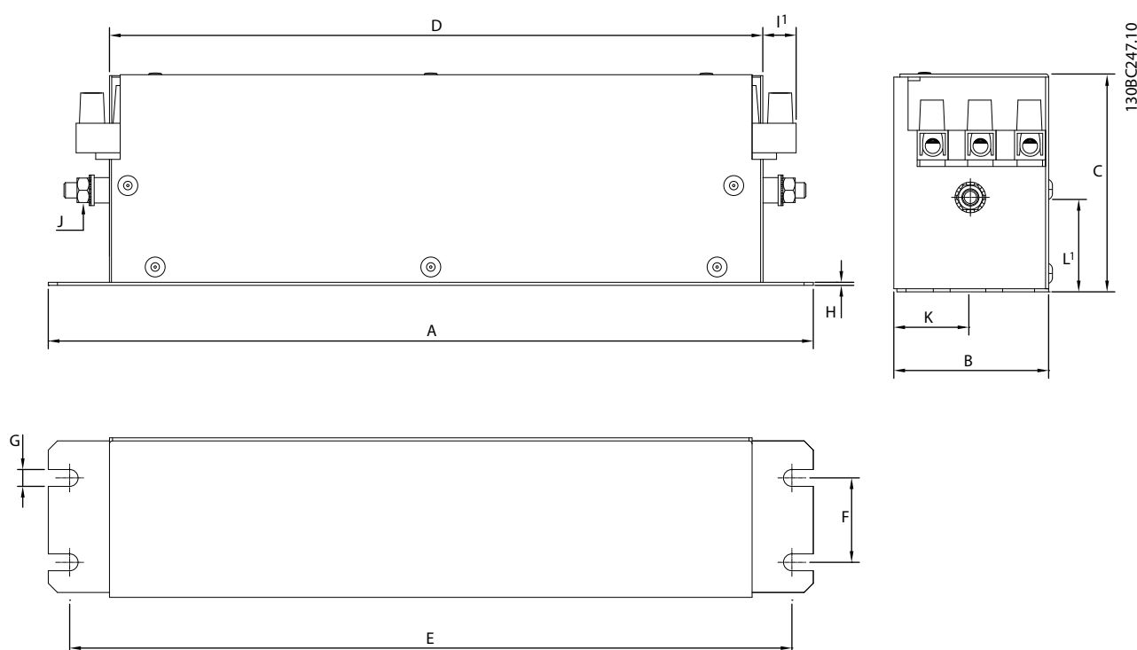
Рисунок 4.9 Фильтр ВЧ-помех - габаритные размеры
