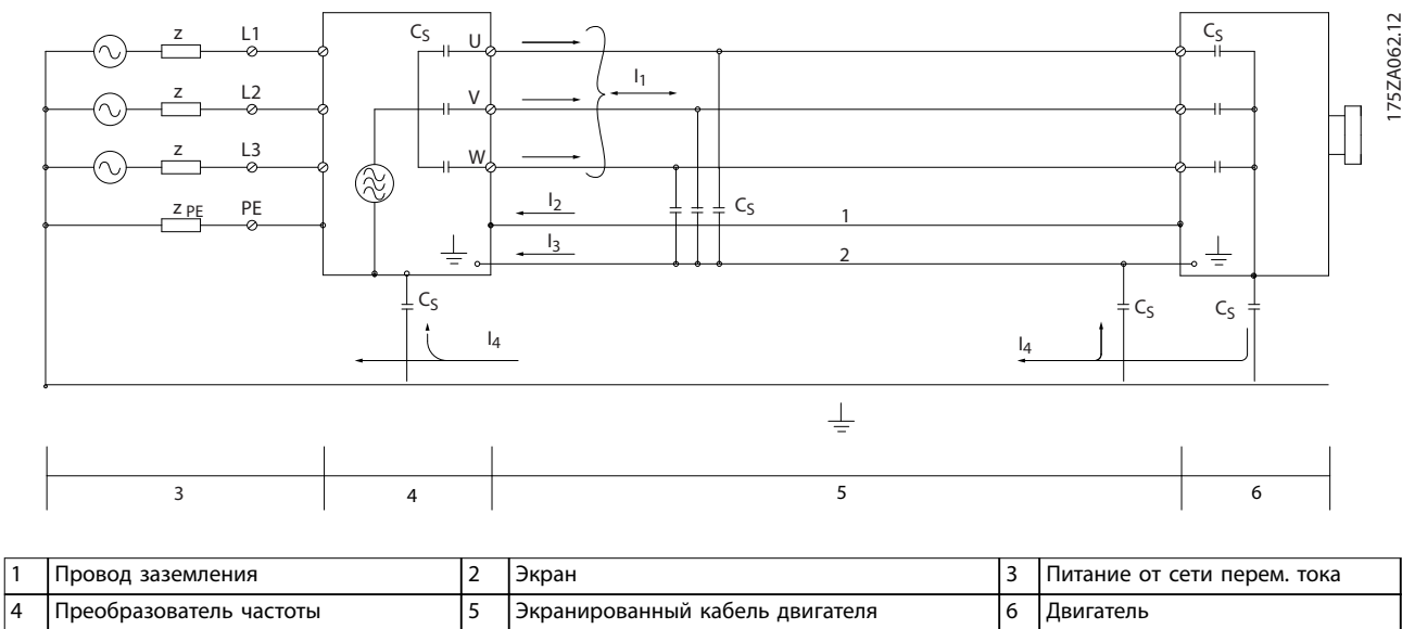
Рисунок 3.52 Генерирование токов утечки
