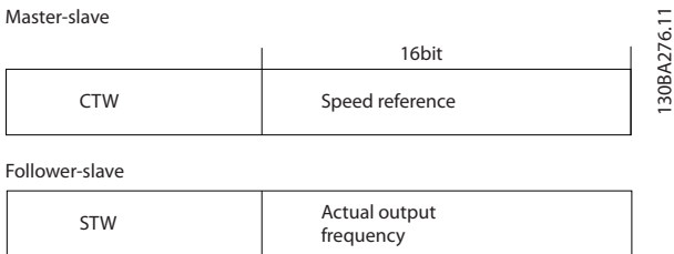
Рисунок 7.17 Текущая выходная частота (MAV)
