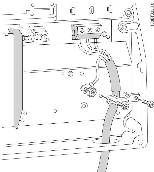
Рисунок 5.13 Подключение двигателя для корпуса I6 IP54, 380–480 В, 22–37 кВт (30–50 л. с.)
