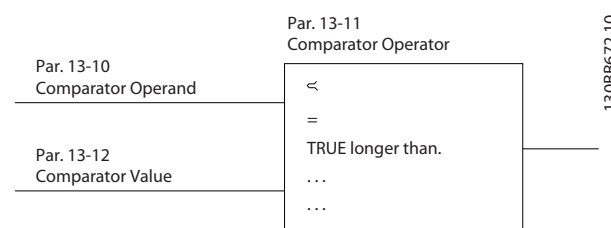
Рисунок 3.14 Компараторы
