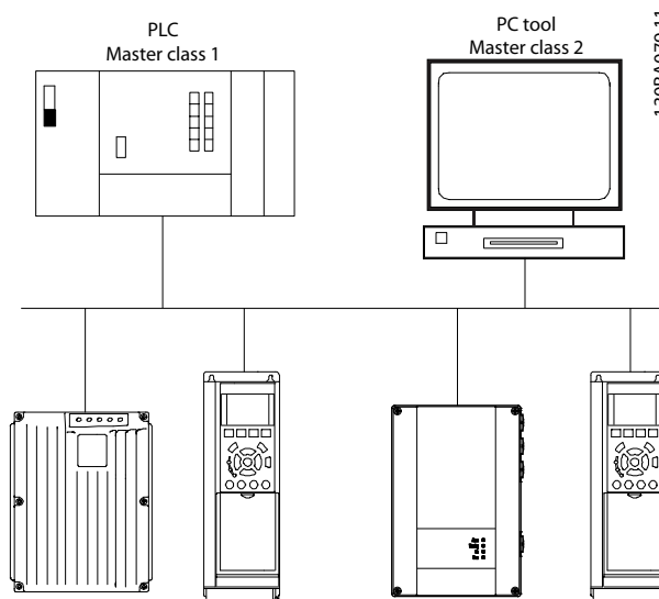
Рисунок 1.2 PROFIBUS DP-V1
