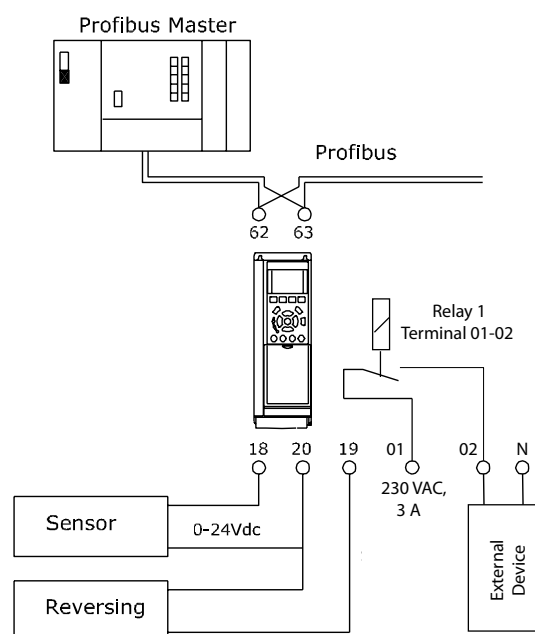
Рисунок 7.1 Схема соединений
