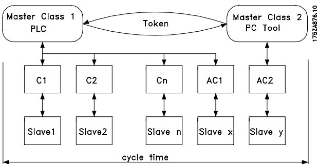
Рисунок 5.1 Цикл DP
