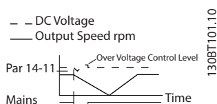
Рисунок 3.34 Управляемое замедление — короткое замыкание сети. После замедления и остановки следует разгон до заданного значения.
