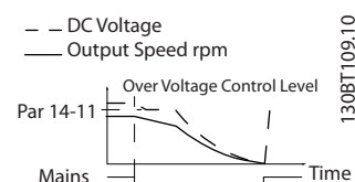
Рисунок 3.37 Кинетический резерв, более длительное замыкание сети. Двигатель останавливается выбегом, как только энергия в системе падает слишком низко.
