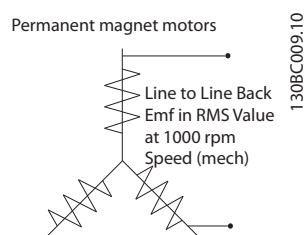
Рисунок 3.7 Определения параметров аппарата противоэдс двигателей с постоянными магнитами
