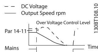
Рисунок 3.35 Управляемое замедление, более длительное размыкание цепи. Замедление длится до тех пор, пока в системе остается энергия, после этого двигатель останавливается выбегом.
