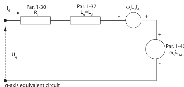
Рисунок 3.5 Эквивалентная схема двигателя для неявнополюсного двигателя с постоянными магнитами (PM)
