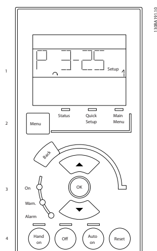
Рисунок 2.10 Цифровая панель местного управления (NLCP)
