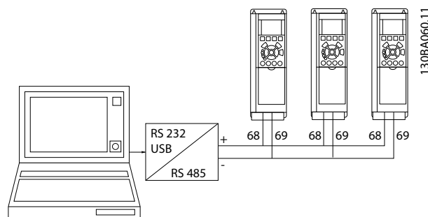
Рисунок 8.1 Параллельные соединения
