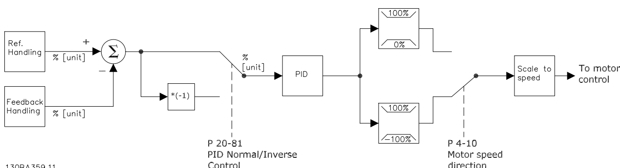
Рисунок 2.26 Блок-схема регулятора с замкнутым контуром
