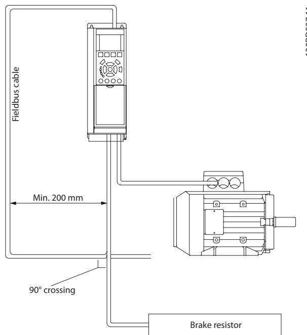
Рисунок 8.4 Прокладка кабелей
