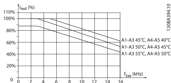
Рисунок 9.5 Снижение номинального тока I_{\text{вых.}} при различных значениях T_{\text{окр. ср., макс.}} для корпуса типа A, модели коммутации 60° AVM, при использовании кабеля двигателя длиной не более 10 м
