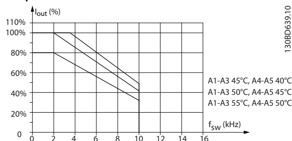
Рисунок 9.4 Снижение номинального тока I_{\text{вых.}} при различных значениях T_{\text{окр. ср., макс.}} для корпусов типа A и модели коммутации SFAVM
