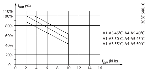
Рисунок 9.6 Снижение номинального тока I_{\text{вых.}} при различных значениях T_{\text{окр. ср., макс.}} для корпусов типа A, модели коммутации SFAVM, при использовании кабеля двигателя длиной не более 10 м
