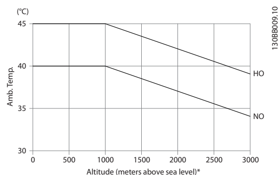
Рисунок 9.26 Пример: При высоте 2000 м и температуре 45 °C ( T_{окр.ср., макс.} - 3,3 K) доступное значение выходного тока составляет 91 % от номинального значения. При температуре 41,7 °C доступное значение выходного тока составляет 100 % от номинального.
