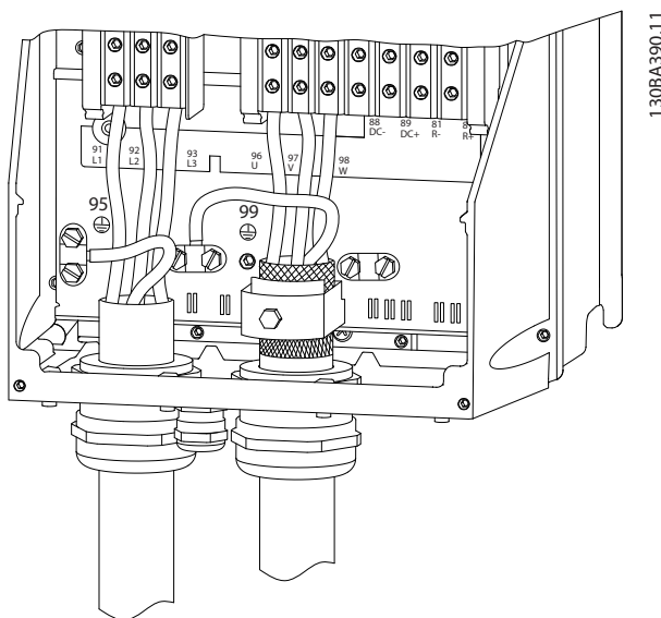
Рисунок 4.8 Проводка двигателя, питания и заземления для типов корпуса B и C с использованием экранированных кабелей
