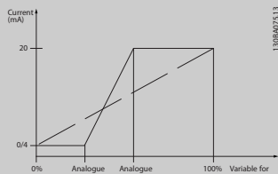
Рисунок 6.13 Зависимость выходного тока от переменной-задания
