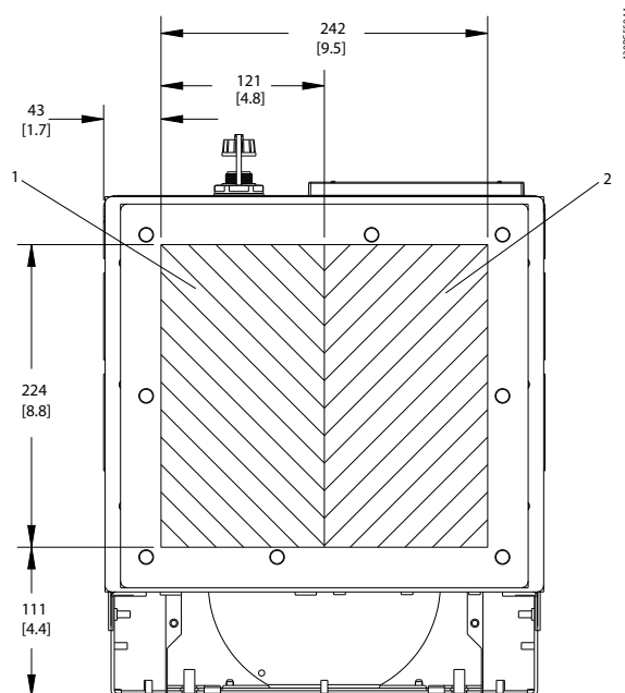
Рисунок 6.82 D5h и D6h, вид снизу
