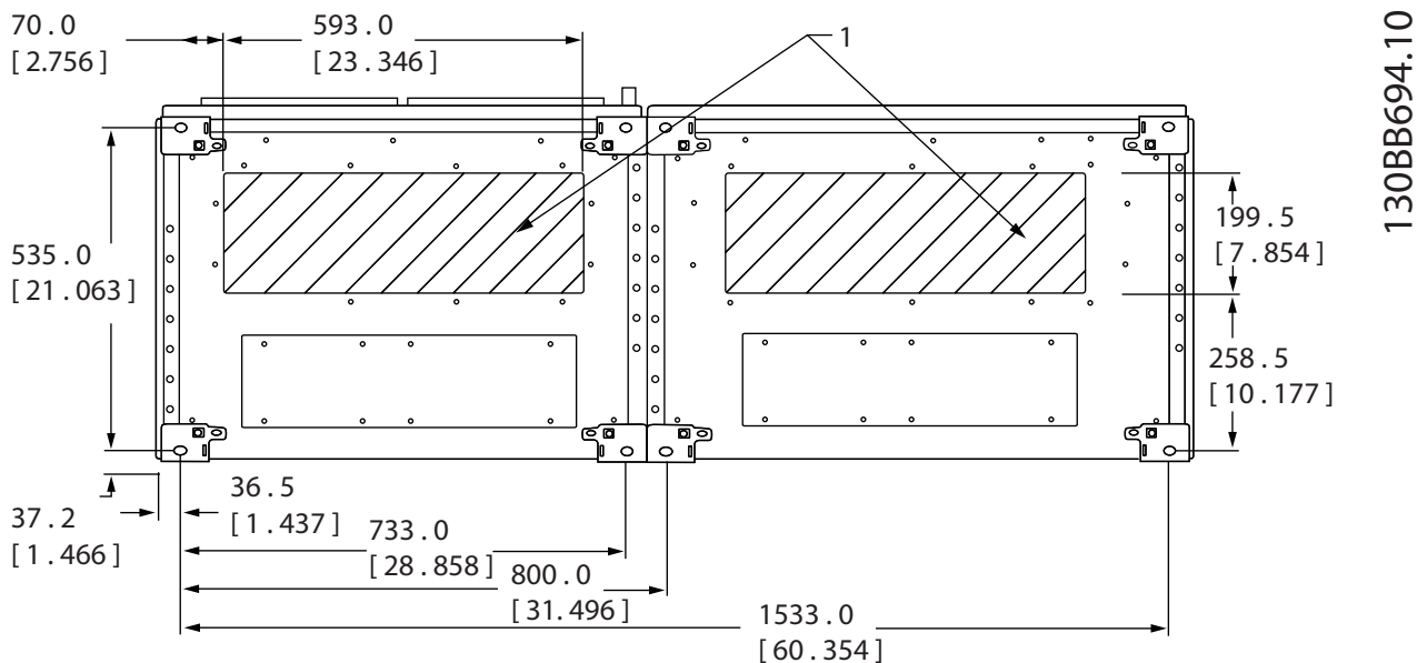
Рисунок 6.91 Типоразмер F10
