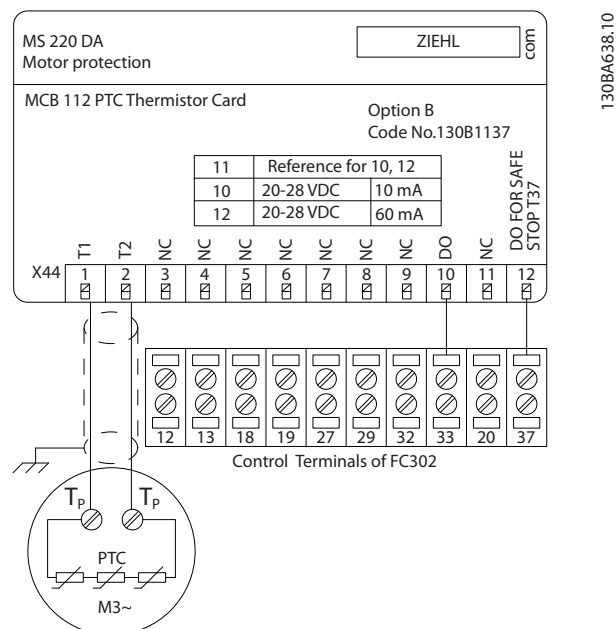
Рисунок 9.15 Монтаж MCB 112
