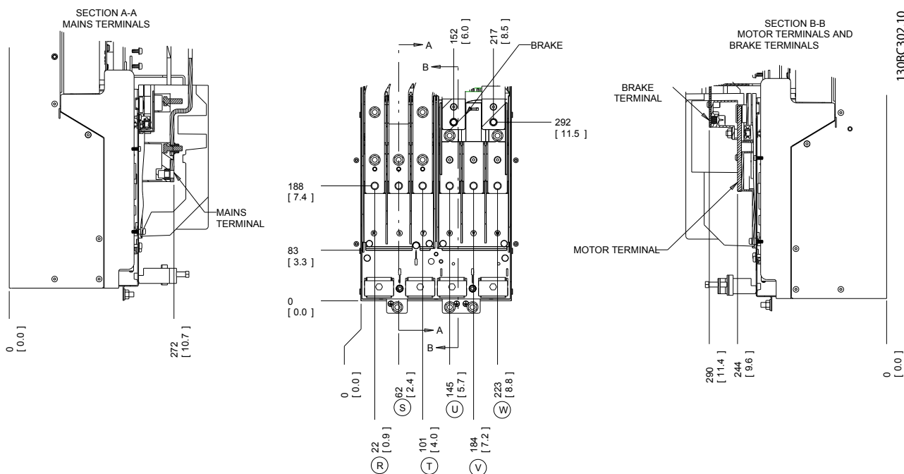
Рисунок 6.47 Расположение силовых разъемов, типоразмер D3h
