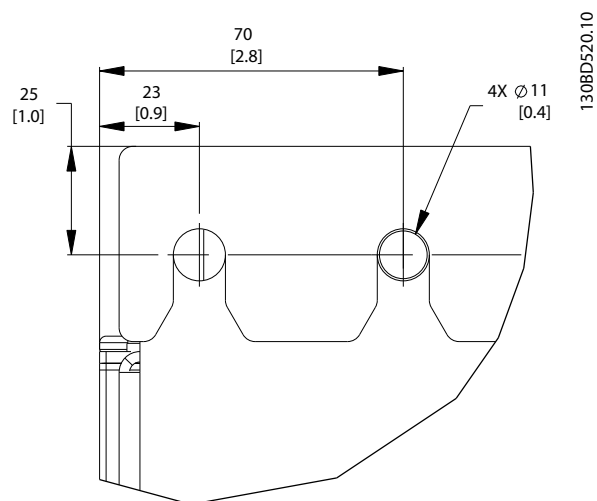
Рисунок 6.20 Детальный чертеж верхнего монтажного отверстия, D7h
