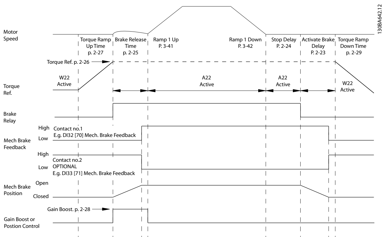
Рисунок 3.34 Последовательность отпущения тормоза при управлении механическим тормозом подъемного механизма
