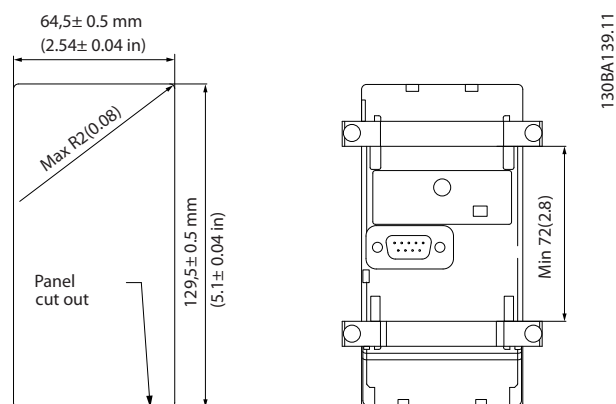
Рисунок 9.18 Размеры
