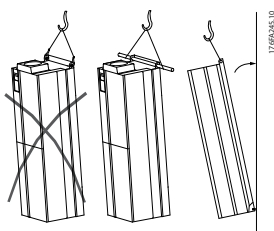
Рисунок 6.3 Рекомендуемый метод подъема, типоразмер E
