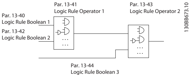
Рисунок 3.38 Правила логики
