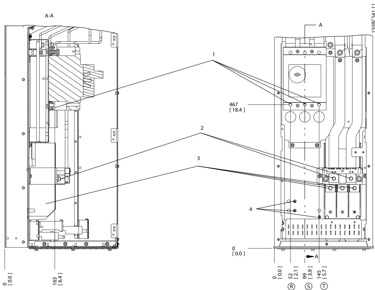
Рисунок 7.11 Расположение клемм, D6h с автоматическим выключателем
