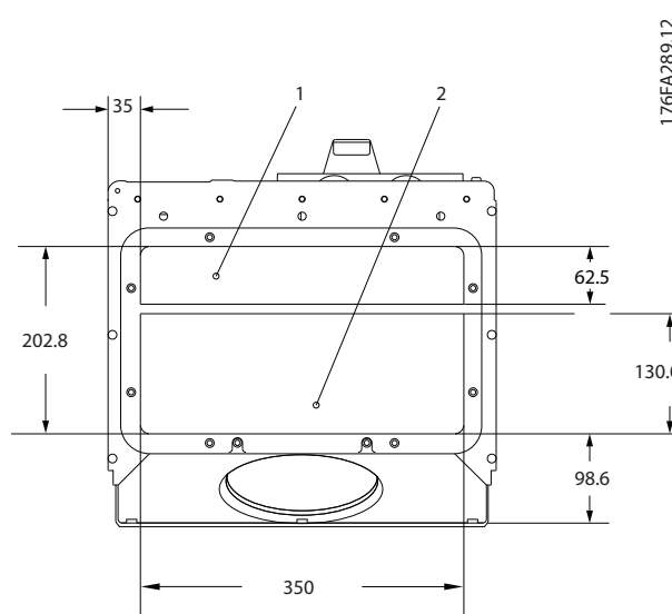
Рисунок 6.84 E1, вид снизу
