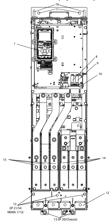
Рисунок 7.3 Внутренние компоненты корпуса типоразмера D
