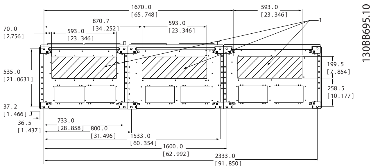
Рисунок 6.92 Типоразмер F11
