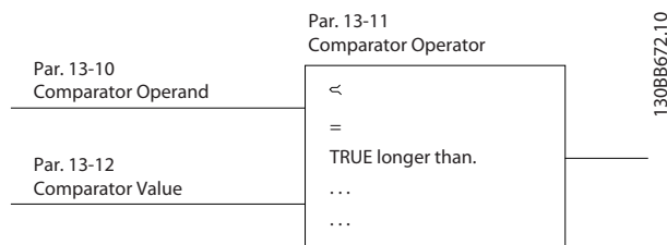
Рисунок 3.37 Компараторы
