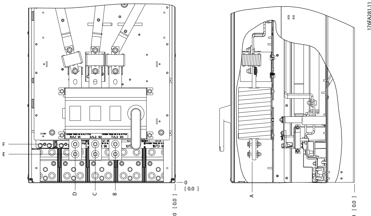
Рисунок 7.22 Подключение электропитания для корпусов IP00, расположение разъединителя
