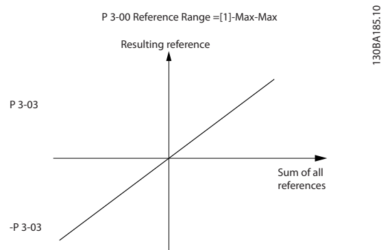
Рисунок 3.12 Результирующее задание
