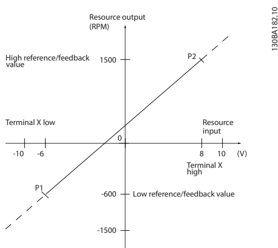
Рисунок 3.15 Масштабирование сигналов обратной связи на аналоговом и импульсном входах
