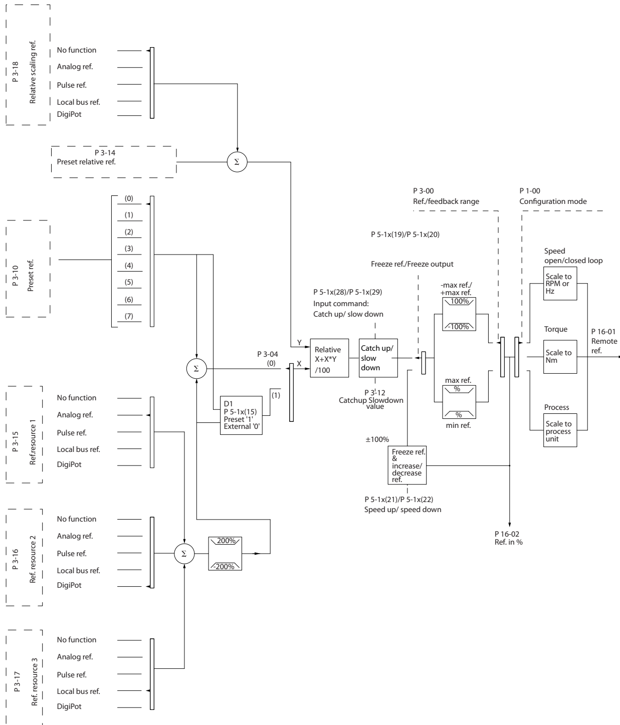
Рисунок 3.10 Дистанционное задание
