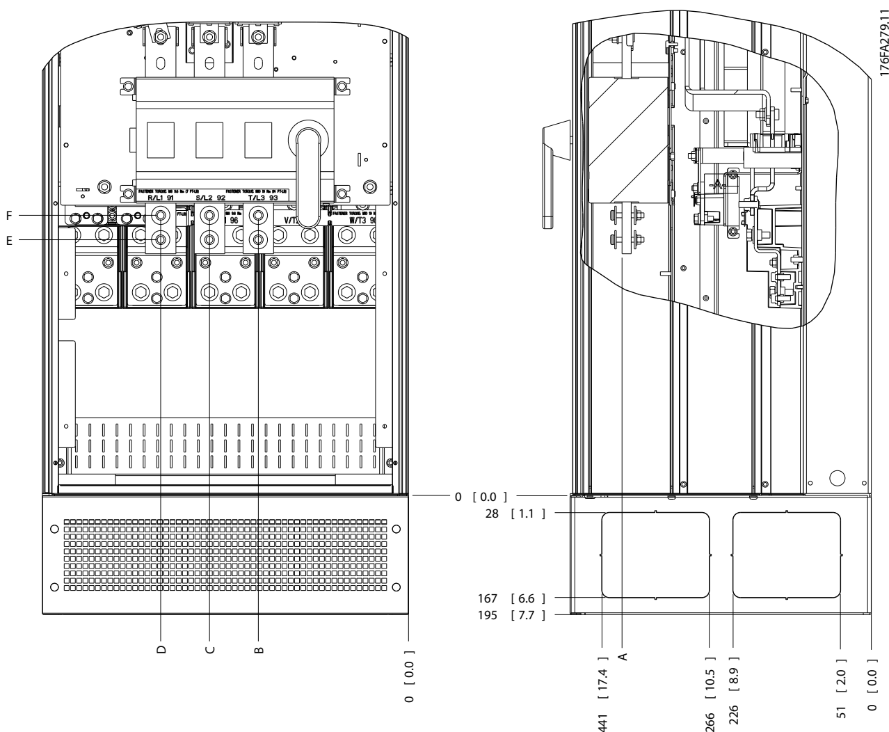
Рисунок 7.19 Расположение расцепителя питания для корпусов IP21 (NEMA тип 1) и IP54 (NEMA тип 12)
