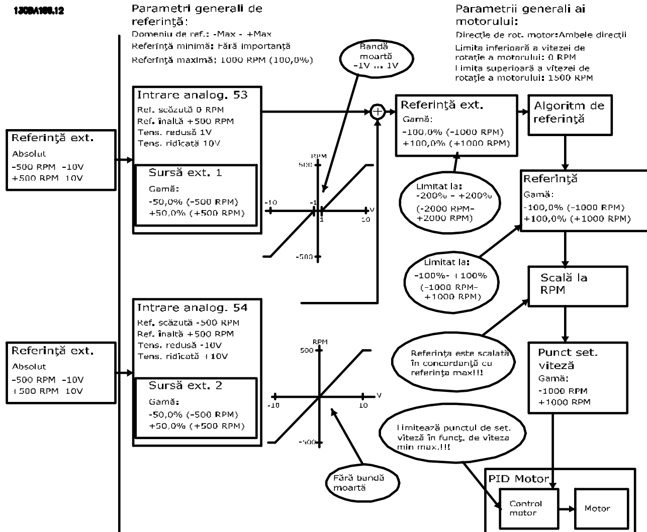
Рисунок 3.20 Задание в диапазоне от отрицательного до положительного значения с зоной нечувствительности, знак определяет направление, от -Макс. до +Макс.
