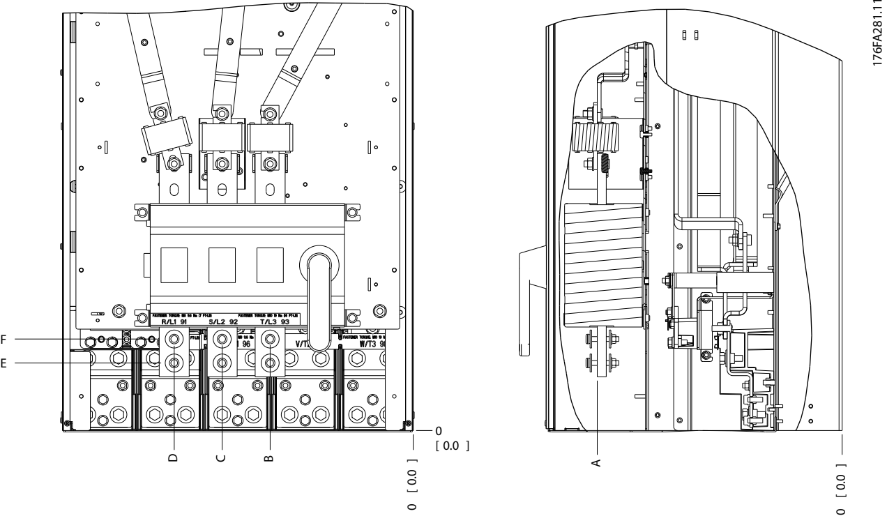
Рисунок 6.66 Расположение разъемов питания на корпусе IP00, расположение распрепителя
