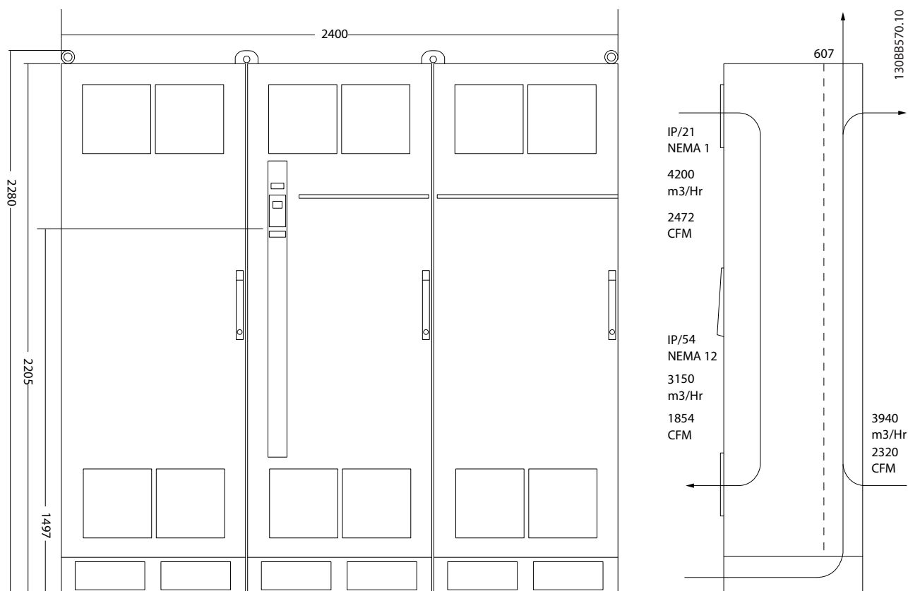
Рисунок 6.30 Габаритные размеры (мм), F11
