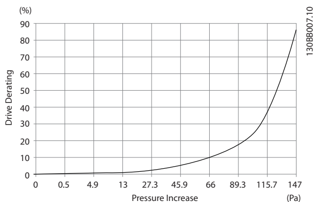
Рисунок 6.95 Снижение номинальных характеристик для корпусов типоразмера D в зависимости от изменения давления. Поток воздуха в преобразователе частоты: 450 куб. футов/мин (765 м³/ч)
