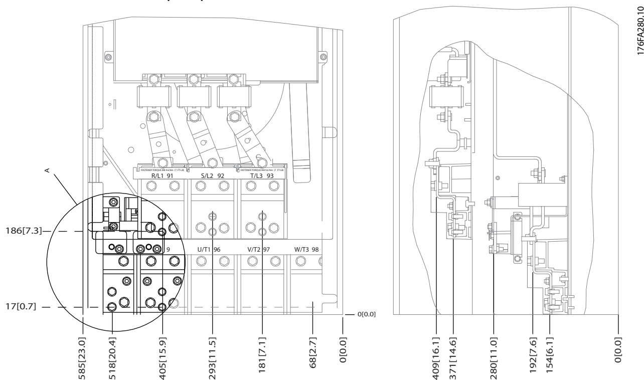
Рисунок 7.20 Расположение клемм электропитания корпусов IP00
