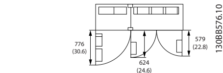
Рисунок 6.44 Пространство перед корпусом типа IP21/IP54, типоразмер F12
