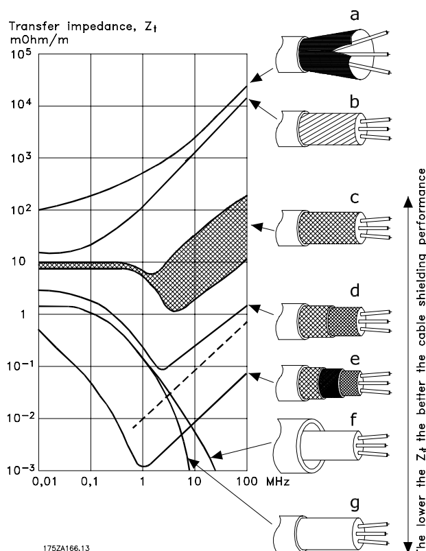
Рисунок 7.58 Передаточный импеданс Z T
