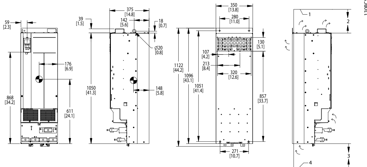
Рисунок 6.13 Габаритные размеры, D4h
