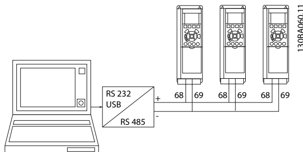
Рисунок 10.1 Параллельные подключения
