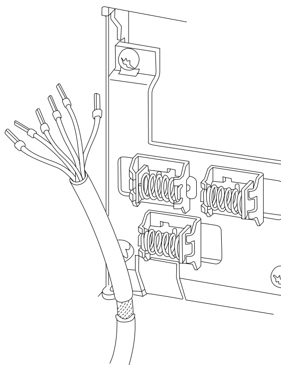
Рисунок 7.47 Заделка экрана и разгрузка натяжения кабеля управления
