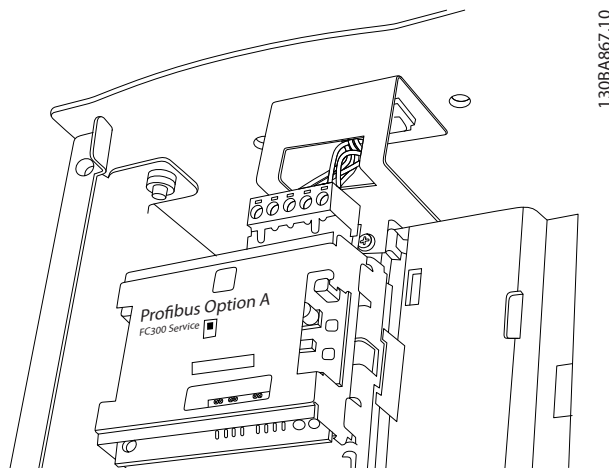
Рисунок 7.37 Подключение периферийной шины сверху
