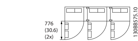
Рисунок 6.43 Пространство перед корпусом типа IP21/IP54, типоразмер F11
