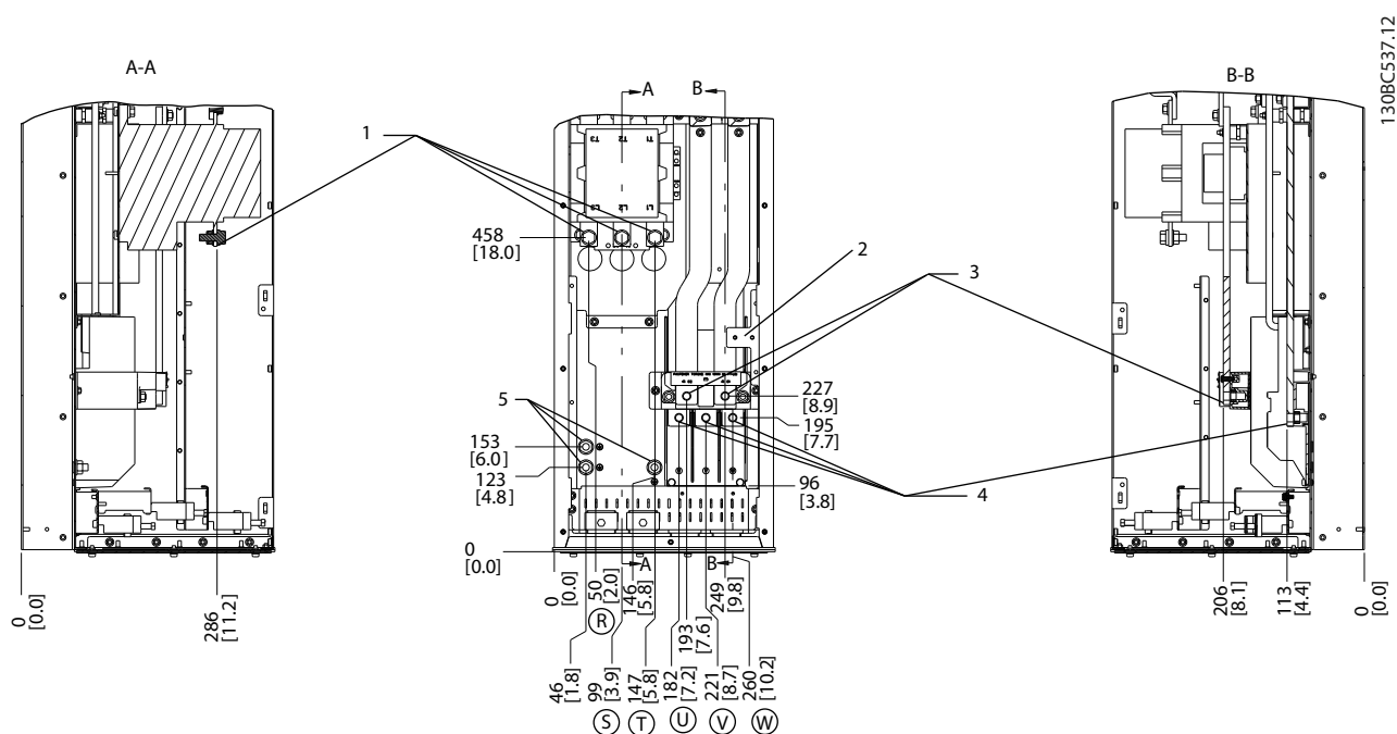
Рисунок 6.52 Расположение клемм, D6h с контактором
