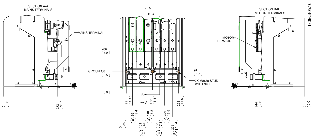
Рисунок 6.46 Расположение силовых разъемов, типоразмер D1h
