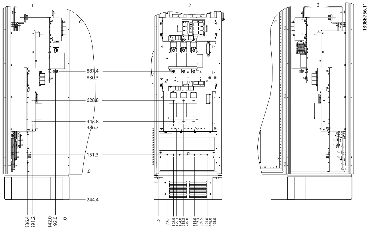
Рисунок 6.78 Расположение клемм — шкаф дополнительных устройств.
