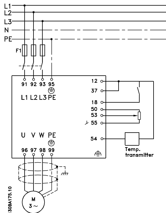
Рисунок 3.24 Двухпроводный датчик
