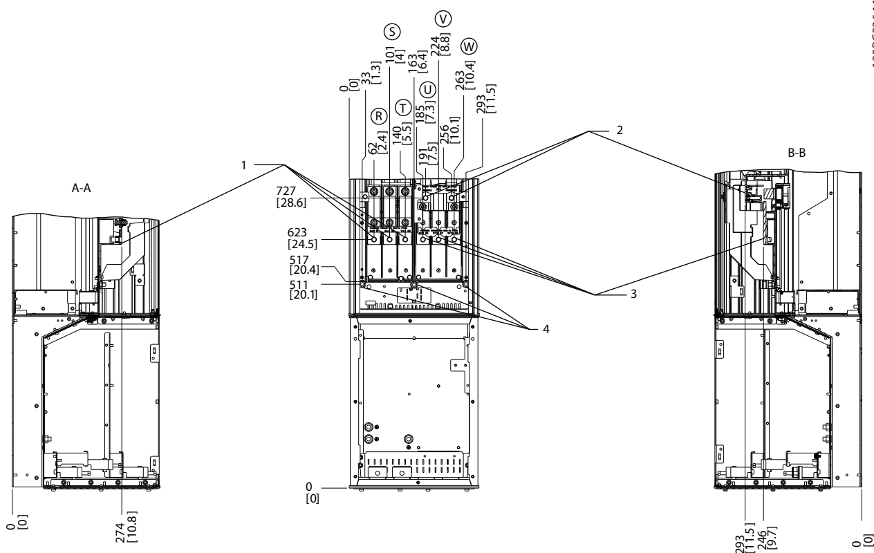
Рисунок 6.51 Расположение клемм, D5h с тормозом
