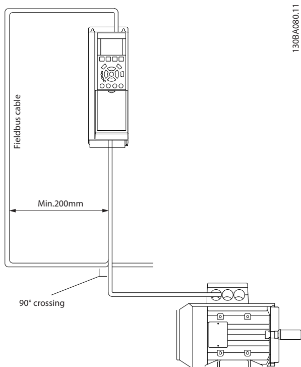
Рисунок 10.3 Обеспечение ЭМС
