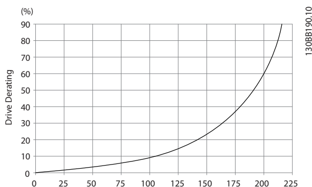
Рисунок 6.98 Снижение номинальных характеристик для корпусов типоразмеров F1, F2, F3, F4 в зависимости от изменения давления. Поток воздуха в преобразователе частоты: 580 куб. футов/мин (985 м³/ч)
