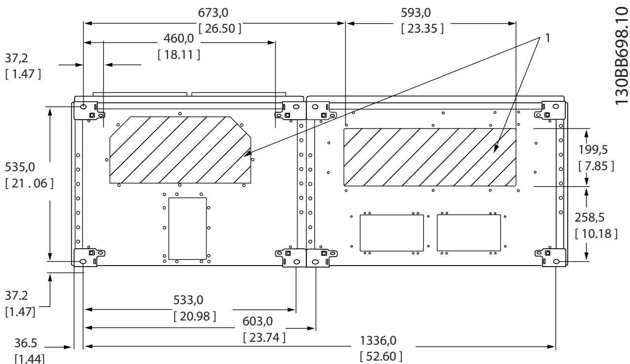
Рисунок 6.90 Типоразмер F9
