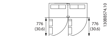
Рисунок 6.42 Пространство перед корпусом типа IP21/IP54, типоразмер F10
