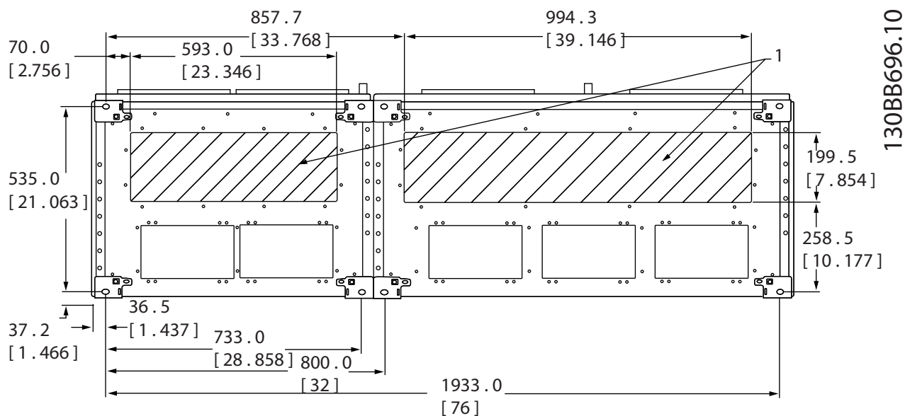
Рисунок 6.93 Типоразмер F12
