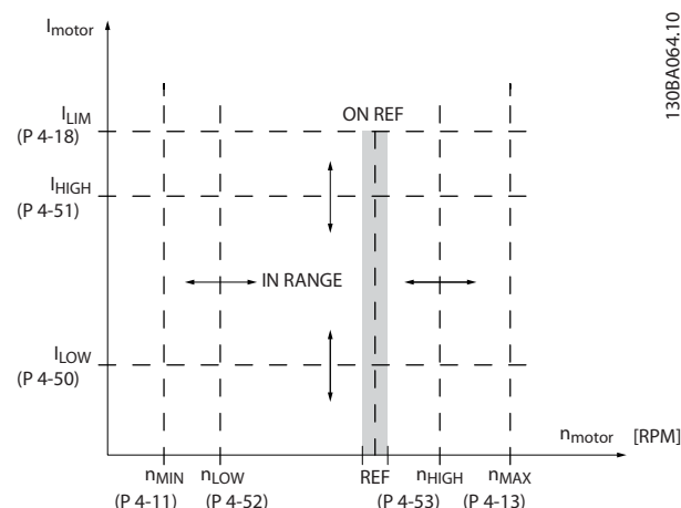
Рисунок 3.35 Настр. предупр.
