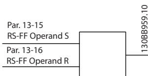
Рисунок 3.55 Триггеры сброса/установки
