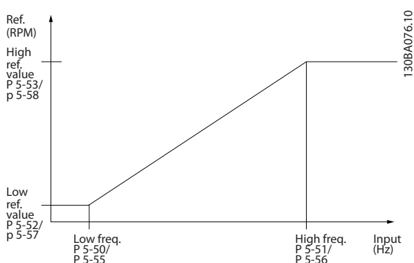
Рисунок 3.40 Импульсный вход
