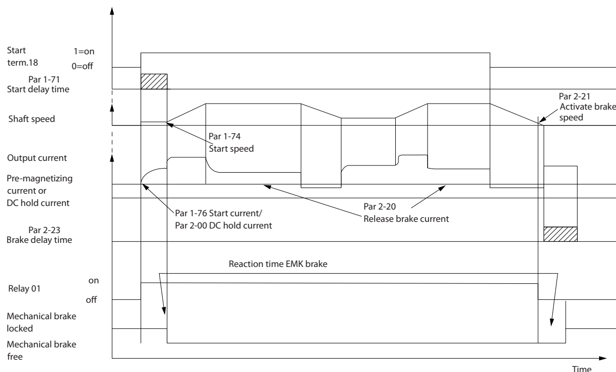
Рисунок 3.21 Механическое торможение
