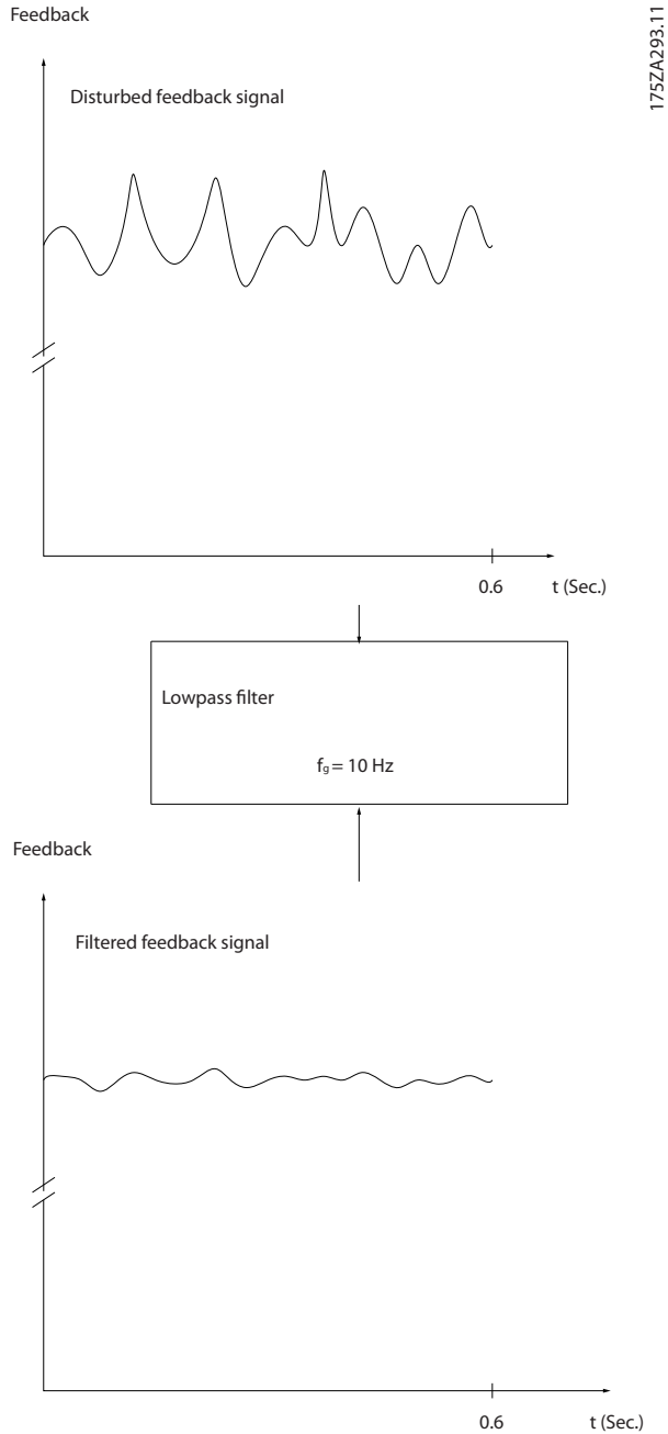
Рисунок 3.49 Сигнал обратной связи
