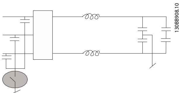
Рисунок 3.64 Фильтр ВЧ-помех
