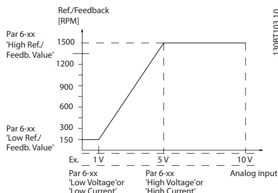
Рисунок 3.44 Аналоговый вход 1
