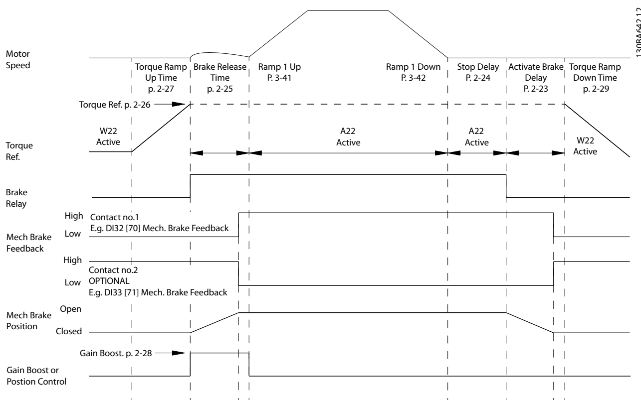
Рисунок 3.22 Последовательность отпускания тормоза при управлении механическим тормозом подъемного механизма Этот способ управления тормозом доступен только при регулировании магнитного потока с обратной связью двигателя или в режиме без использования датчиков и доступен при работе с асинхронными двигателями и неавнополюсными двигателями с постоянными магнитами.
