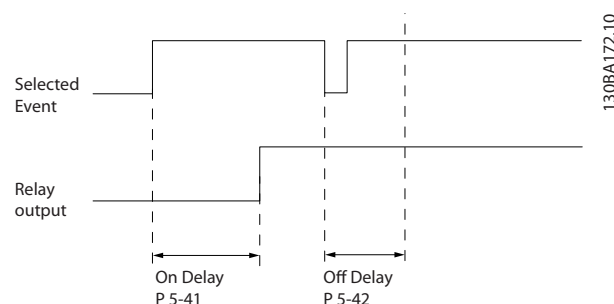
Рисунок 3.39 Задержка выключения, реле
