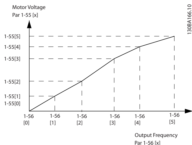
Рисунок 3.12 Характеристика U/f
