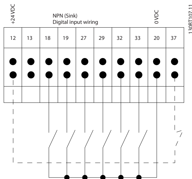
Рисунок 1.4 NPN (сток)
