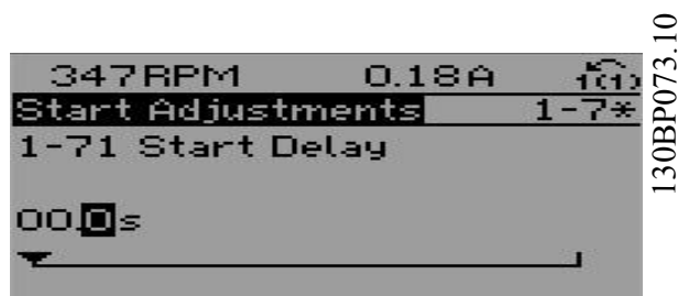
Рисунок 2.19 Выбор цифры
