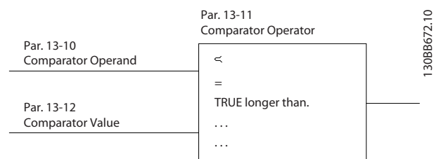
Рисунок 3.54 Компараторы
