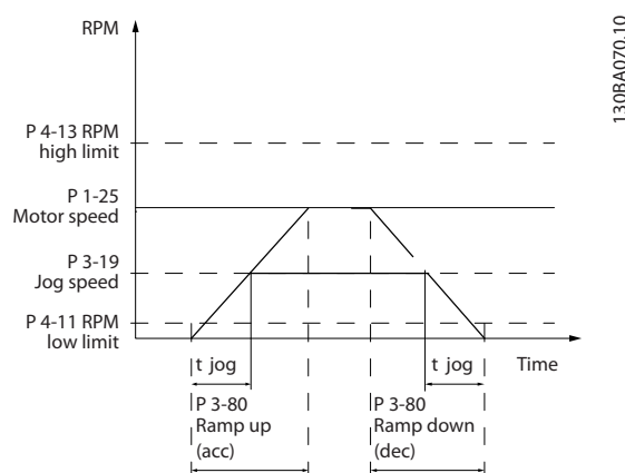
Рисунок 3.29 Темп изм. скор.при перех. на фикс. скор.
