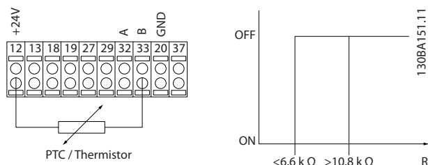
Рисунок 3.19 Подключение термистора
