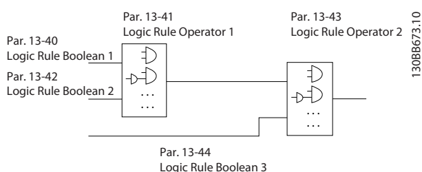
Рисунок 3.57 Логические соотношения
