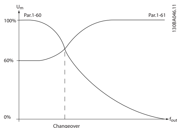
Рисунок 3.13 Переключение нагрузки
