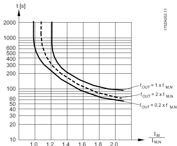
Рисунок 3.18 Профиль ЭТР
