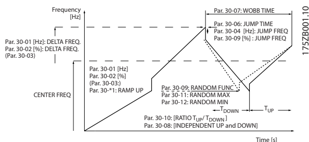
Рисунок 3.68 Генератор колебаний
