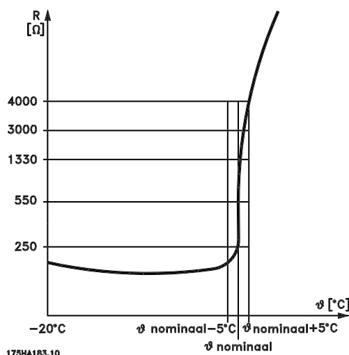
Рисунок 3.14 Профиль РТС
