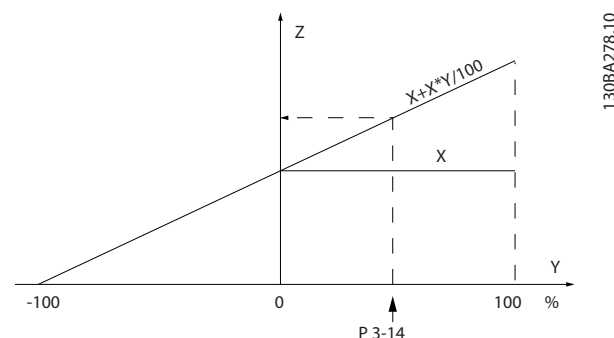
Рисунок 3.25 Фактическое задание
