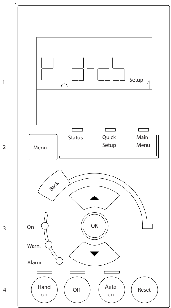
Рисунок 2.21 Кнопки LCP
