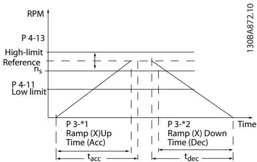
Рисунок 3.27 Линейное время изменения скорости
