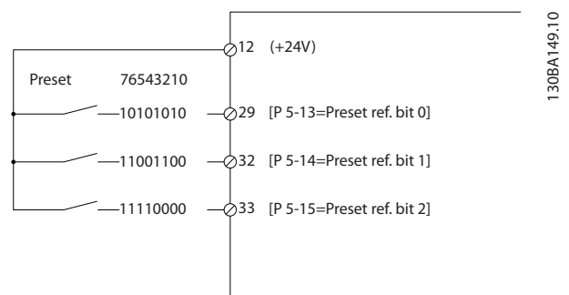
Рисунок 3.23 Предустановленное задание
