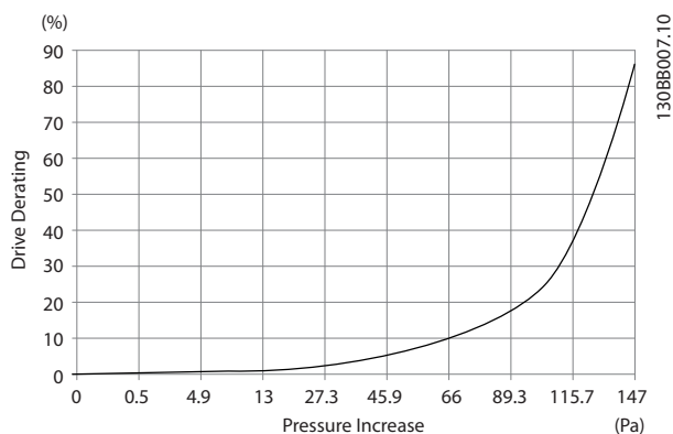
Рисунок 4.21 Корпус D Снижение значений относит. изменения давления
