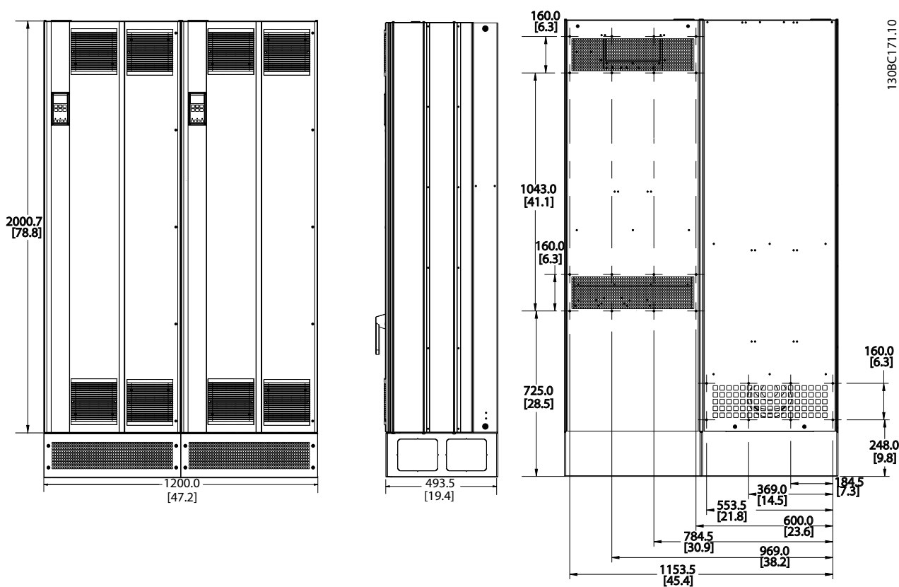
Рисунок 4.7 Типоразмер E9
