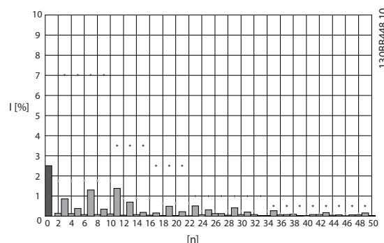
Рисунок 3.2 Типичный спектр гармонических частот и значение THD на сетевых клеммах привода n = порядок гармоники лимиты ◇.....IEEE519 ( I_{sc}/I_L > 20 ) для индивидуальных гармоник
