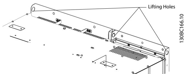
Рисунок 4.2 Рекомендуемый метод подъема, типоразмеры D13
