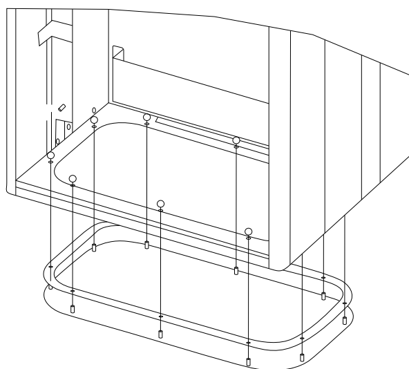
Рисунок 4.28 Монтаж нижней платы, типоразмер E9
