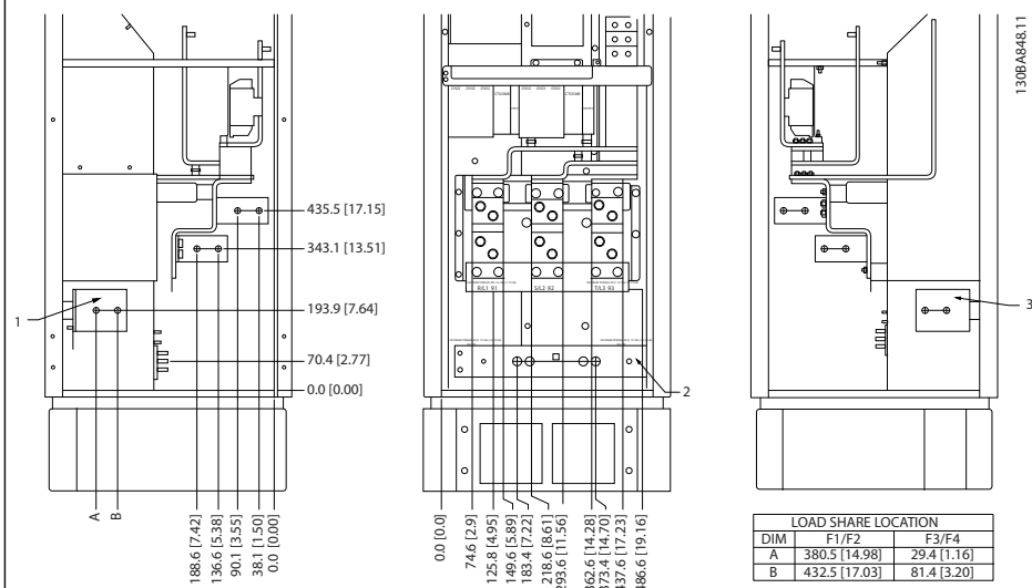
Рисунок 4.19 Расположение клемм — Выпрямитель
