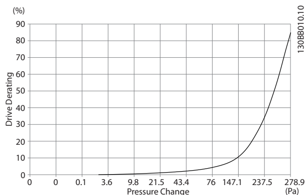
Рисунок 4.22 Корпус E Снижение значений относит. изменения давления (Малый вентилятор), P315
