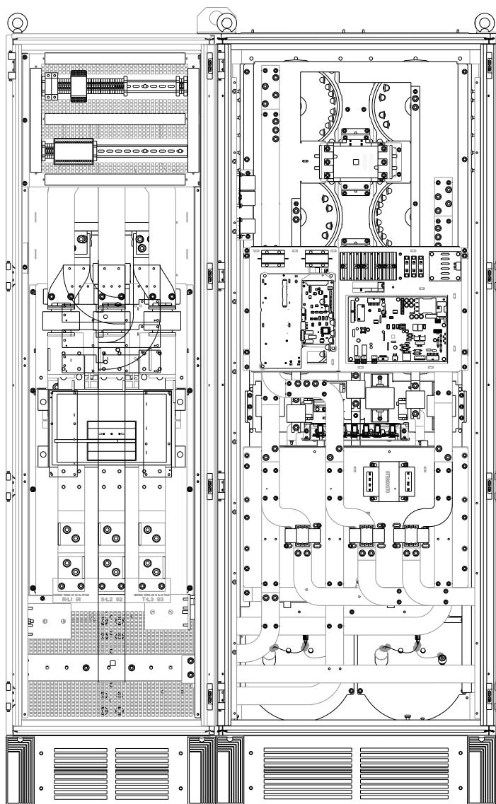
Рисунок 4.34 Активный фильтр, типоразмер F18
