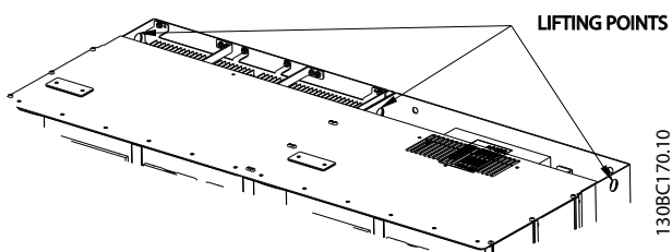
Рисунок 4.3 Рекомендуемый метод подъема, типоразмеры E9
