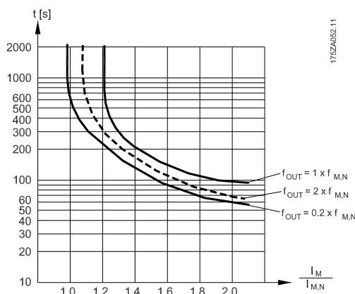
Рисунок 6.3 Профиль ЭТР
