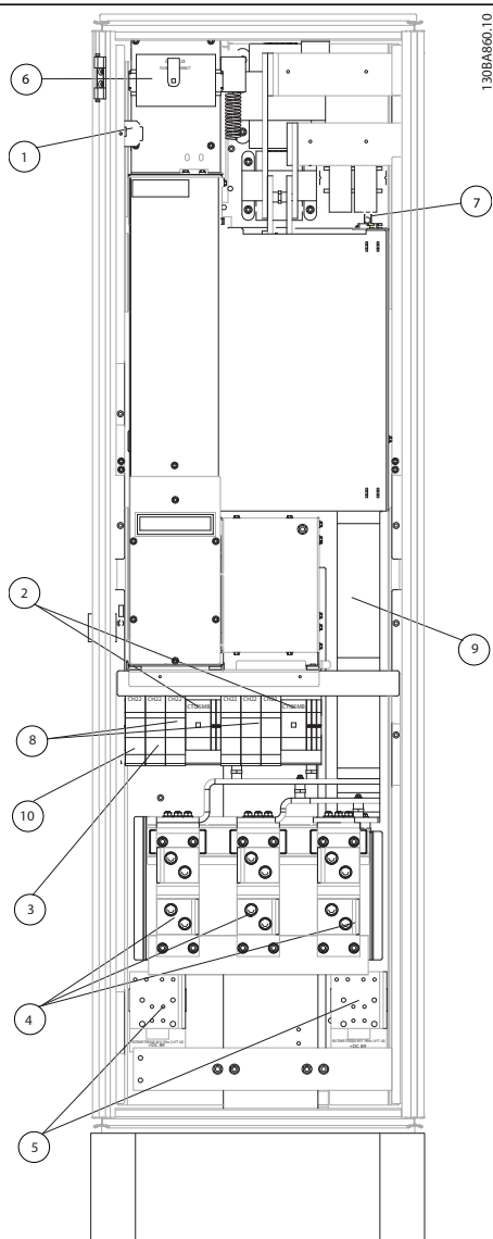
Рисунок 4.35 Шкаф выпрямителя, типоразмер F18
