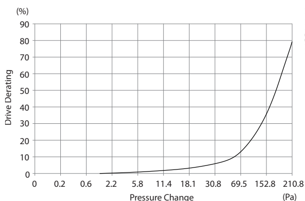
Рисунок 4.23 Корпус E Снижение значений относит. изменение давления (Большой вентилятор), P355-P450
