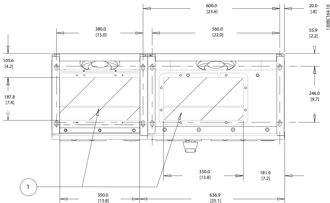
Рисунок 4.26 Типоразмер D13
