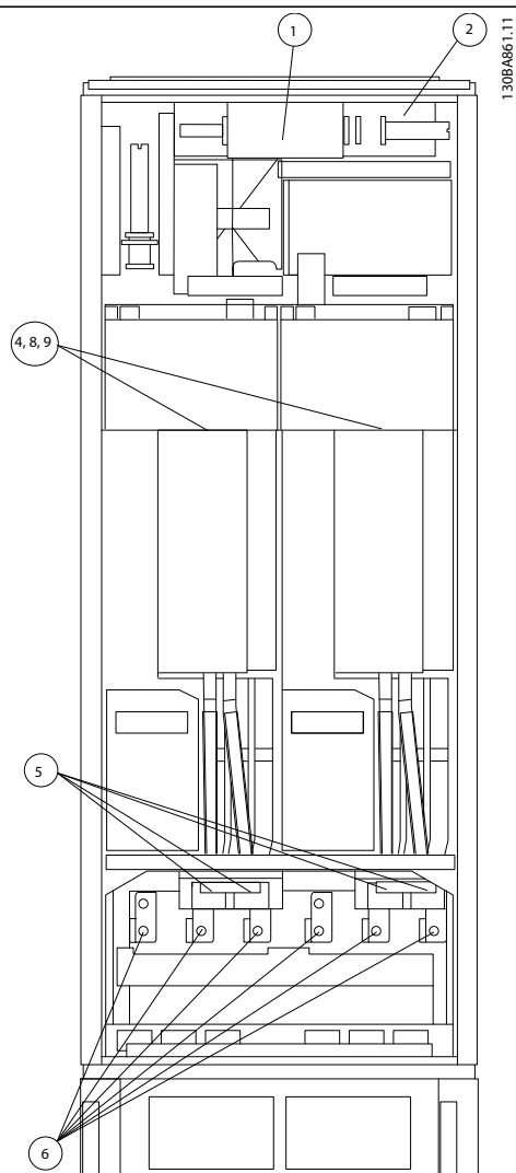
Рисунок 4.36 Шкаф инвертора, типоразмер F18
