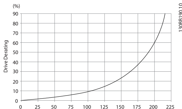
Рисунок 4.24 Корпус F Снижение значений относит. изменения давления
