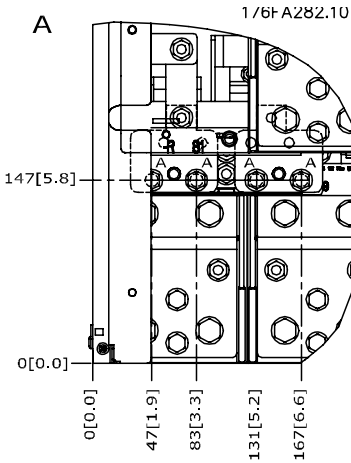
Рисунок 3.19: Расположение разъемов питания на корпусе IP00
