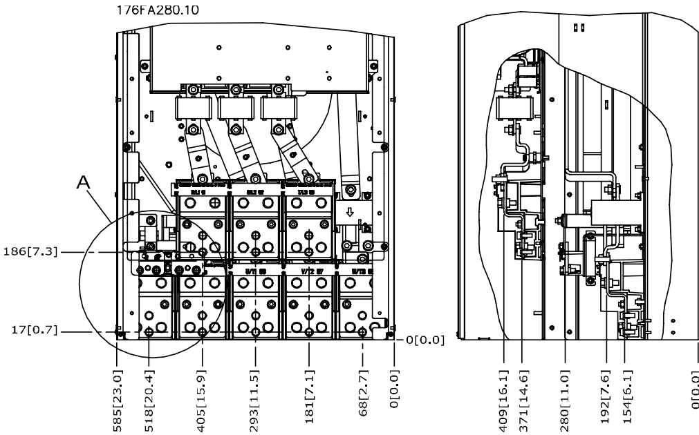
Рисунок 3.18: Расположение разъемов питания на корпусе IP00
