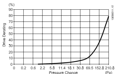
Рисунок 3.29: Корпус E Снижение значений относит. Изменение давления (Большой вентилятор), P315T5-P400T5 и P500T7-P560T7
