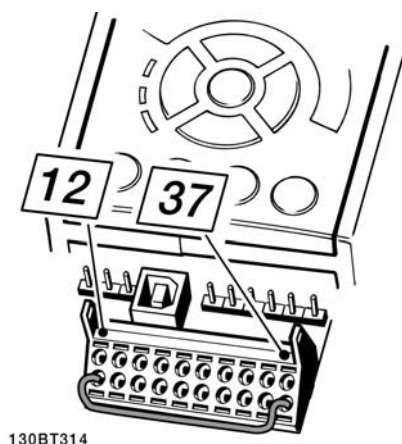
Рисунок 2.1: Соедините перемычкой клемму 37 и источник напряжения 24 В=.
