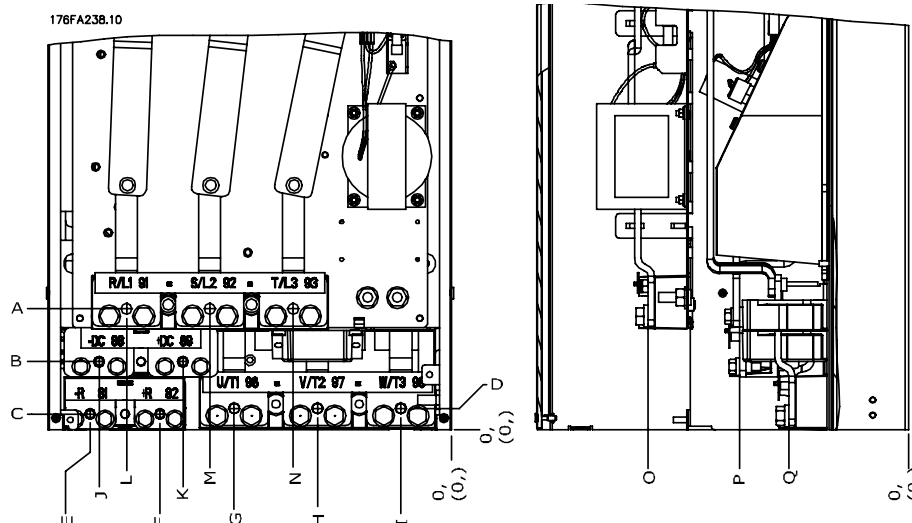
Рисунок 3.13: Расположение силовых разъемов, размер корпуса D3 и D4
