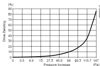
Рисунок 3.27: Корпус D Снижение значений относит. Изменение давления
