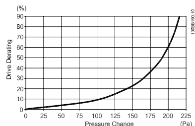
Рисунок 3.30: Корпус F1, F2, F3, F4 Снижение значений относит. Изменение давления
