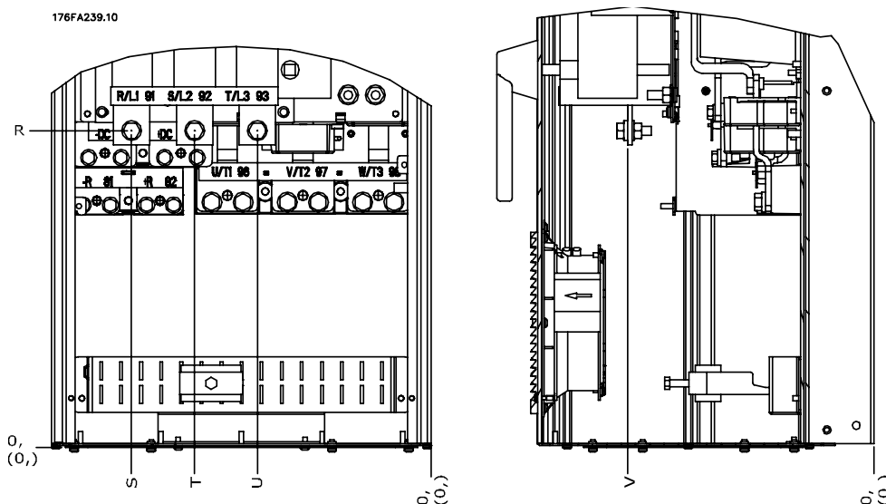
Рисунок 3.14: Расположение клемм электропитания с разъединителем, размер корпуса D1 и D2
