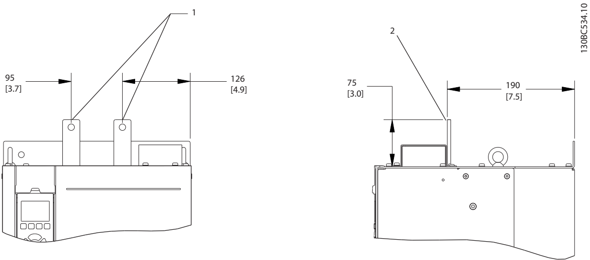
Рисунок 2.12 Клеммы цепи разделения нагрузки и рекуперации, D4h
