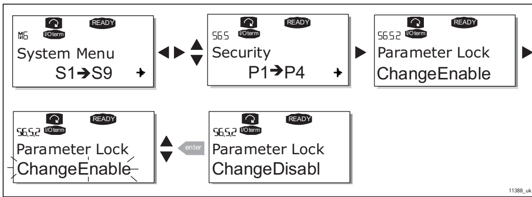
Figure 74. Parameter locking
