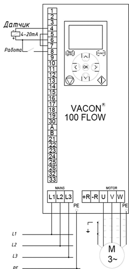
Рисунок 5. Режим поддержания постоянного давления, фиксированная уставка.
