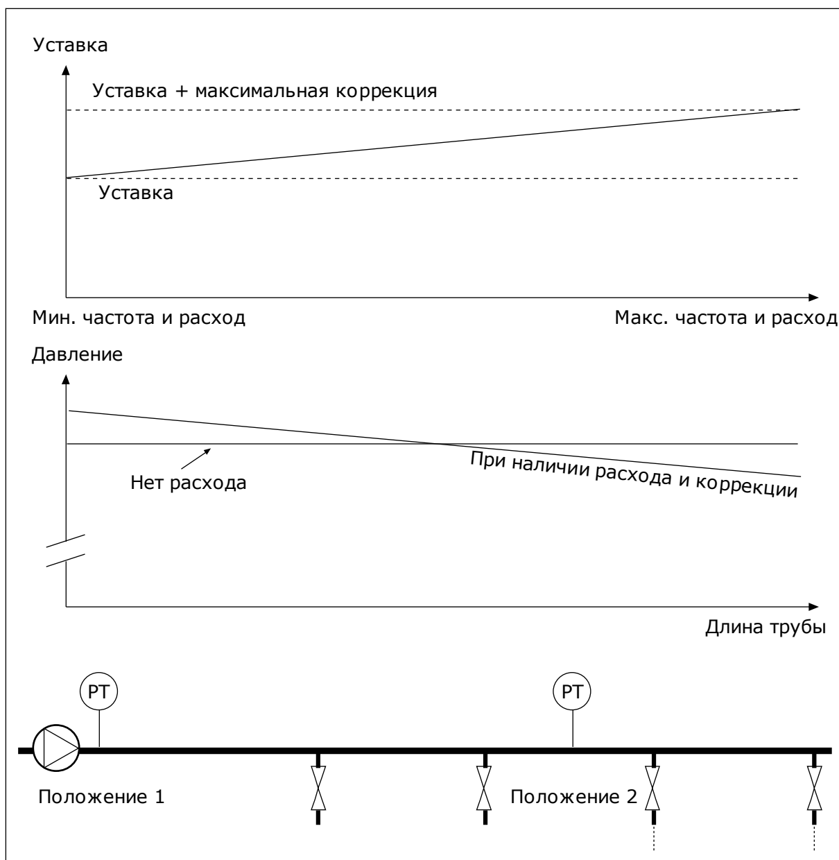
Рис. 84: Уставка 1, обеспечивающая компенсацию падения давления
