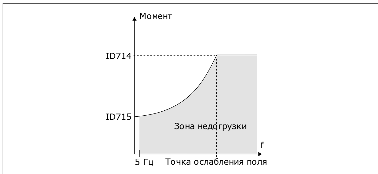
Рис. 68: Настройка минимальной нагрузки
