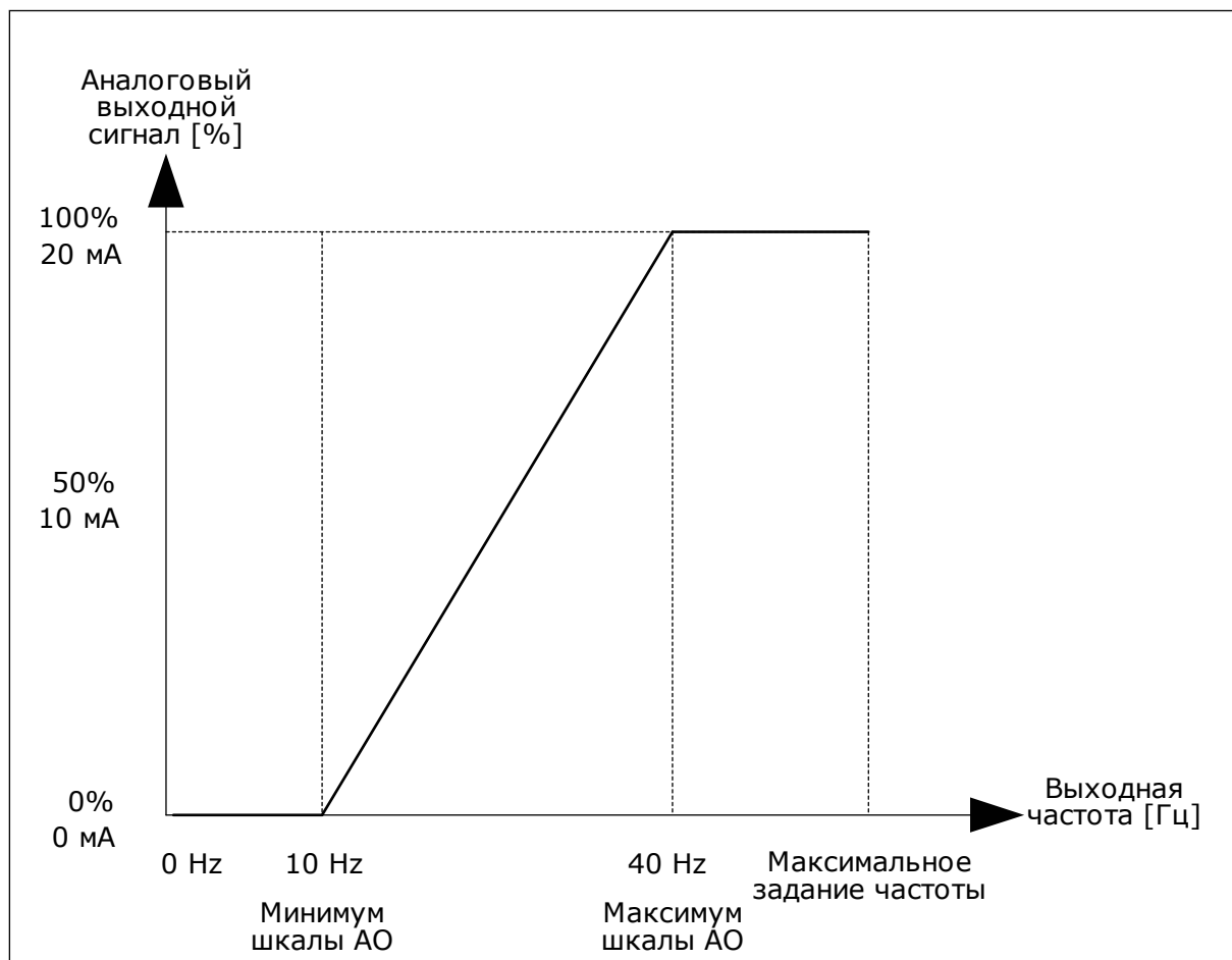
Рис. 61: Масштабирование сигнала AO1
