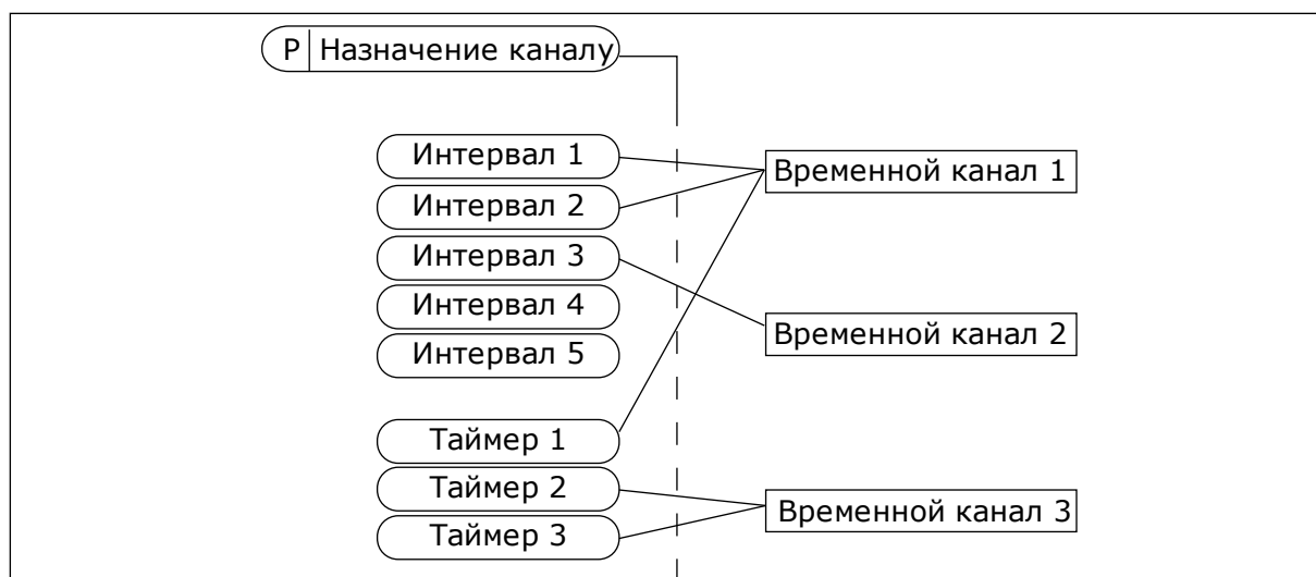
Рис. 72: Имеется возможность гибкого назначения интервалов и таймеров для временных каналов. Для каждого интервала и таймера предусмотрен собственный параметр для назначения временному каналу.
