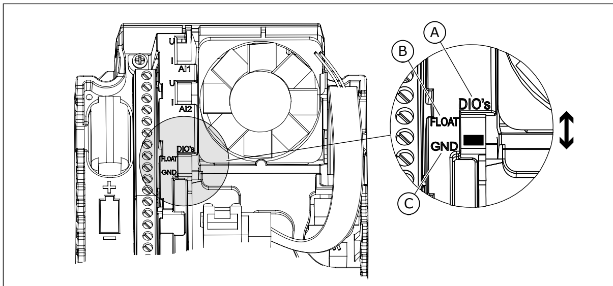
Рис. 7: DIP-переключатель
