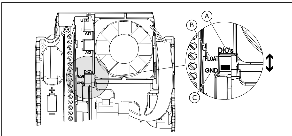
Рис. 96: DIP-переключатель изоляции
