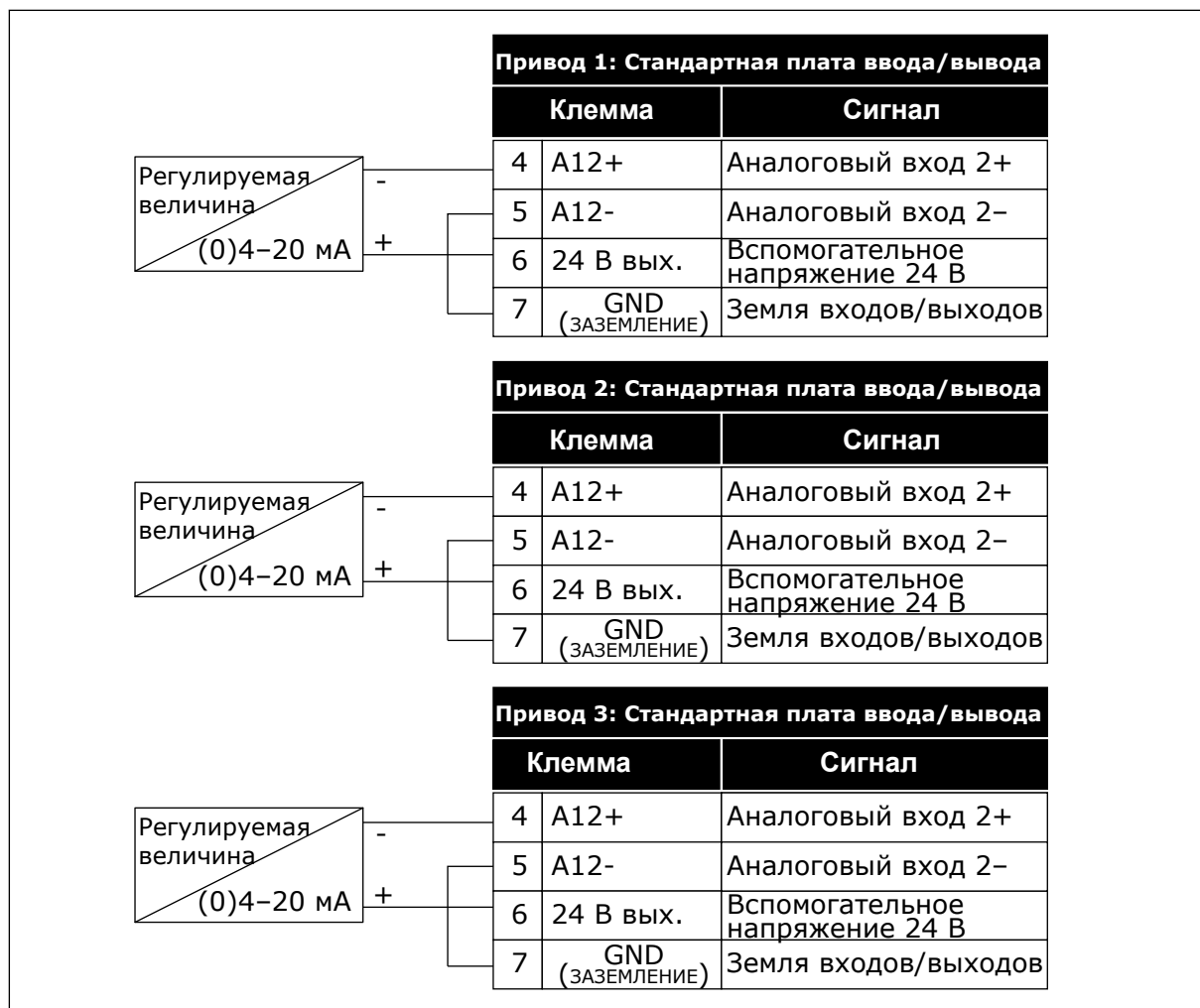
Рис. 93: Подключение отдельных датчиков обратной связи к каждому приводу
