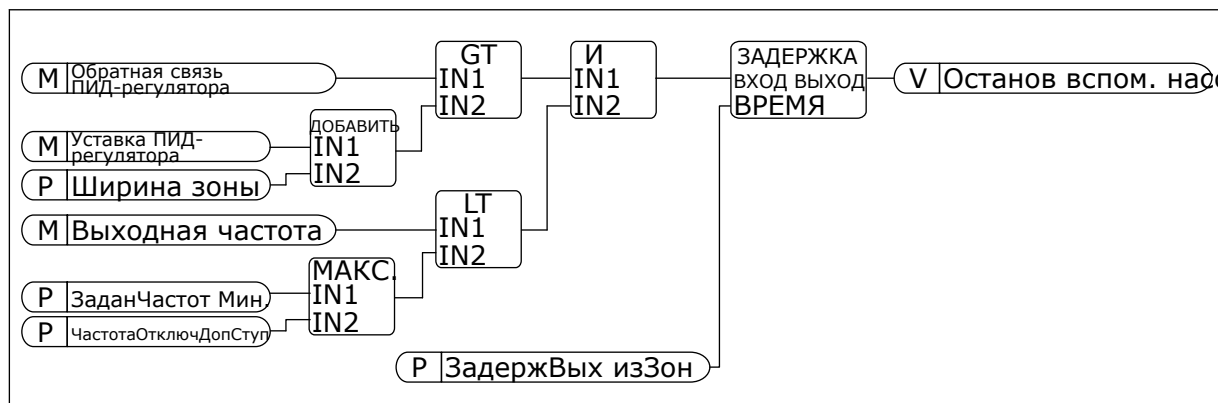
Рис. 101: Частота отключения доп. ступени
