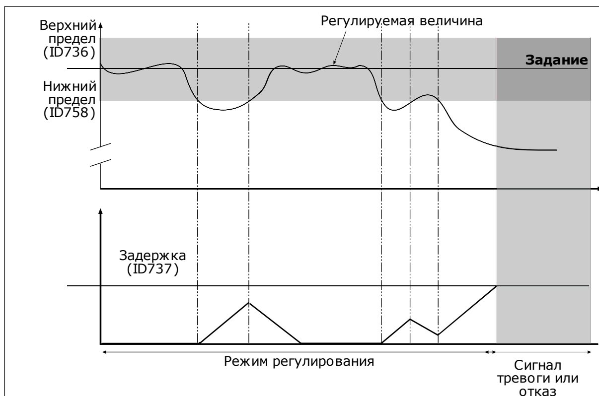
Рис. 82: Функция контроля обратной связи
