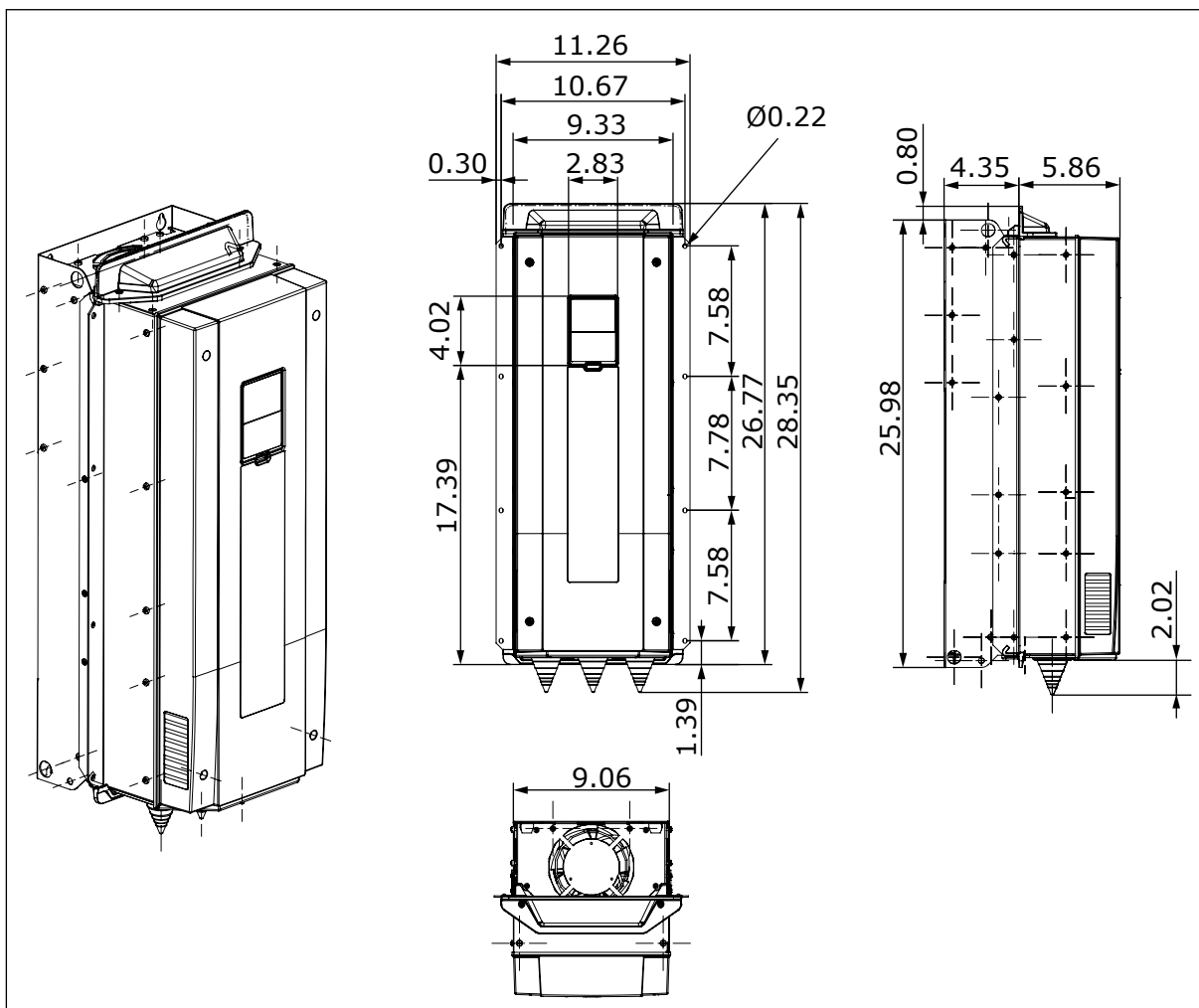
Рис. 30: Габариты преобразователя частоты, монтаж с использованием фланца, MR7 (дюйм)
