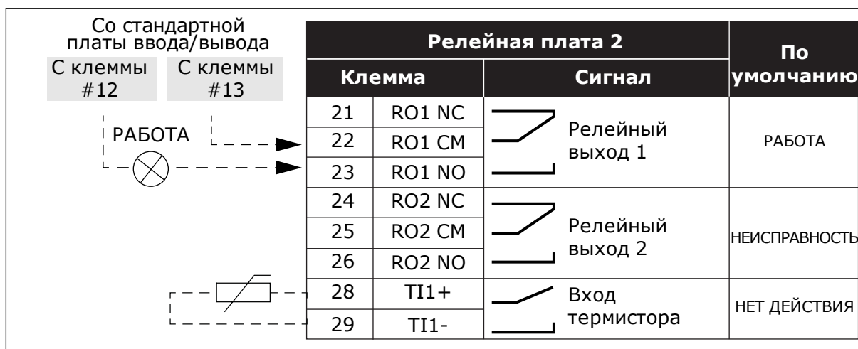
Рис. 27: Дополнительная релейная плата (+SBF4)
