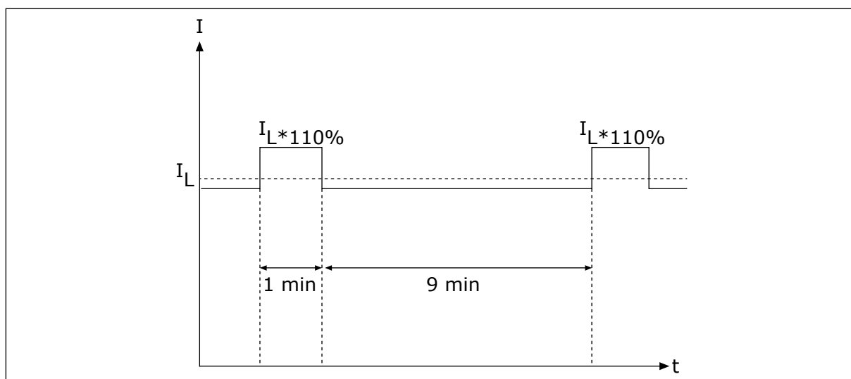
Рис. 37: Низкая перегрузка в Vacon® 100 HVAC
