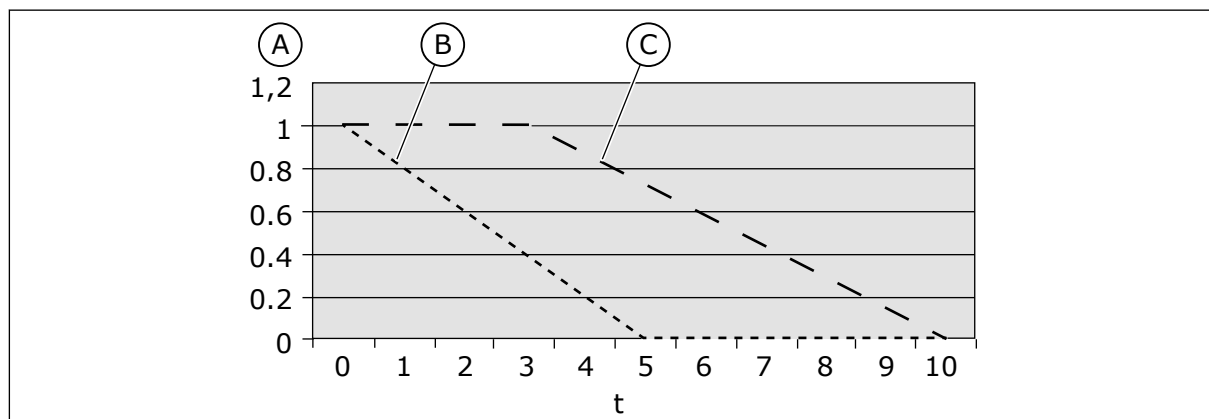
Рис. 34: Импульсы LD и HD
