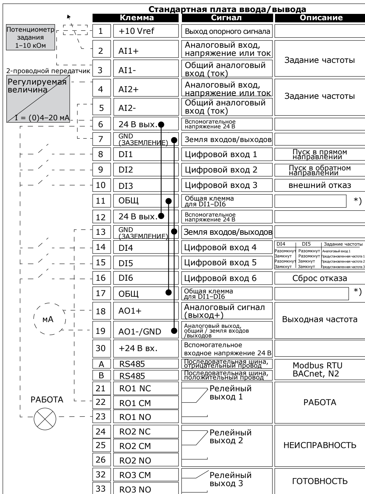
Рис. 25: Сигналы клемм управления привода на стандартной плате ввода/вывода и пример подключения. При заказе с дополнительным кодом +SBF4 релейный выход 3 замещается входом термистора.
