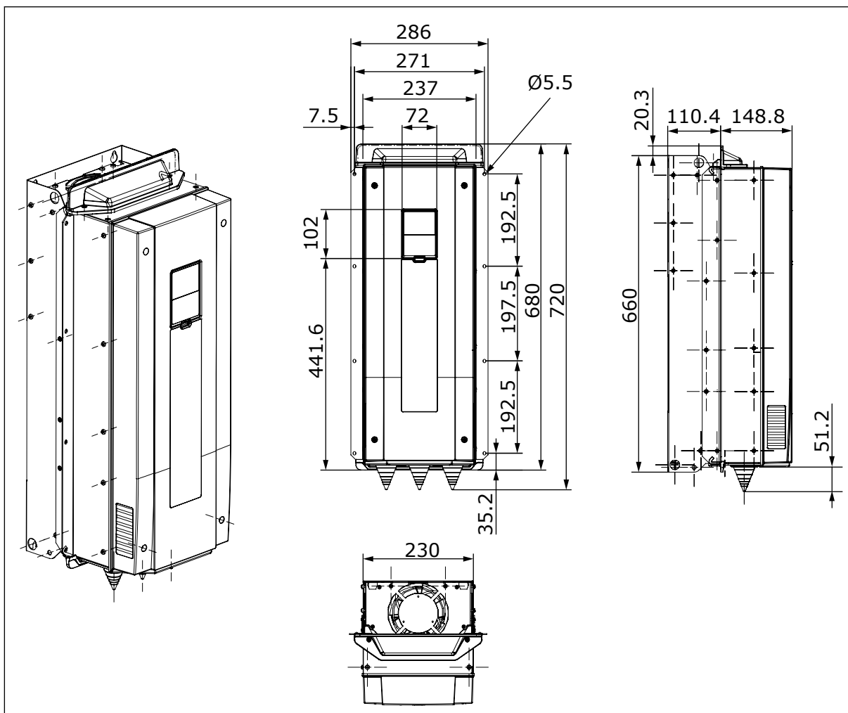
Рис. 16: Настенный монтаж привода переменного тока, фланцевое крепление, MR7
