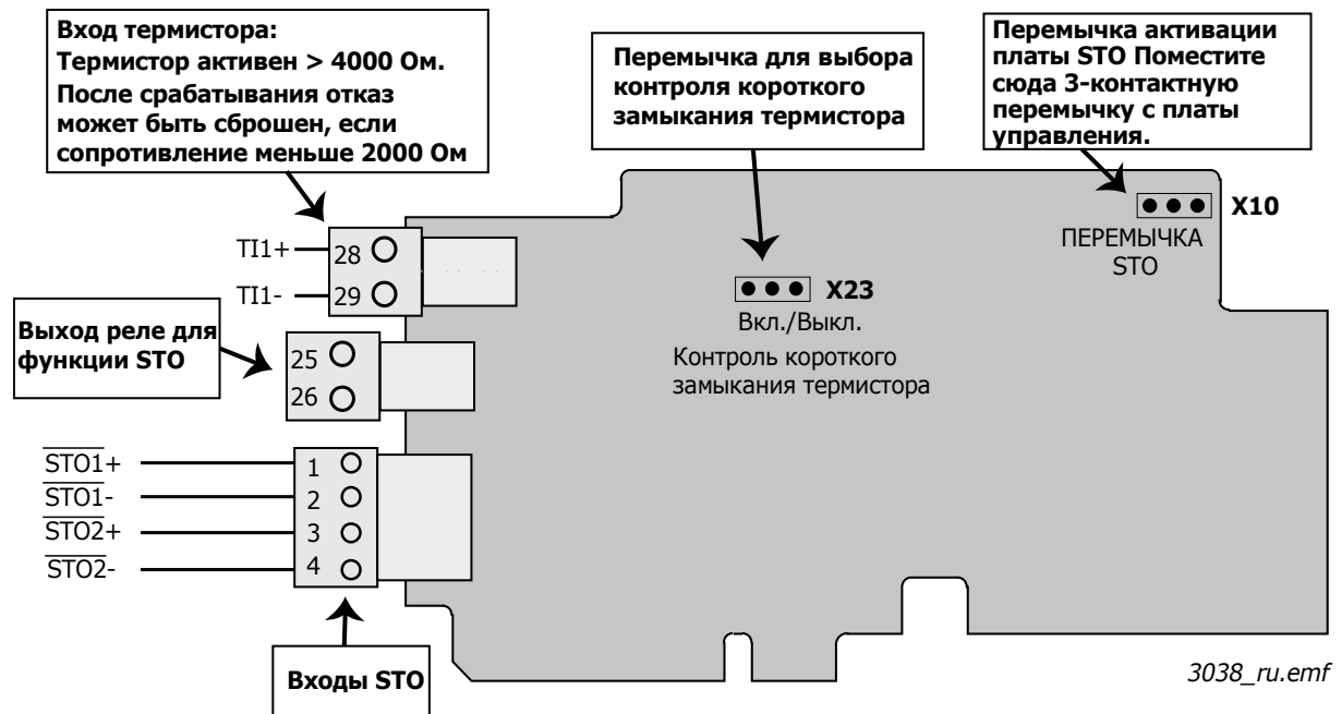
Рис. 1. Топология платы OPTBJ
