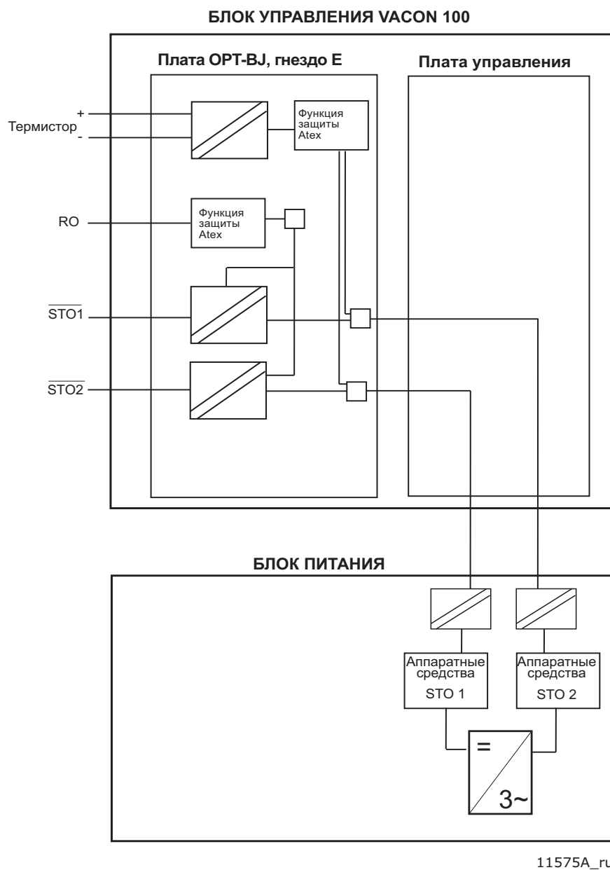
Рис. 9. Принцип действия термисторной функции в преобразователе частоты Vacon 100 с платой OPTBJ, MR4-10.
