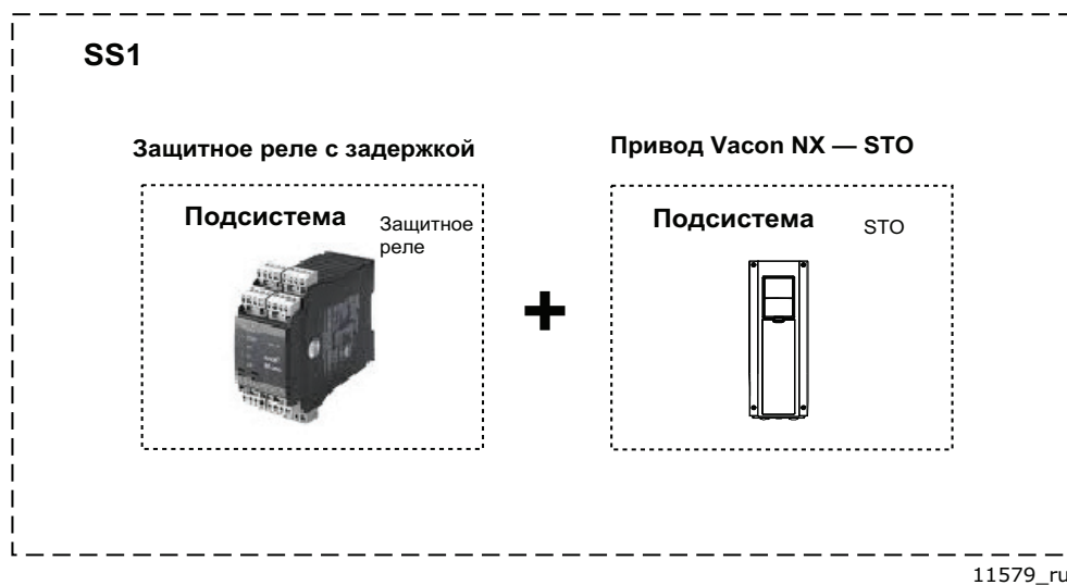
Рис. 7. Функция SS1
