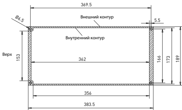
Рис. 5: Размеры выреза для фланцевого крепления приводов типоразмеров M14 (единица: мм)
