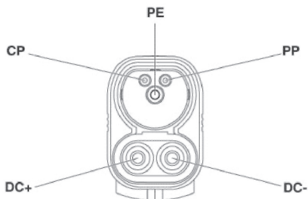
Рисунок 8.2 Определение контактов разъема CCS2
