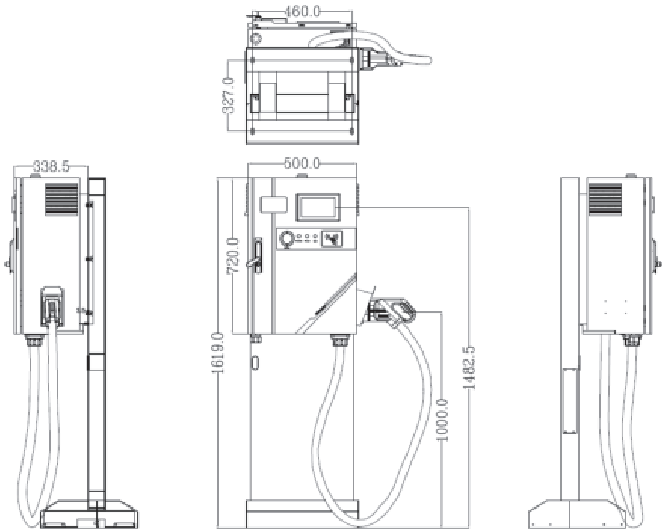
Рисунок 7.1 Размеры зарядного устройства (мм)
