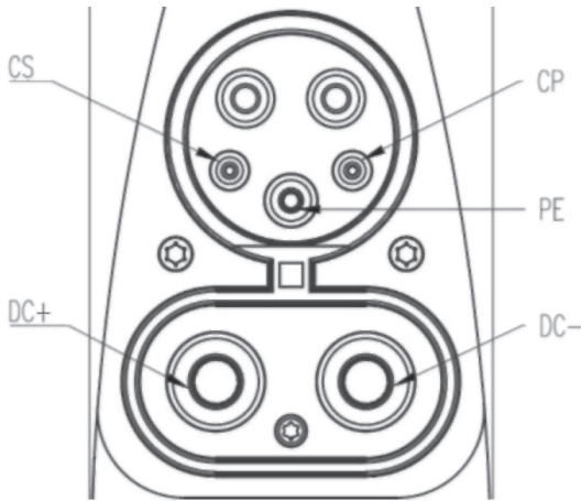
Рисунок 8.5 Определение контактов вилки CCS1
