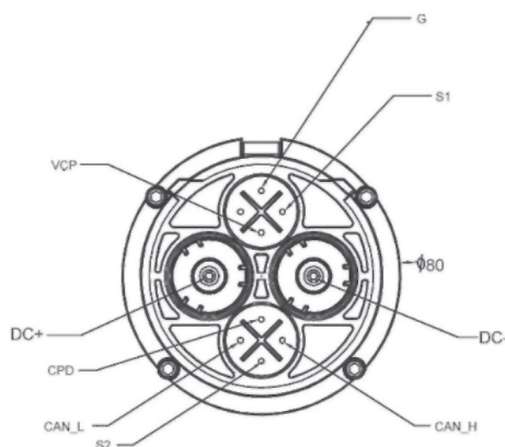
Рисунок 8.3.1 Определение контактов вилки CHAdeMO
