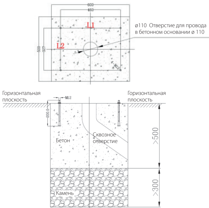
Рисунок 7.2.3 Строительный чертеж
