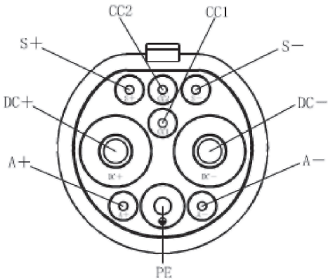
Рисунок 8.4 Определение контактов вилки постоянного тока GB/T
