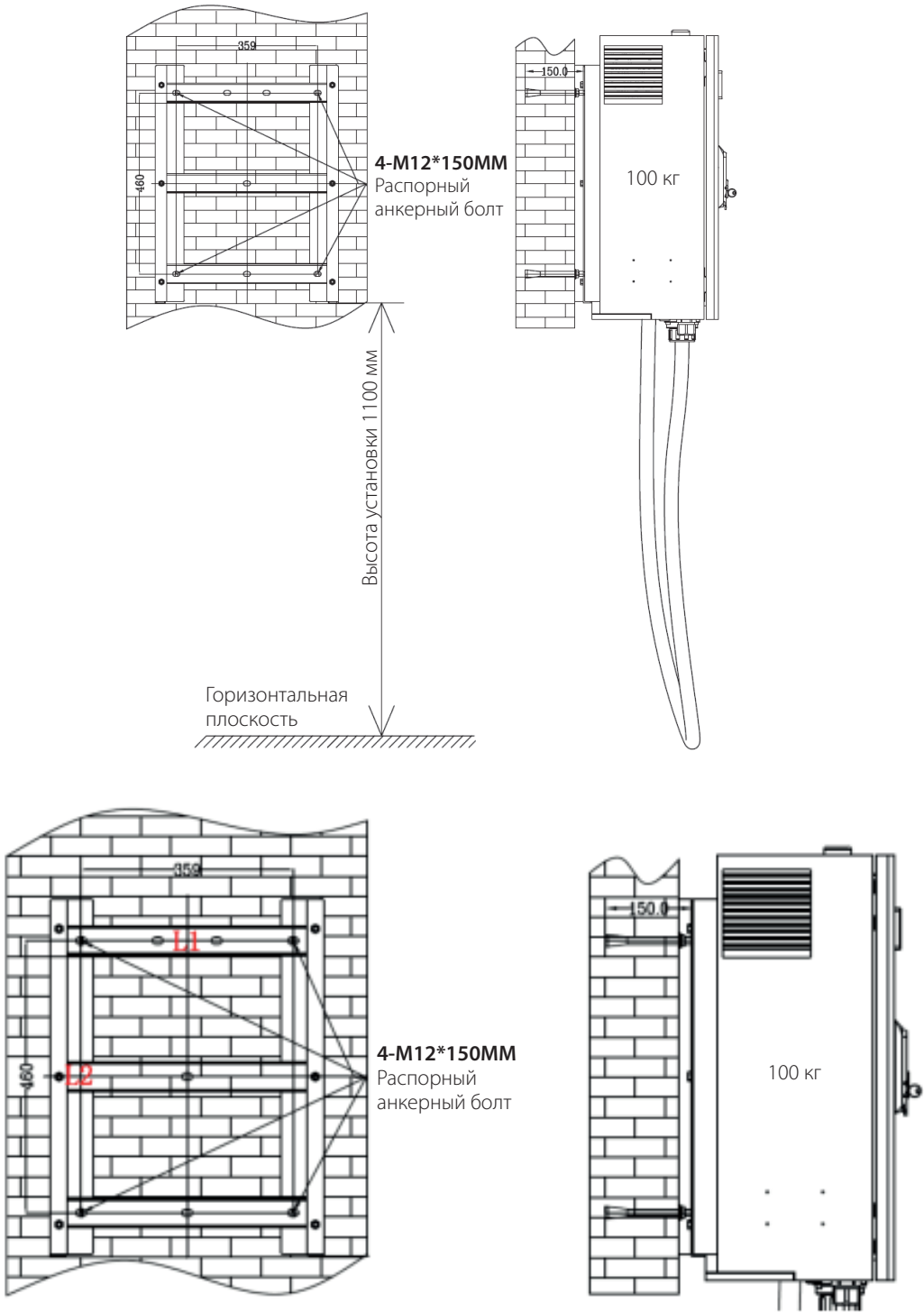
Рисунок 7.2.1 Монтажные чертежи дополнительной опоры
