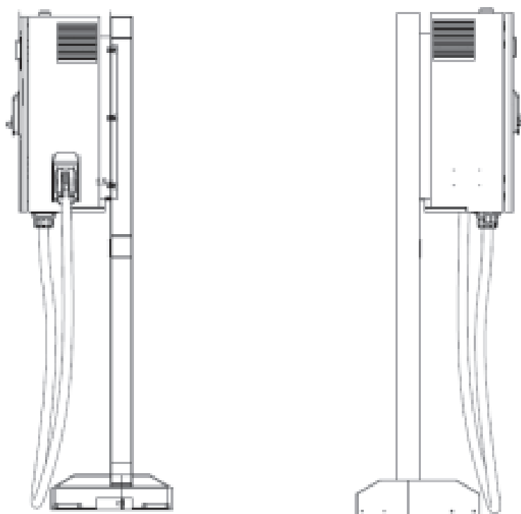
Рисунок 7.2.2 Монтажный чертеж зарядной станции
