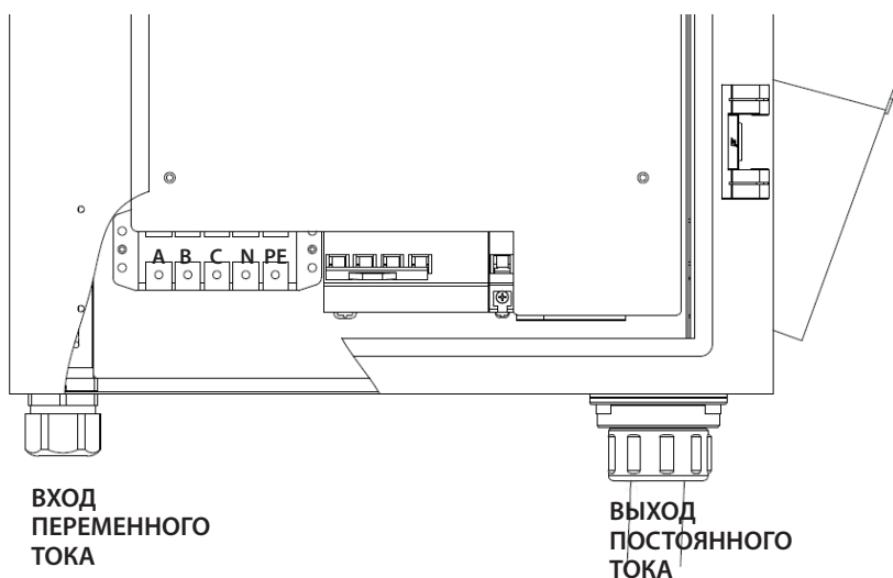
Рисунок 8.1 Схема подключения входного переменного тока зарядного устройства
