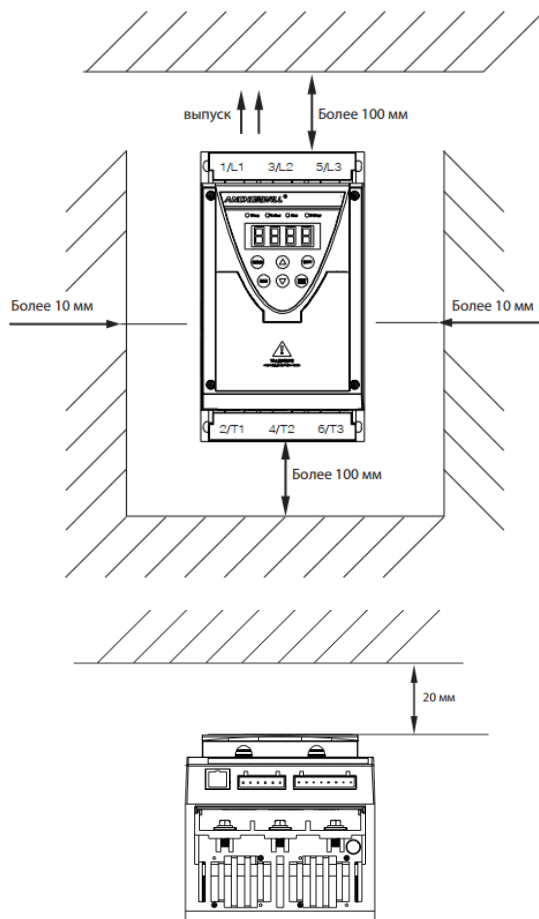
Рис. 3-1а Расстояние между местами установки (мм)
