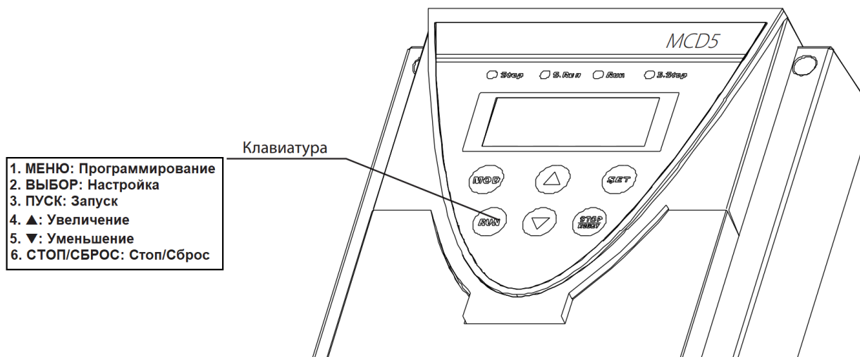
Рис. 4-1 ЖК дисплей и блок клавиатуры
