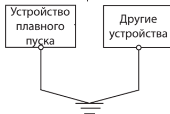
Рис. 3-8b Схема заземления
