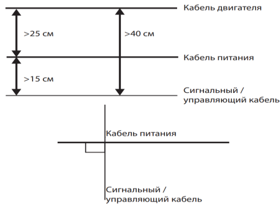
Рис. 3-7 Требования к разводке системы
