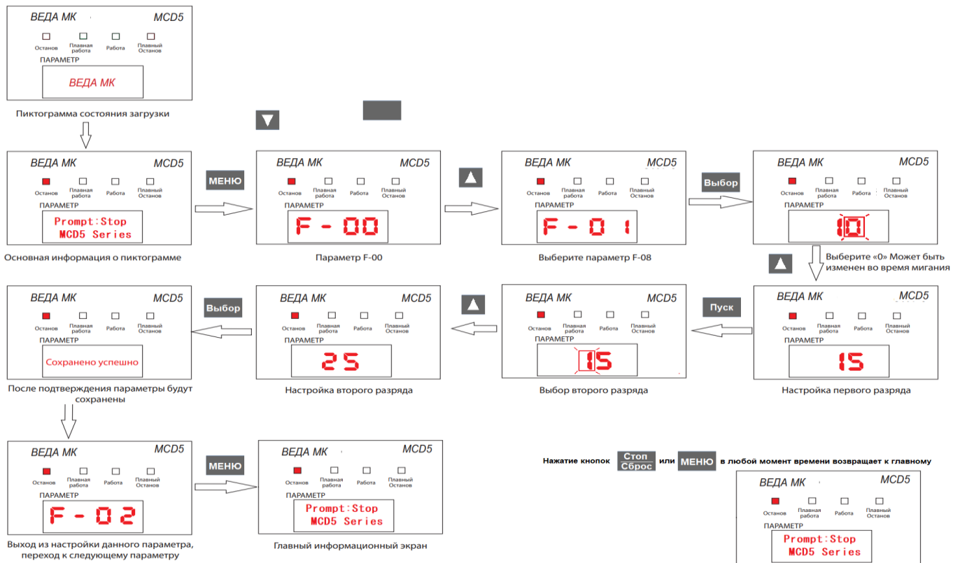
Рис. 4-4 Схема экрана
