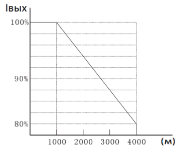
Рис. 1-2 Зависимость между номинальным током устройства плавного пуска и высотой над уровнем моря
