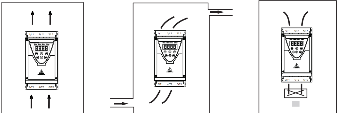
Рис. 3-1d Направление вентиляции
