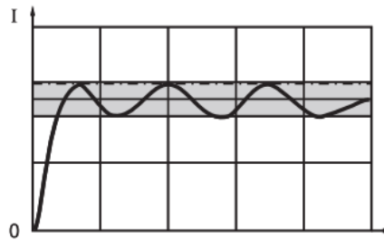
Рис. 5-4 Напряжение и время останова
