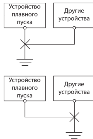
Рис. 3-8с Схема заземления 3
