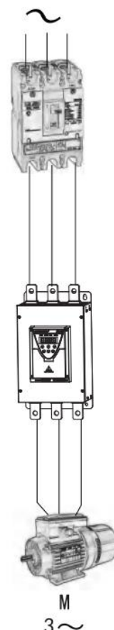
Рис. 3-2b Схема подключения силовой цепи УПП MCD5 с внутренним байпасным контактором
