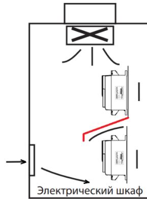
Рис. 3-1с Установка нескольких устройств друг над другом
