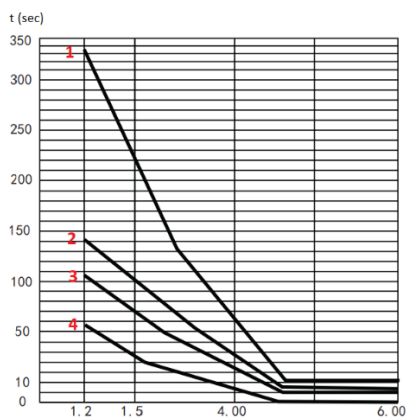
Рис. 5-7 Кривые класса перегрузки
