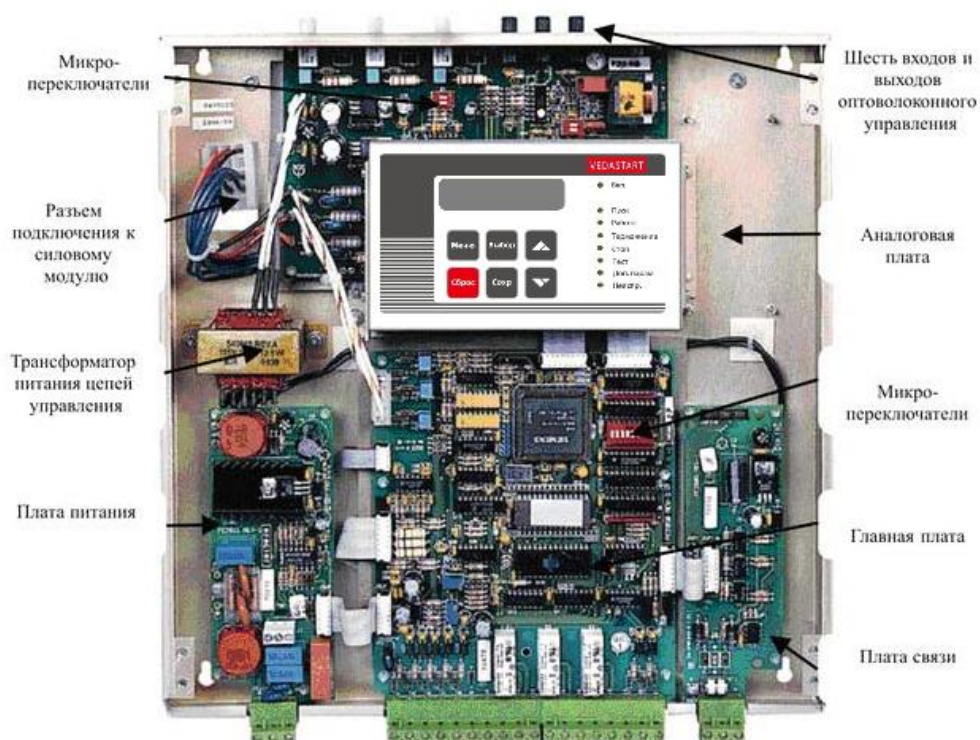
Рис. 7.4 – Модуль управления
