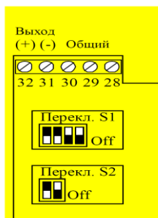
Рис. 7.6 – Модуль аналогового выхода
