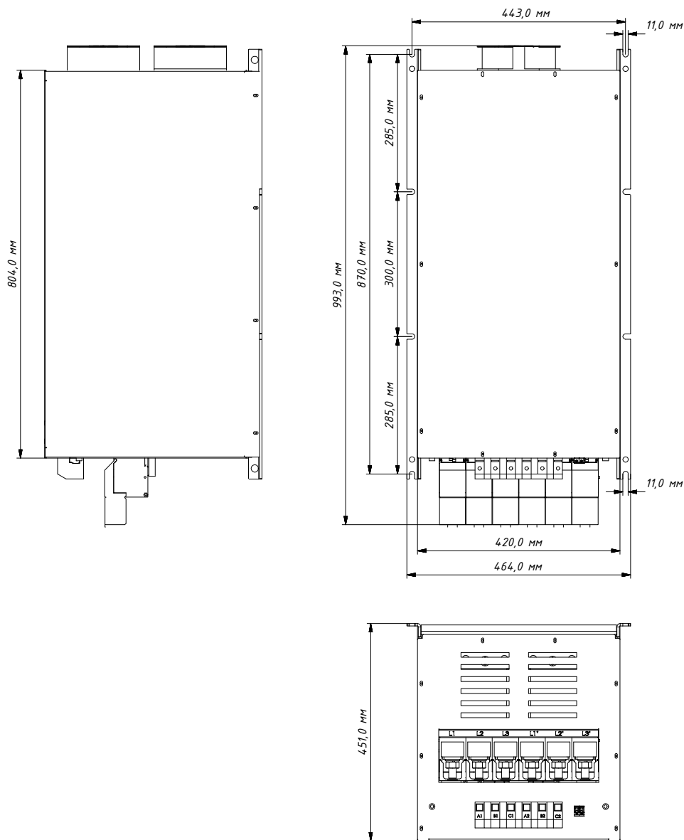
Рисунок 4.3.9. Типоразмер X7
