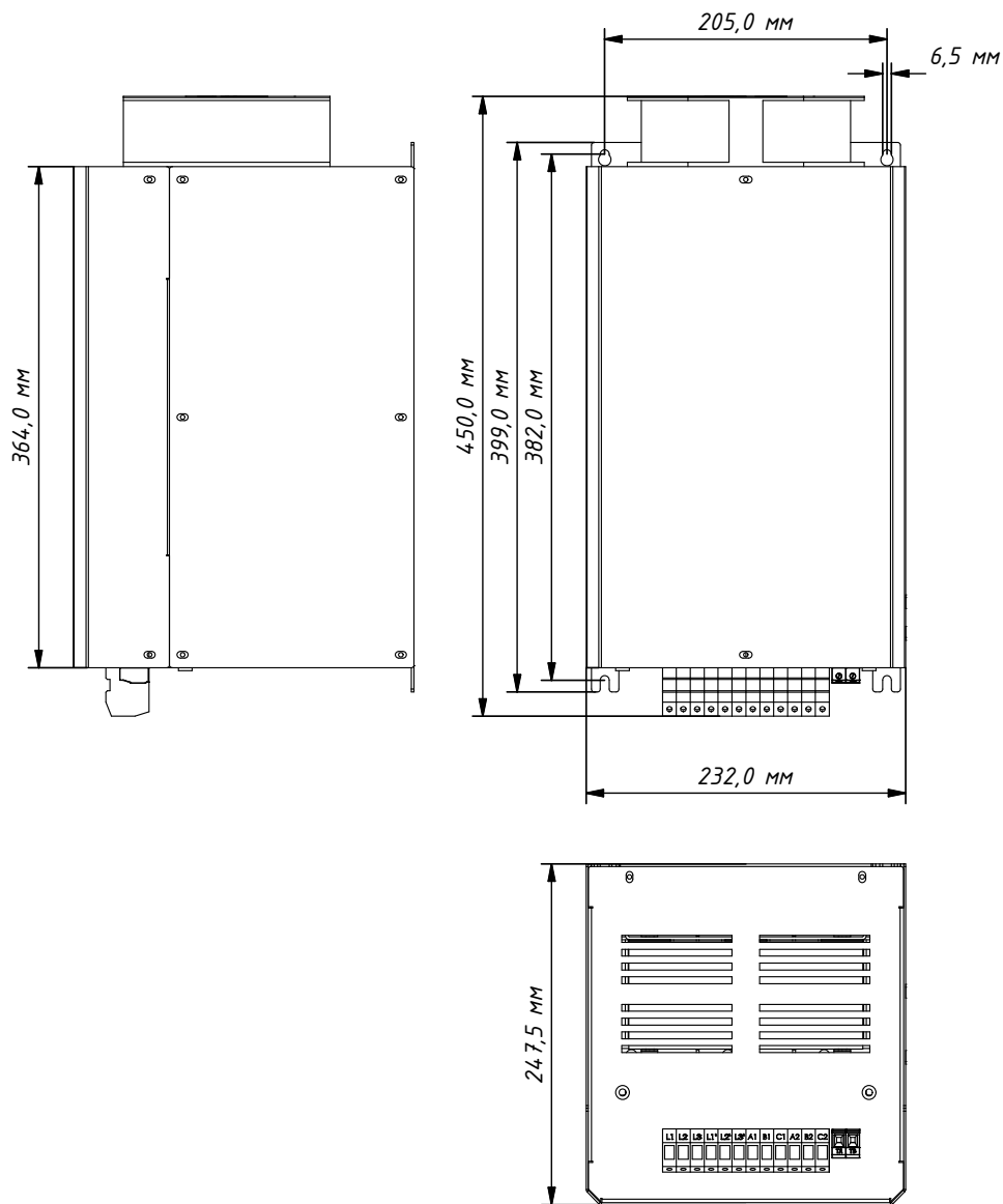
Рисунок 4.3.4. Типоразмер X2
