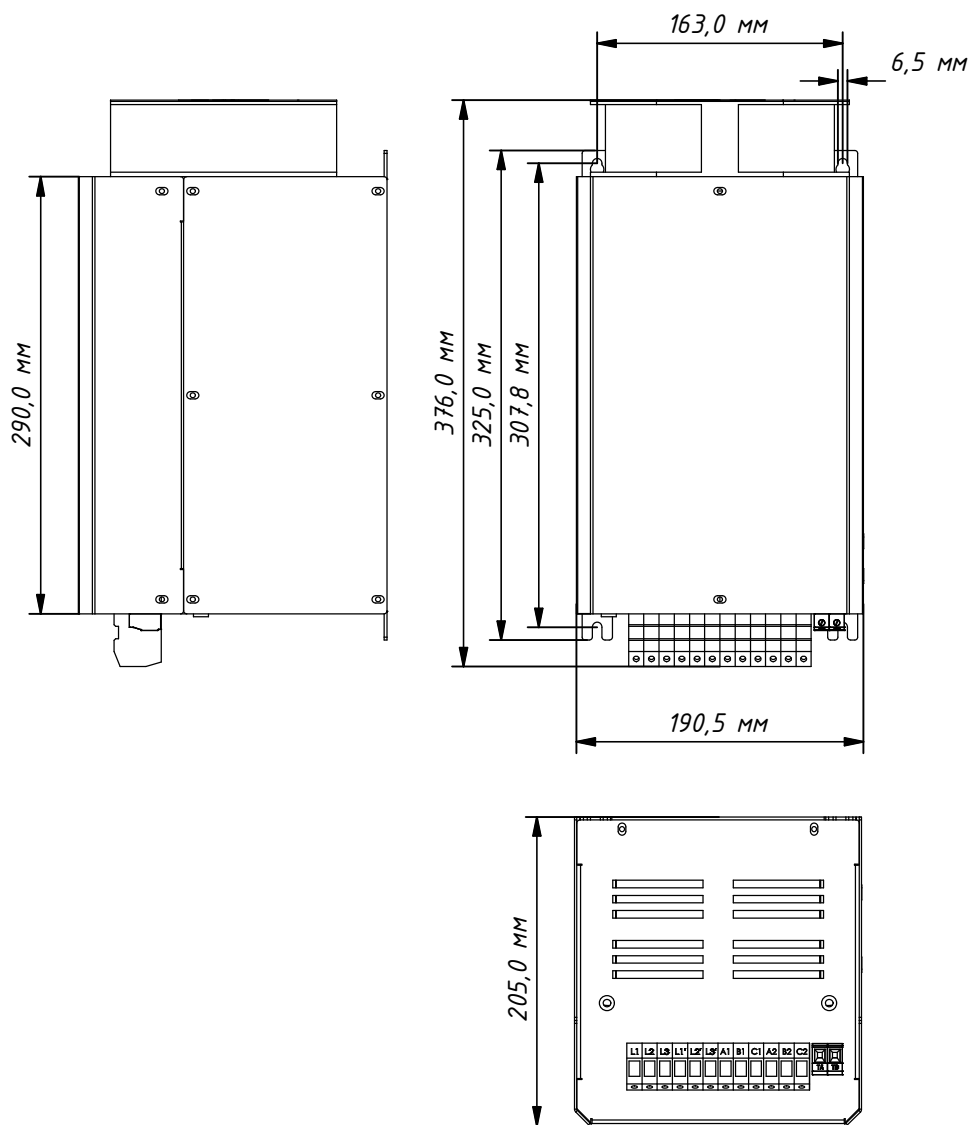
Рисунок 4.3.3. Типоразмер X1
