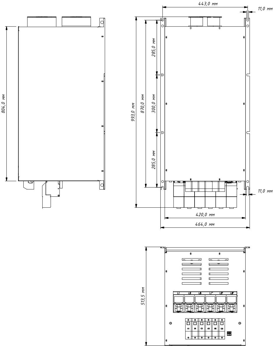
Рисунок 4.3.10. Типоразмер X8
