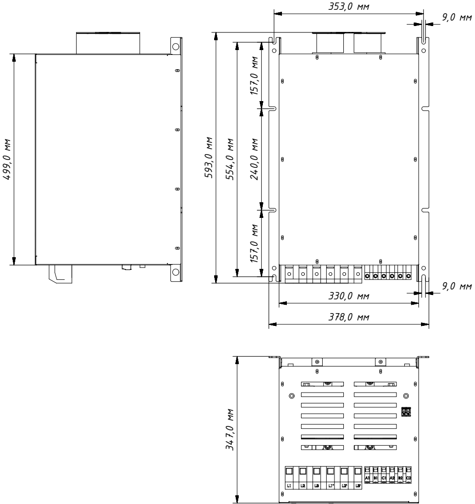
Рисунок 4.3.6. Типоразмер X4
