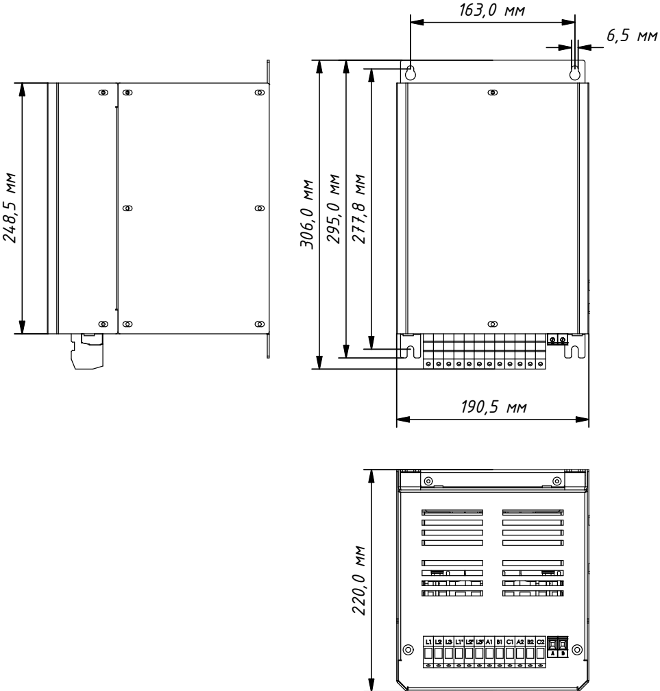
Рисунок 4.3.2. Типоразмер X1-2
