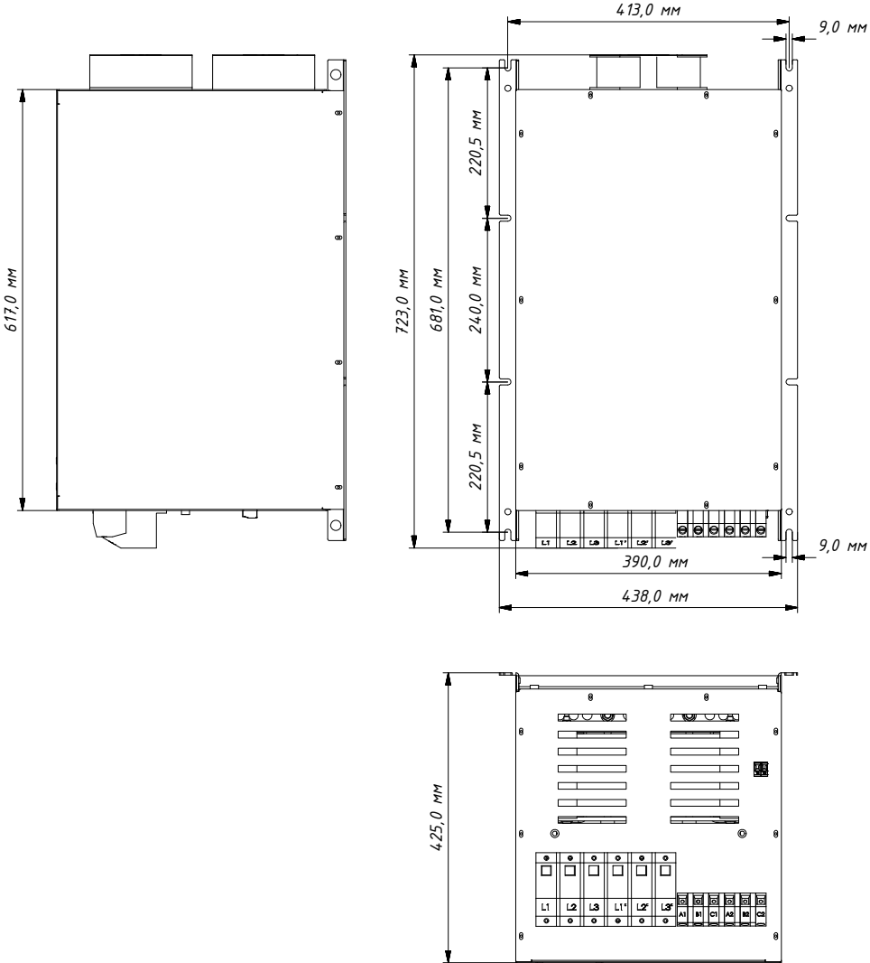
Рисунок 4.3.8. Типоразмер X6
