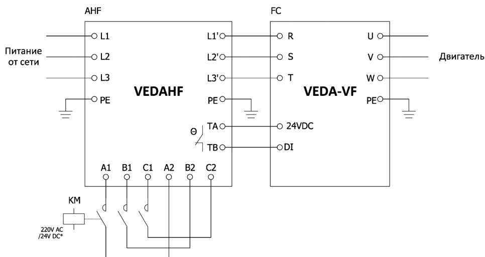
Рисунок 4.5.1. Схема подключения
