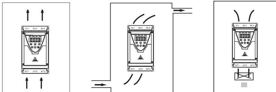
Рис. 3-1d. Направление вентиляции
