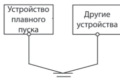
Рис. 3-8b. Схема заземления
