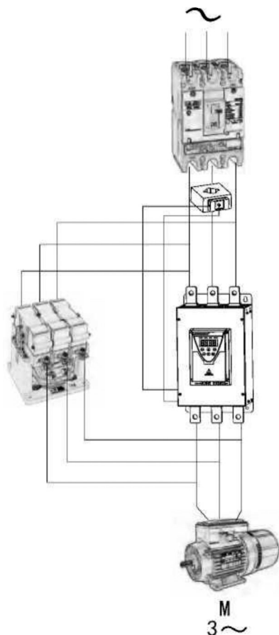
Рис. 3-2а. Схема подключения силовой цепи УПП без байпасного контактора.
